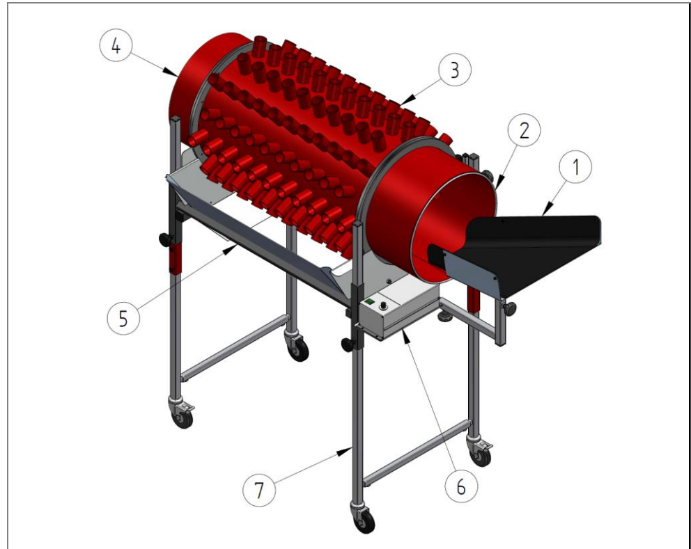
Abb. 3: Loch- und Igel-Separiertrommel
