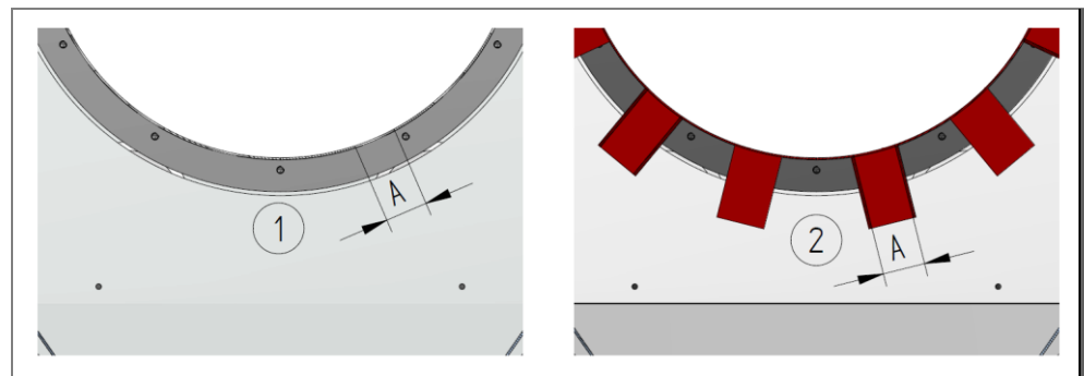
Abb. 4: Loch- und Igel-Separiertrommel
