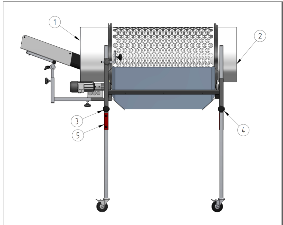
Abb. 9: Einstellen der Höhen und Neigung
