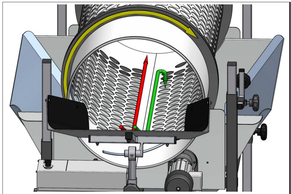
Abb. 2: Funktionsprinzip und Teiledurchlaufrichtung
