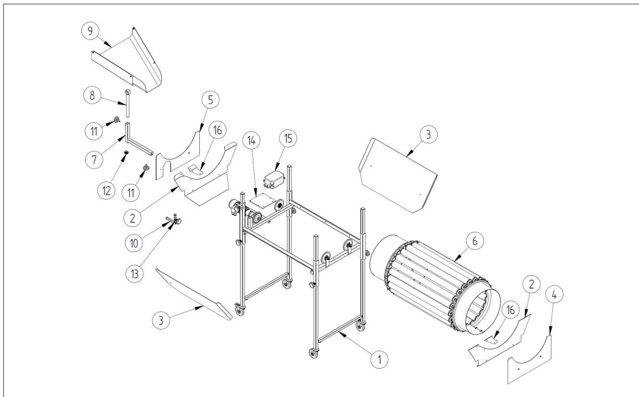
Abb. 19: Stückliste: Separiertrommel mit Einzelverstellung – ZZ.866.0001
