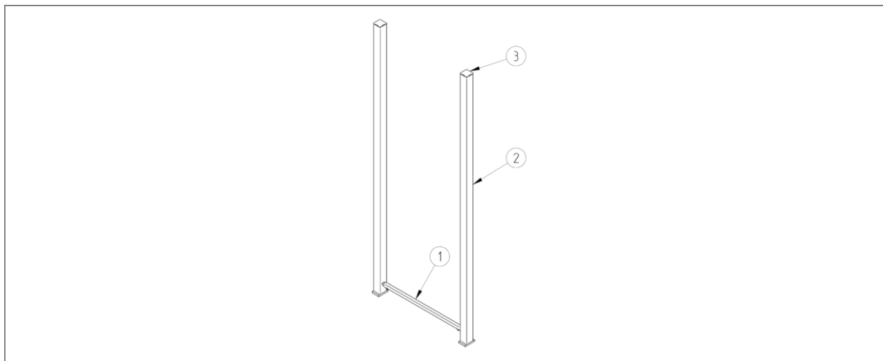
Abb. 25: Stückliste: Einzelständer – verstärkt – U.860.0017
