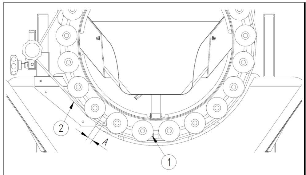
Abb. 4: Separierrollen und die Separierspalte dazwischen
