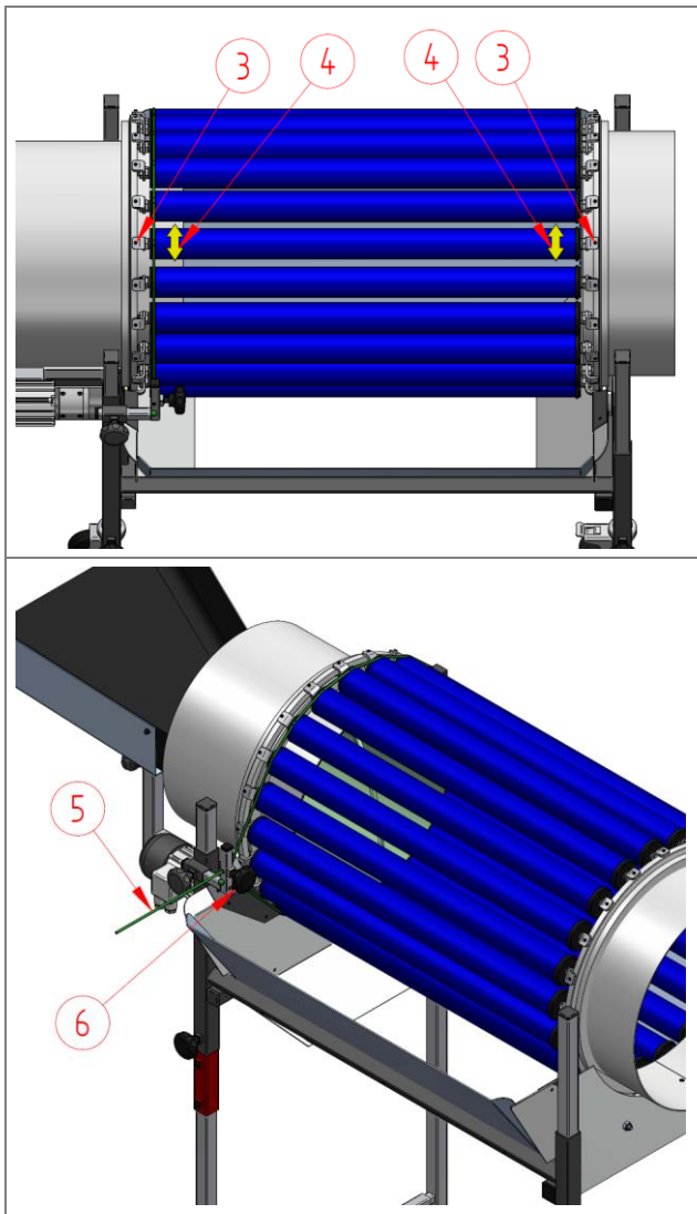
Abb. 10: Separierspalt einstellen (Einzelverstellung)
