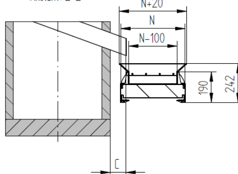
Ansicht: Z-Z
