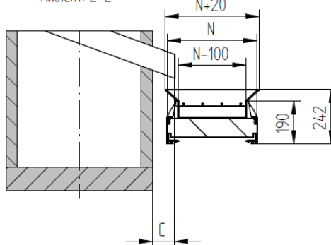
Ansicht: Z-Z
