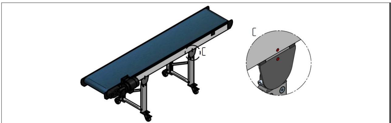
Abb. 34: Gesamtaufbau Montage Förderband mit Untergestell AM 010 (exemplarisch)
