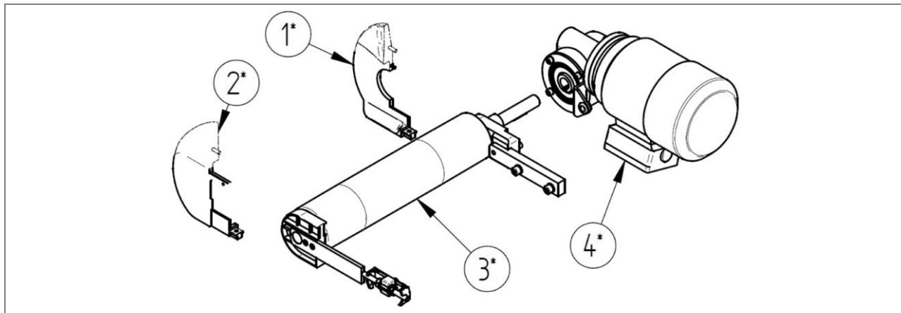
Abb. 102: Stückliste: Flanschtrieb - Antriebsposition 23 - ZZ.900.0150.00
