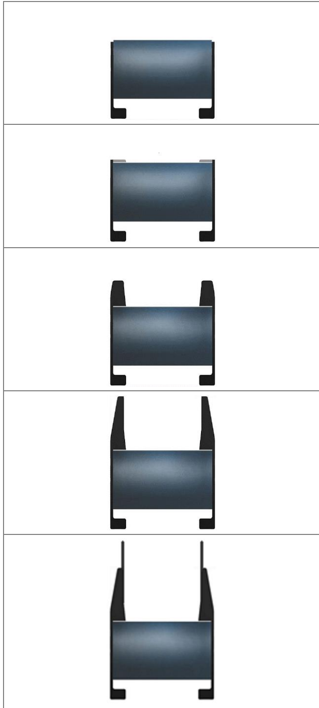
Abb. 12: Seitenführungen „GL“
