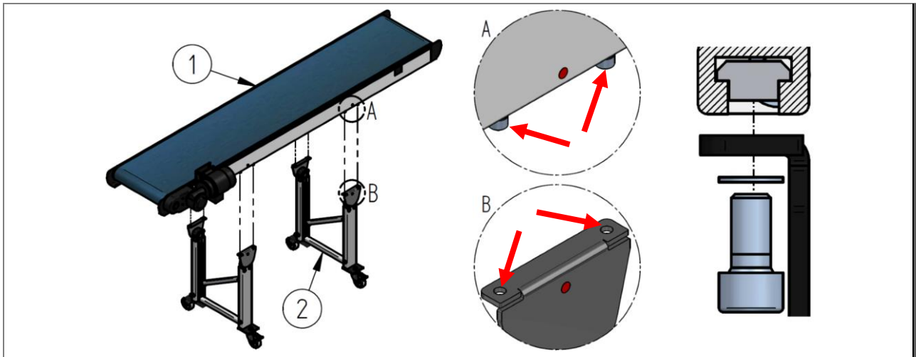
Abb. 33: Montage Förderband mit Untergestell AM 010 (exemplarisch)
