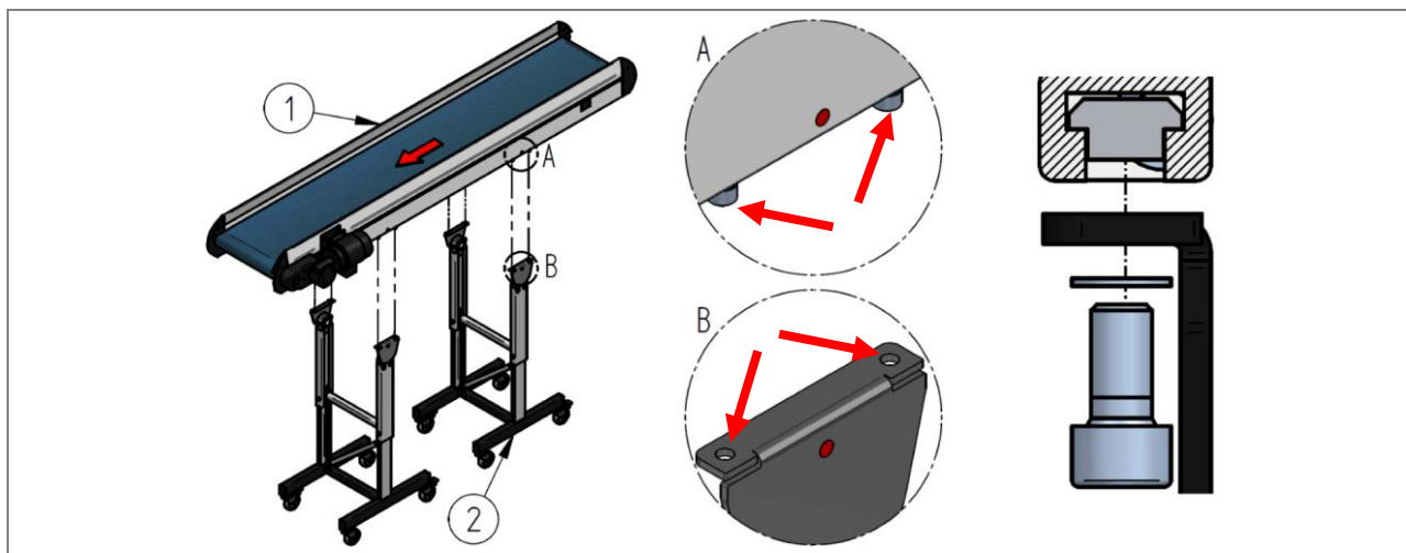
Abb. 45: Montage Förderband mit Untergestell HE 010 – HM 010 (exemplarisch)
