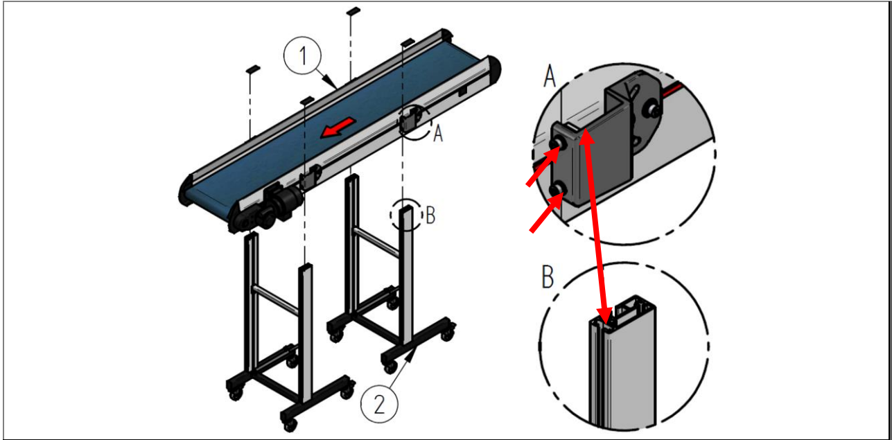
Abb. 49: Montage Förderband mit Untergestell HE 020 – HM 140 (exemplarisch)
