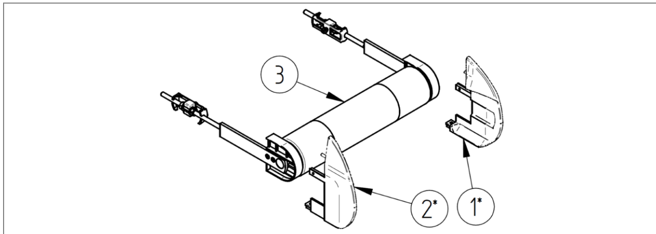
Abb. 82: Stückliste: Multi-Tech Umlenkeinheit Ø80– ZZ.800.0216.00
