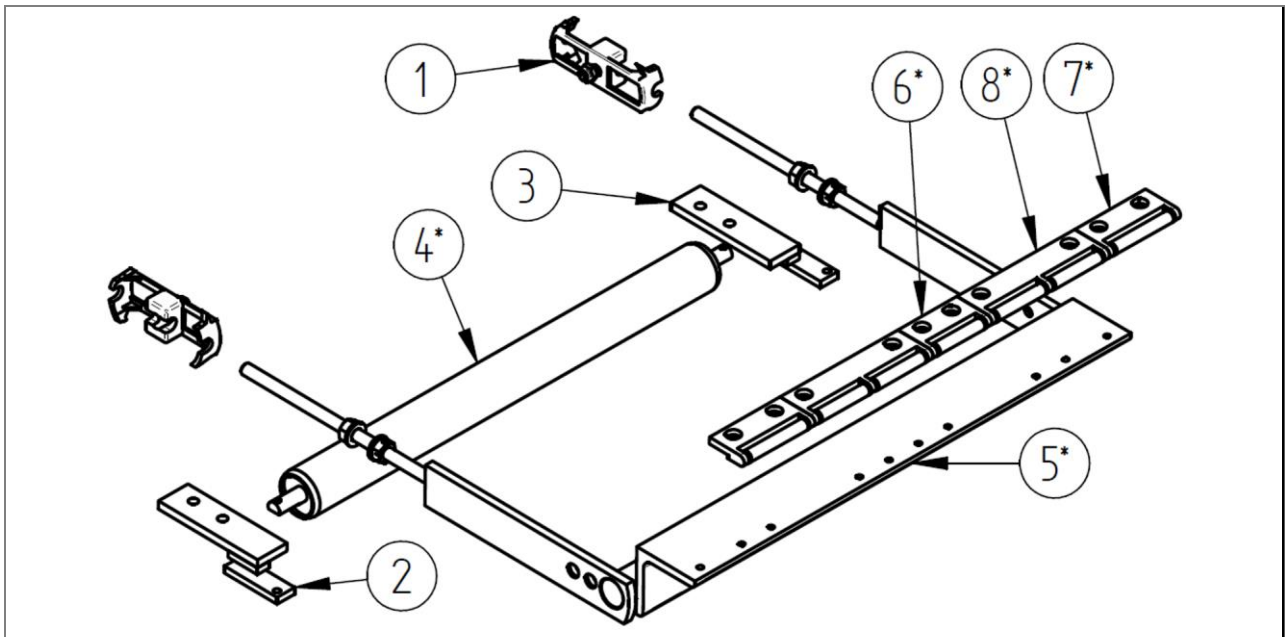
Abb. 87: Stückliste: Multi-Tech Rollende Messerkante Ø16/Ø08– ZZ.800.0171.00/ZZ.800.0172.00
