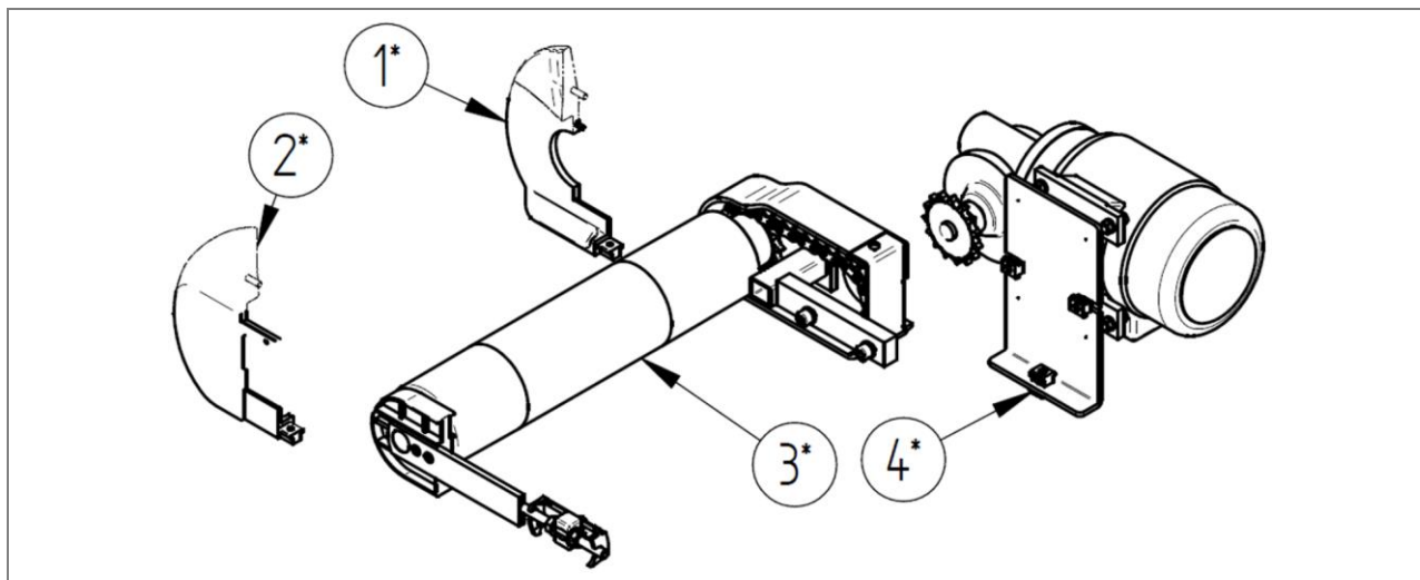
Abb. 91: Stückliste: Außenliegender Antrieb - Antriebsposition 23 - ZZ.900.0143.00
