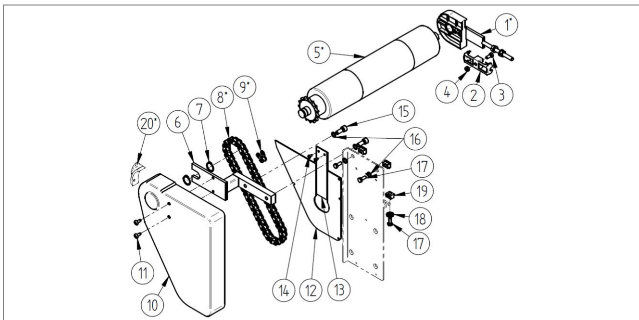
Abb. 95: Stückliste: Unterhalb liegender Antrieb - Antriebseinheit - Antriebsposition 14 - ZZ.900.0072.00
