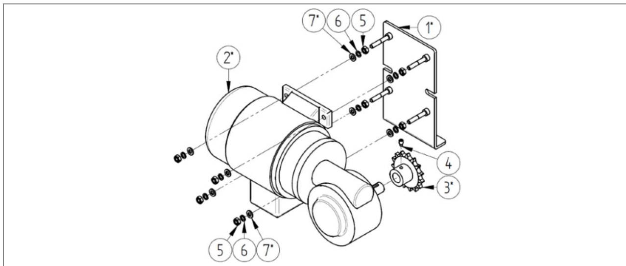
Abb. 93: Stückliste: Außenliegender Antrieb - Motoreinheit - Antriebsposition 23 - T.900.0002.02
