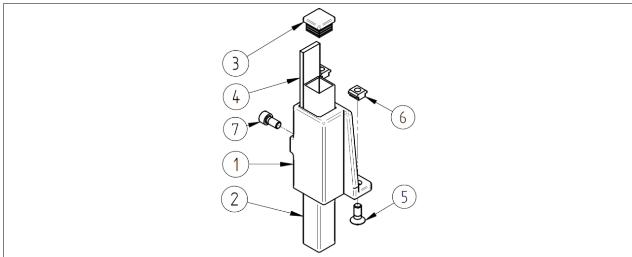
Abb. 114: Stückliste: Förderbandabstützung IK1 U.800.0182.00
