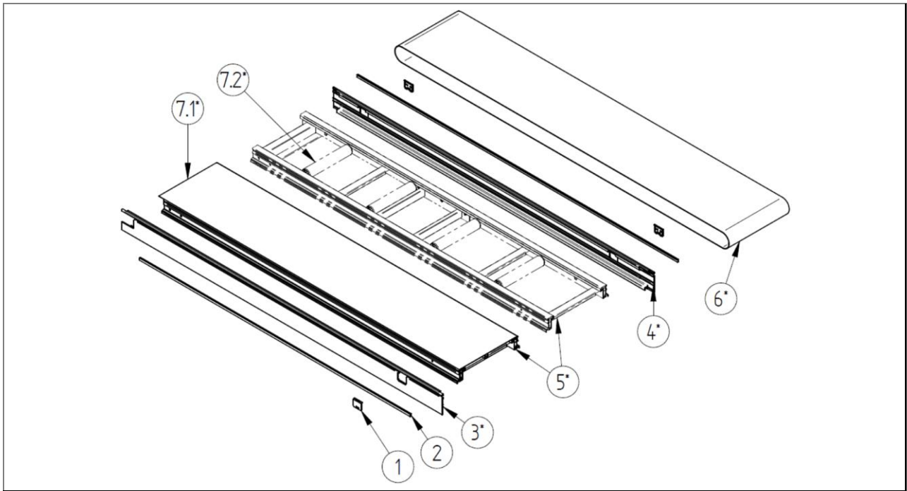
Abb. 80: Stückliste: Förderbandkörper GL0 und GL7 - U.116.0002.00
