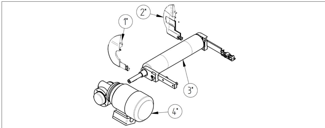
Abb. 100: Stückliste: Flanschantrieb - Antriebsposition 14 - ZZ.900.0149.00
