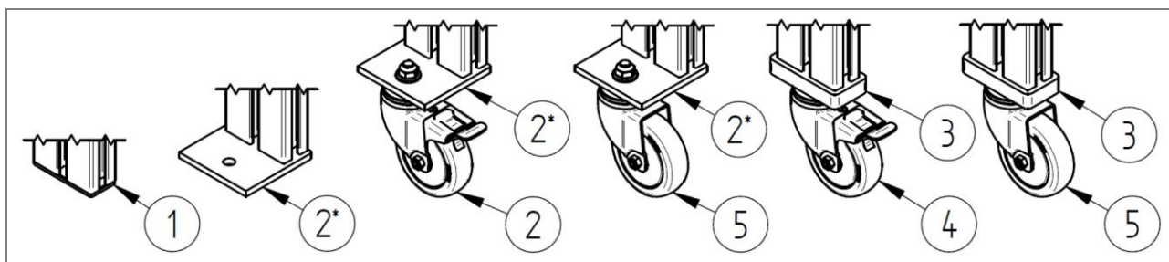
Abb. 126: Stückliste Förderbandabstützung
