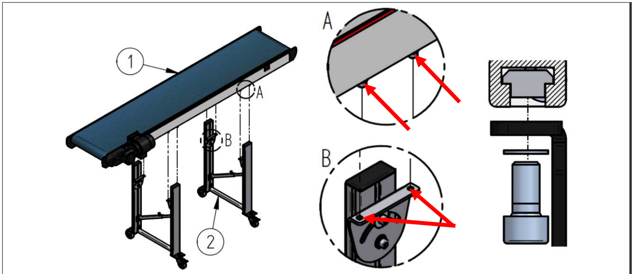
Abb. 41: Montage Förderband mit Untergestell HE 030 – HM 260 (exemplarisch)
