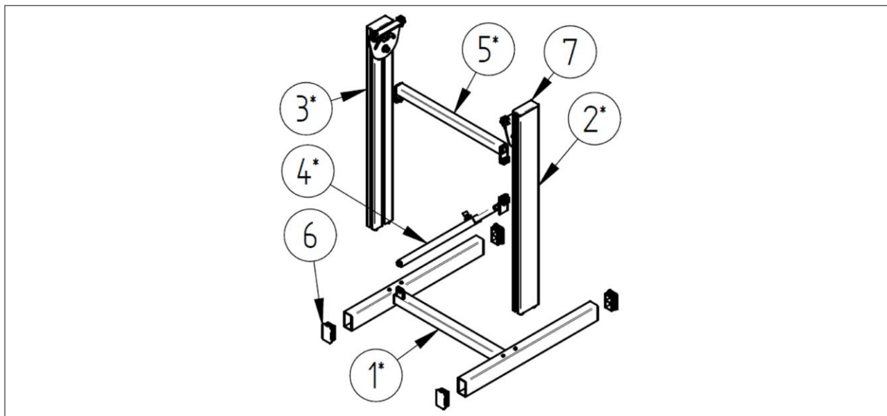
Abb. 129: Stückliste: Untergestell HE 030/HM 260 ZZ.800.0196
