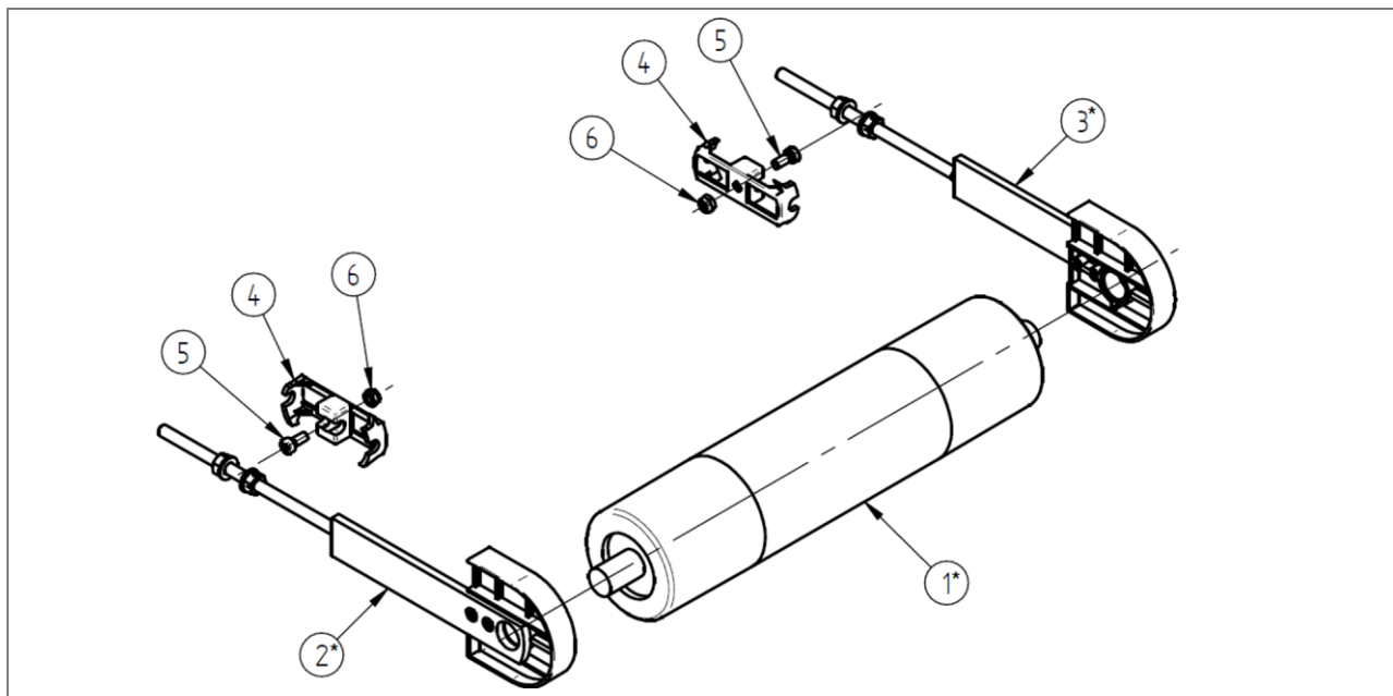
Abb. 83: Stückliste: Multi-Tech Umlenkeinheit Ø80– ZZ.800.0093.03
