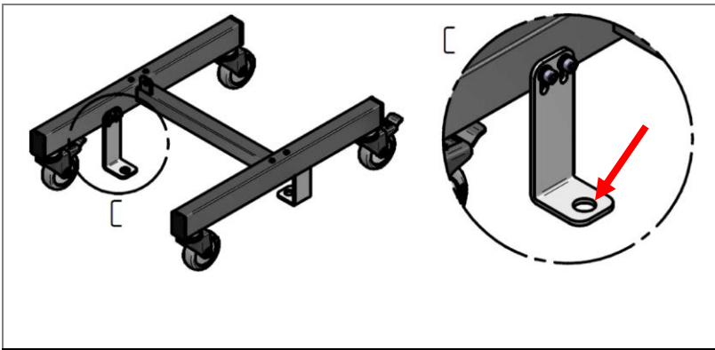
Abb. 57: Bodenbefestigung
