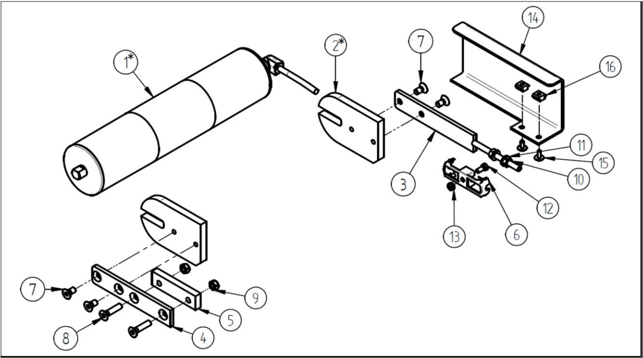
Abb. 107: Stückliste: Trommelmotor - Antriebseinheit - Antriebsposition 23 - ZZ.900.0094.01
