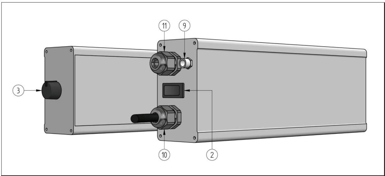
Afb. 7: Besturingseenheid (links vooraanzicht inlaatzijde, rechts achteraanzicht uitlaatzijde)
