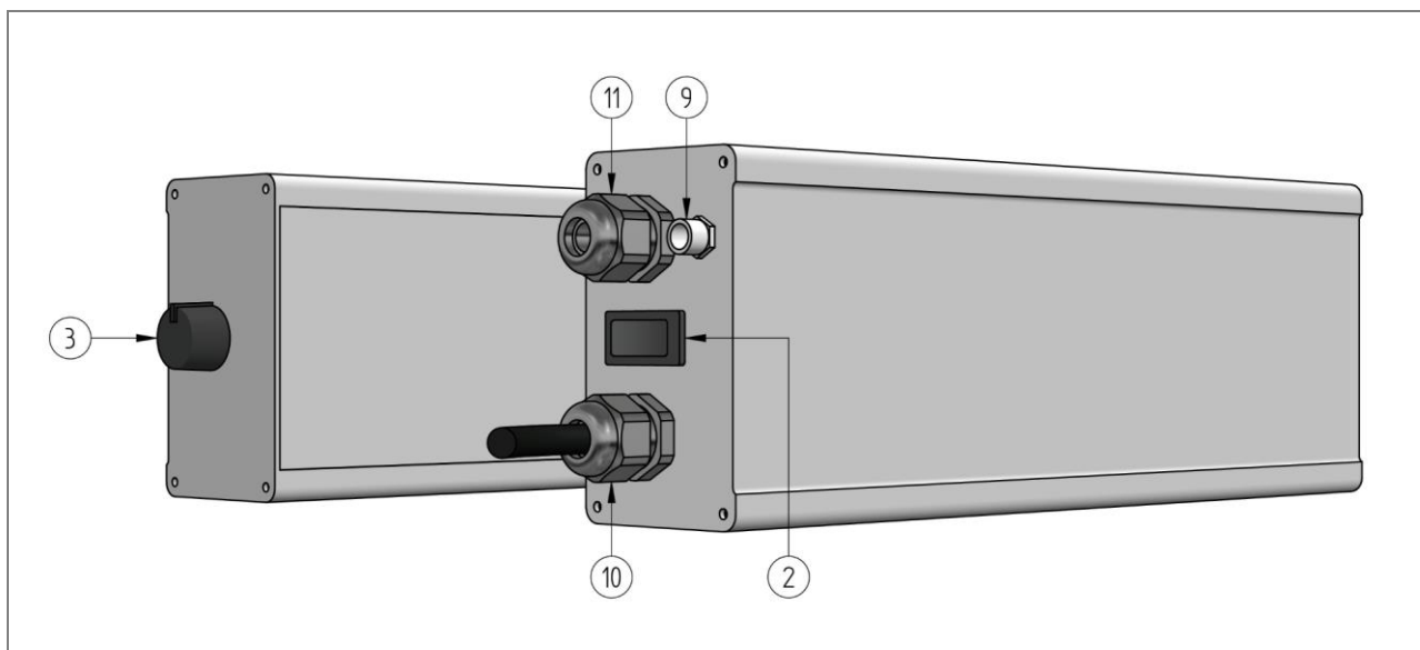
Afb. 11: Besturingseenheid
