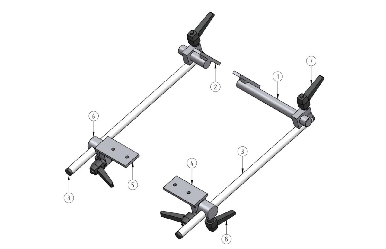
Afb. 17: Opbouwframe SAL/SAR
