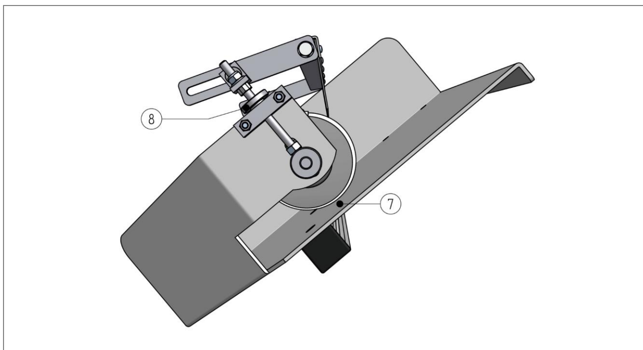
Afb. 6: Zijaanzicht met scheidingsspleet
