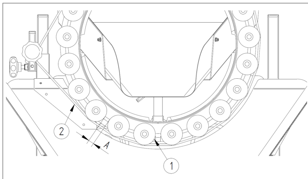
Afb. 4: Scheidingsrollen en de scheidingsspleet daartussen
