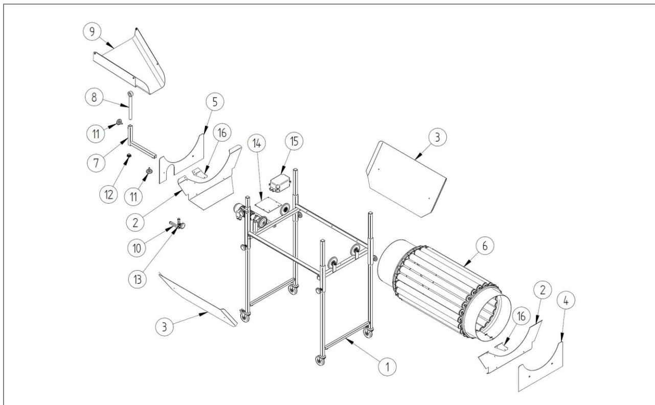
Afb. 19: Stuklijst: Scheidingstroommel met individuele afstelling – ZZ.866.0001
