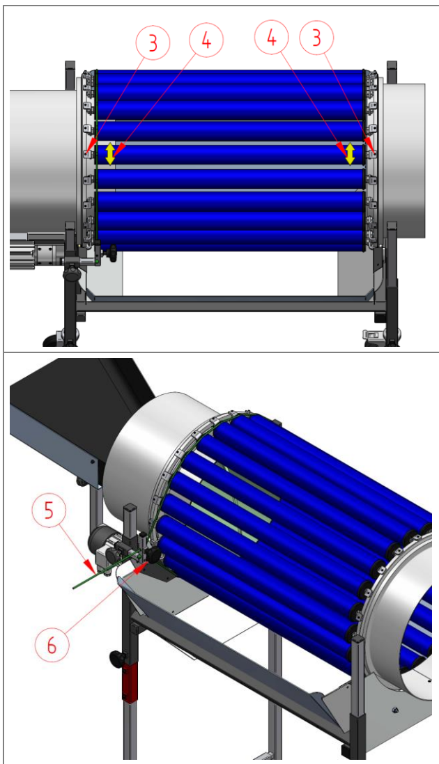
Afb. 10: Scheidingsspleet instellen (individuele afstelling)
