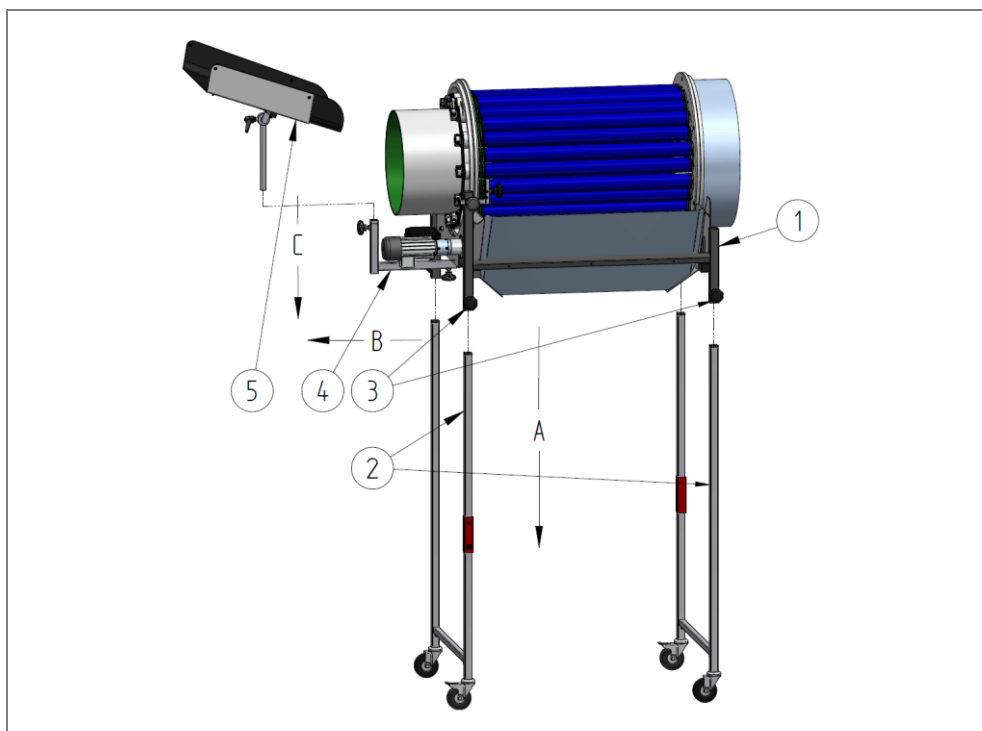
Afb. 9: Montage
