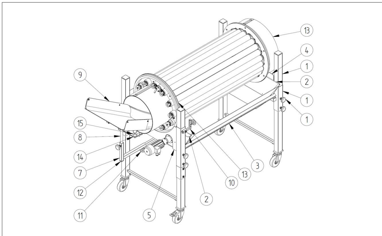
Afb. 23: Stuklijst: Scheidingstroommel PZ 35XX B, versterkt – ZZ.865.0008
