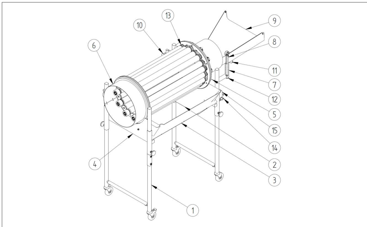
Afb. 20: Stuklijst: Scheidingstroomel PZ 25XX B – ZZ.865.0002
