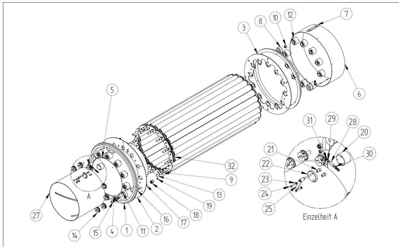
Afb. 26: Stuklijst: Trommelkooi KPZ 35XX B, versterkt – U.865.0006
