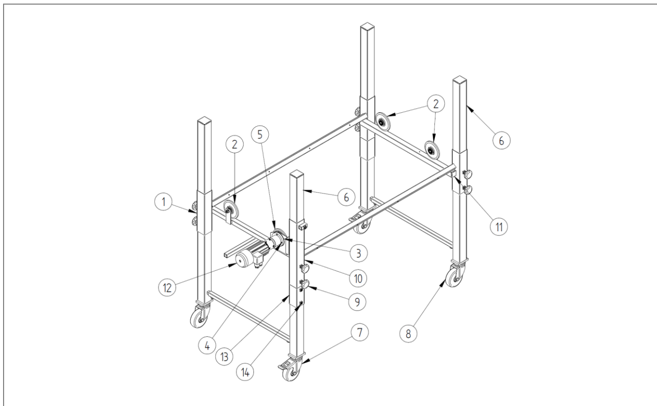
Afb. 29: Stuklijst: Onderstel – versterkt – ZZ.860.0005
