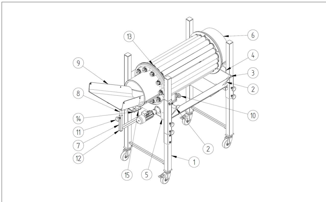
Afb. 22: Stuklijst: Scheidingstroommel PZ 25XX B, versterkt – ZZ.865.0067
