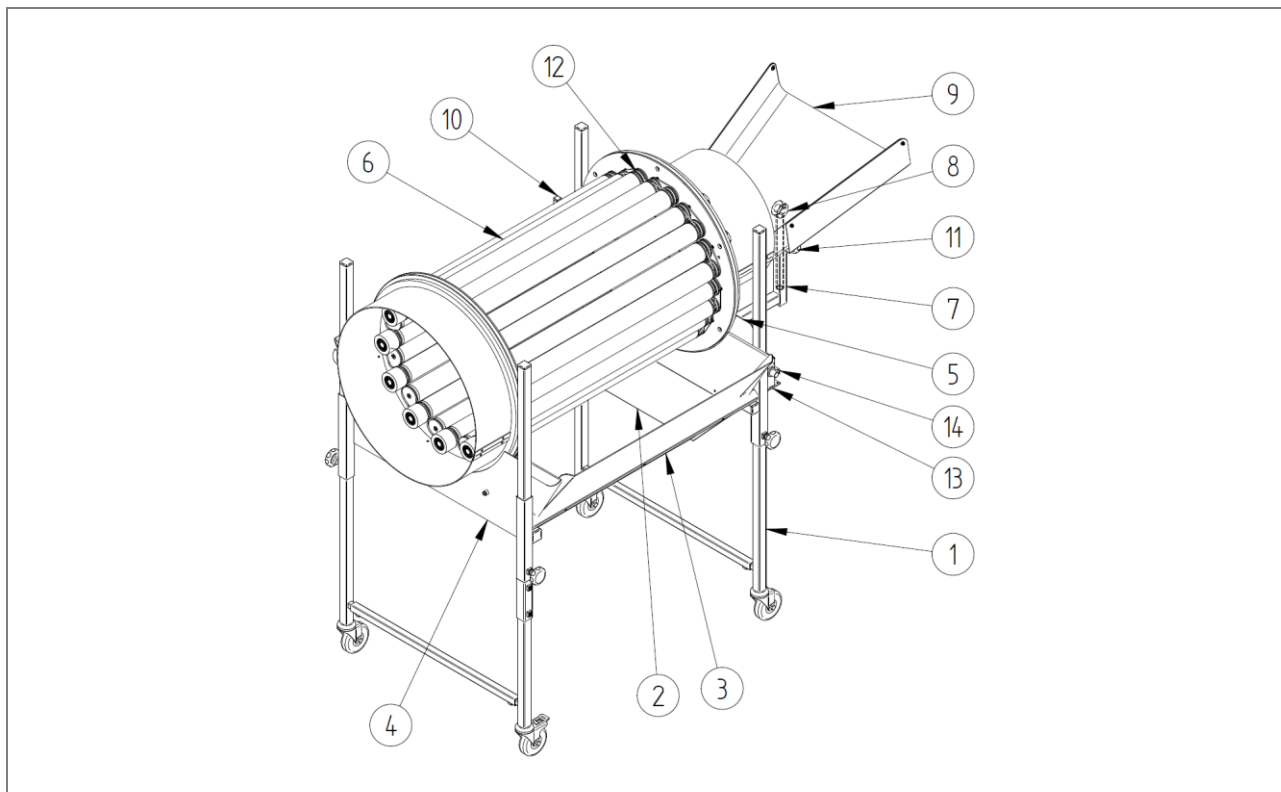
Afb. 21: Stuklijst: Scheidingstroommel PZ 35XX B – ZZ.865.0001
