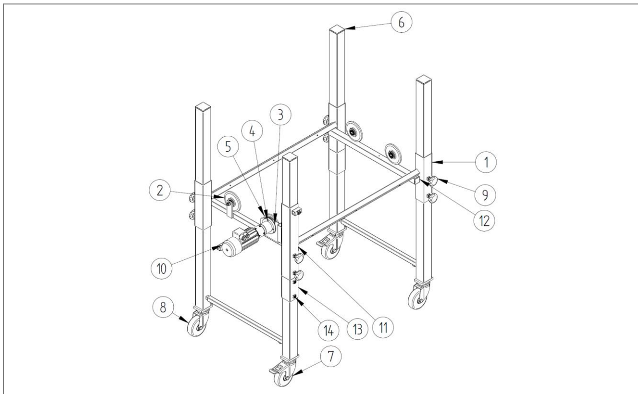
Afb. 28: Stuklijst: Onderstel – versterkt – ZZ.860.0021
