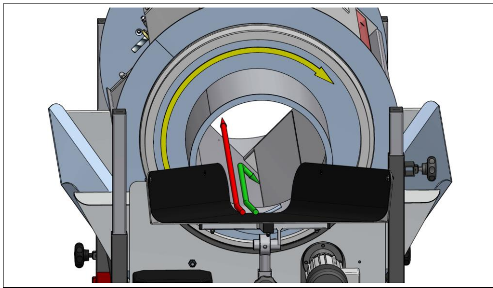
Afb. 2: Werkingsprincipe en doorlooprichting van de delen
