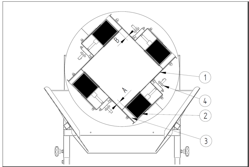
Afb. 4: Uitvalschachten van de scheidingsstrommel in verschillende posities
