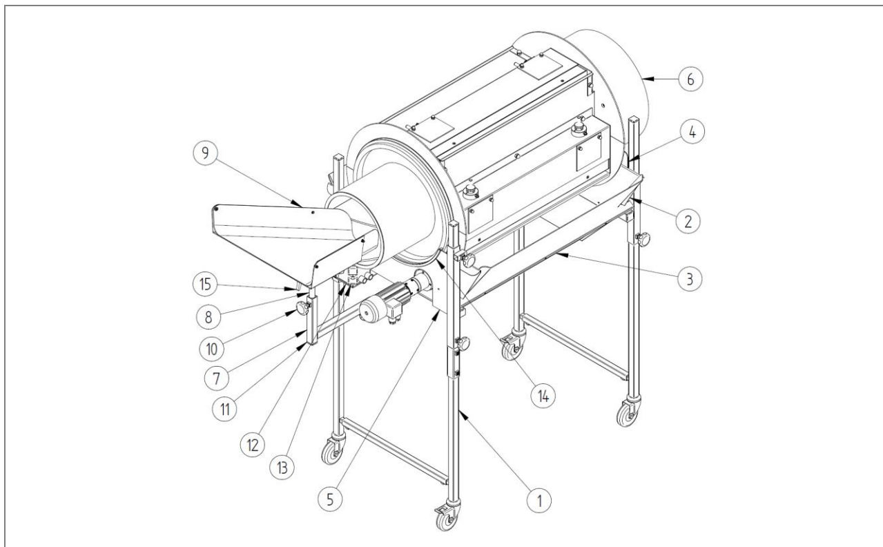
Afb. 17: Stuklijst: Rechthoekige scheidingstrommel R – ZZ.861.0065
