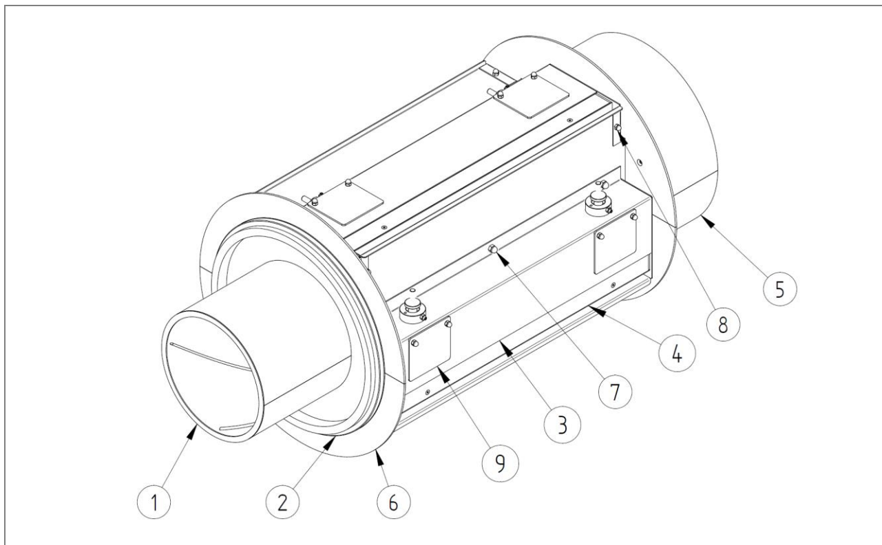
Afb. 18: Stuklijst: Trommelkooi KR – U.867.0062 / U.867.0084
