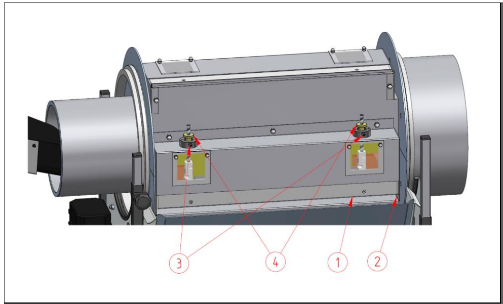
Afb. 9: Scheidingsspleet instellen
