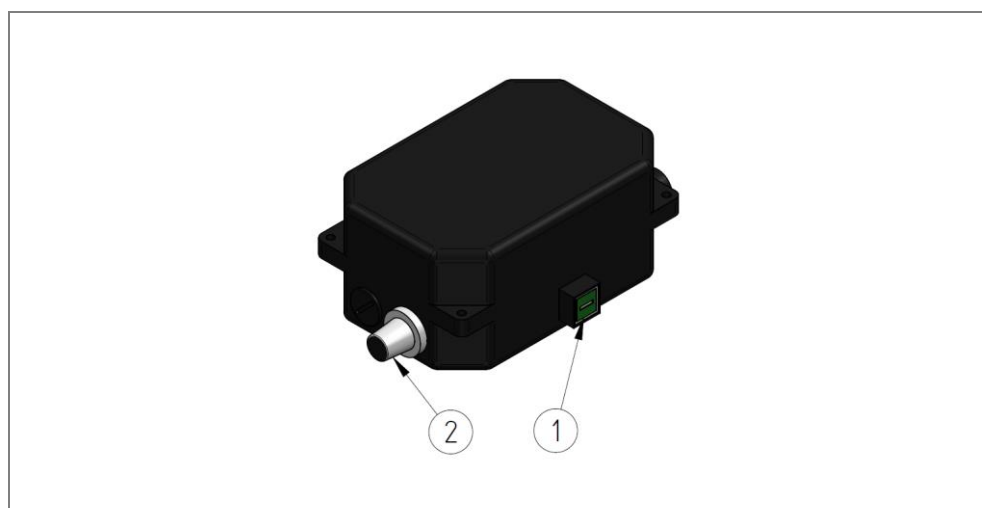
Afb. 14: Bedieningselementen bedrijfssoort "traploos regelbaar"
