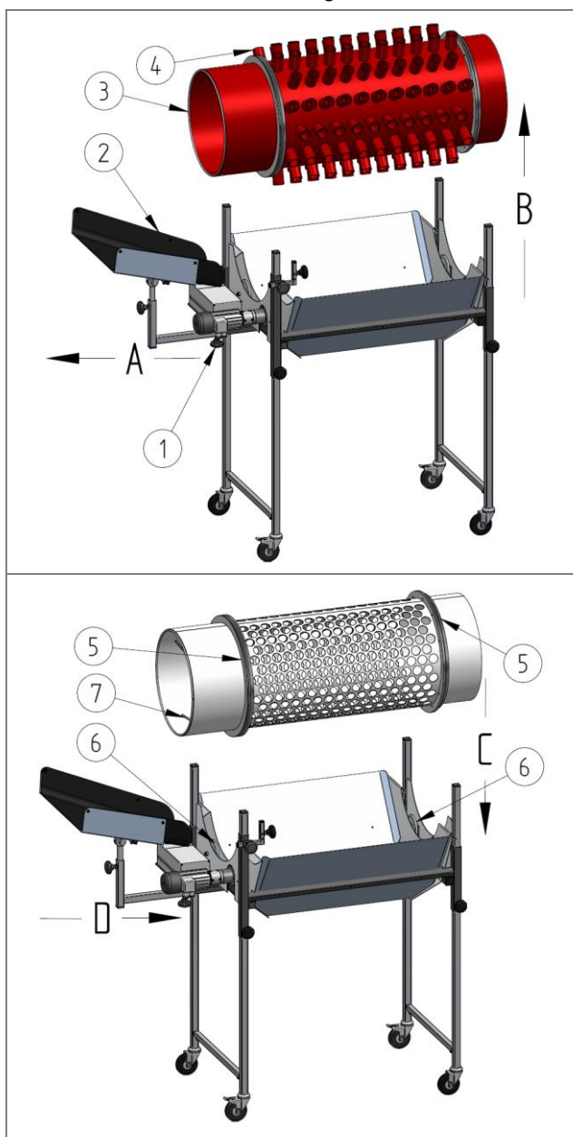
Afb. 11: Vervisseling van de trommelkooi, op de afbeelding zijn als voorbeeld de gaten- en Igel-trommelkooi te zien.
