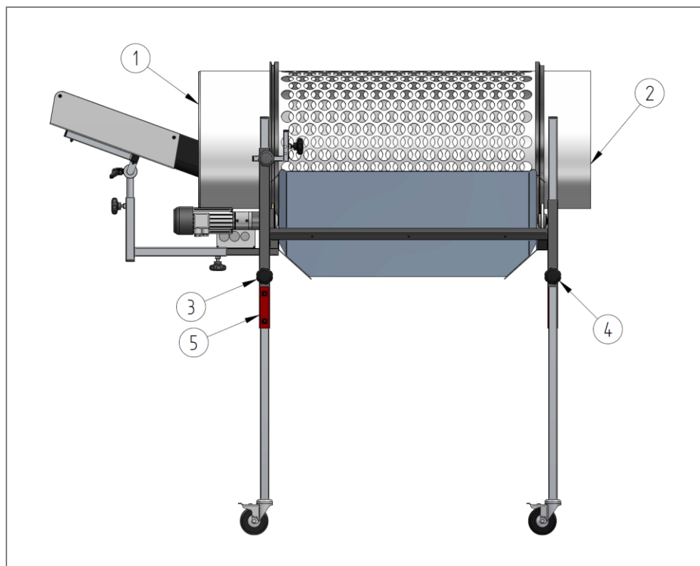
Afb. 9: Instellen van de hoogtes en de hellingshoek
