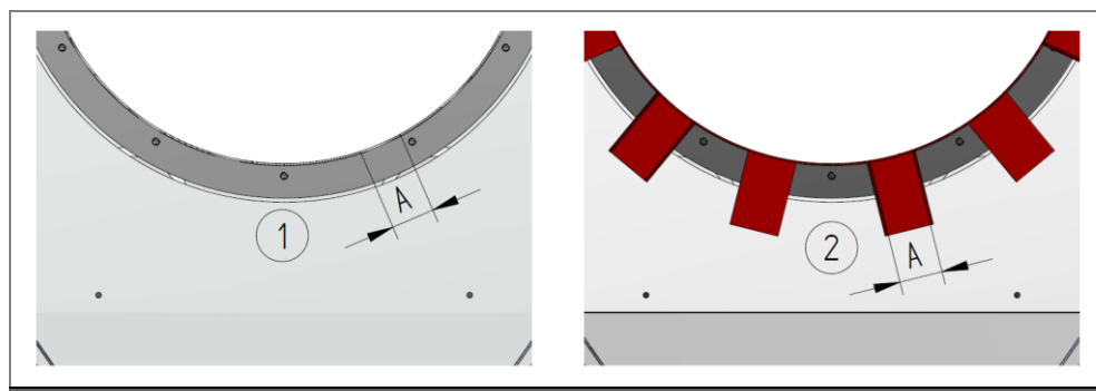
Afb. 4: Gatenscheidingsstrommel
