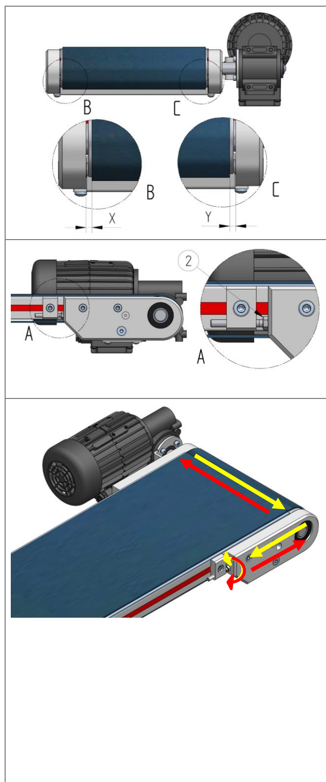
59. ábra: A heveder szinkronfutásának beállítása a hajtási tartományban
