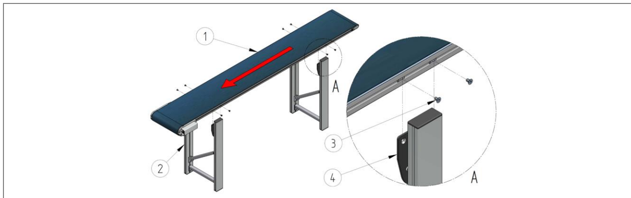
32. ábra: Az AM 1030 alvázass szállítószalag szerelése (példa)
