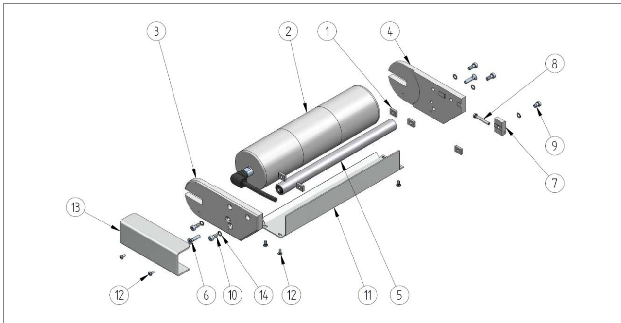
88. ábra: Darabjegyzék: Dobmotor - Hajtásegység/Motoregység - Hajtáspozíció: 1234 - ZZ.900.163
