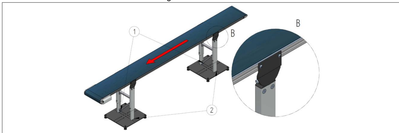
45. ábra: Teljes felépítés - A BE 010 – BM 010 alváz szállítószalag szerelése (példa)
