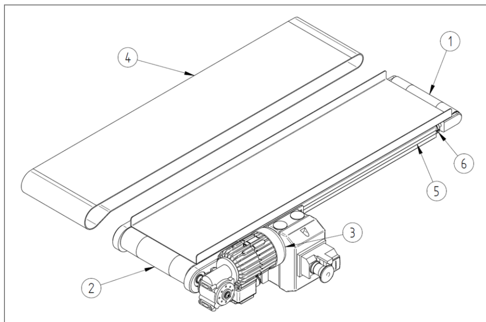
8. ábra: Az egyenes hevederes szállítoszalag (példa) robbantott rajza
