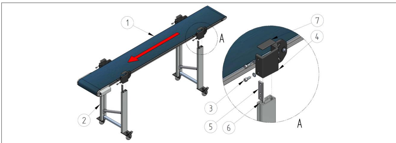
28. ábra: Az AM 140 alváz as szállítószalag szerelése (példa)
