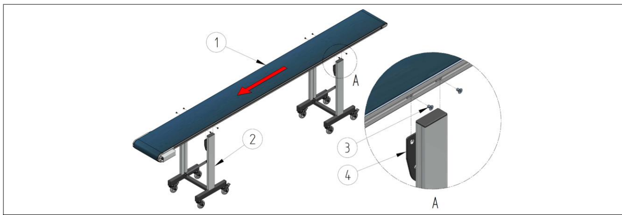
40. ábra: A HE 060 – HM 590 alváz as szállítószalag szerelése (példa)
