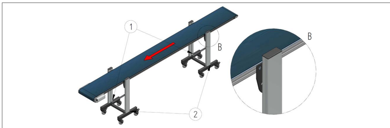
41. ábra: Teljes felépítés - A HE 030 – HM 590 alváz as szállítószalag szerelése (példa)
