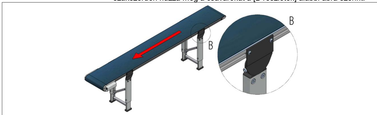
26. ábra: Teljes felépítés - Az AM 920 alvázass szállítószalag szerelése (példa)
