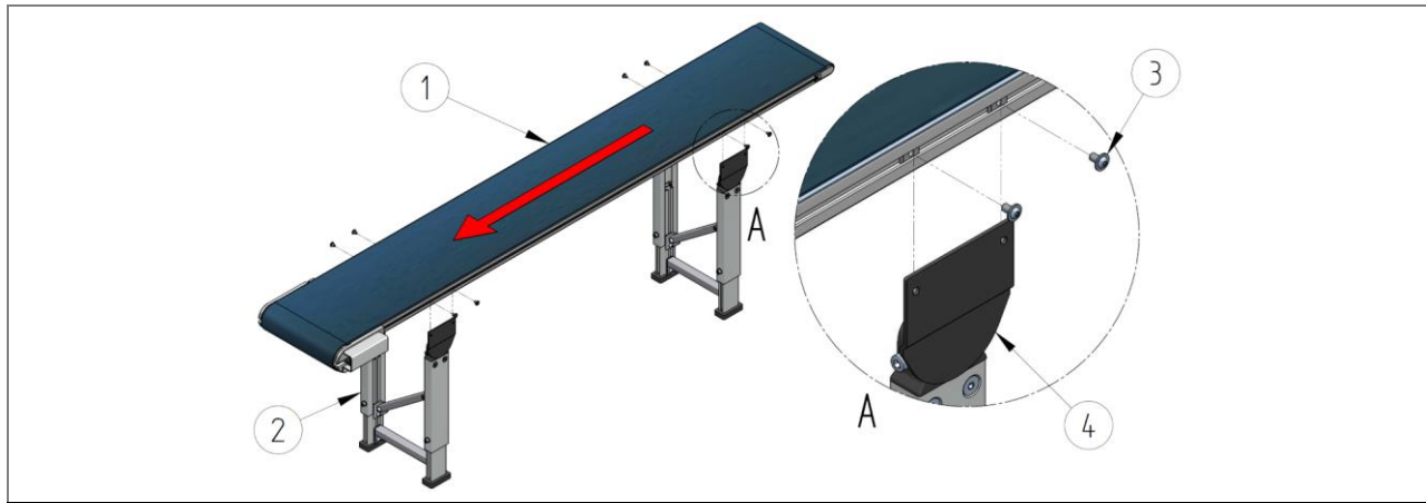
25. ábra: Az AM 920 alvázass szállítószalag szerelése (példa)
