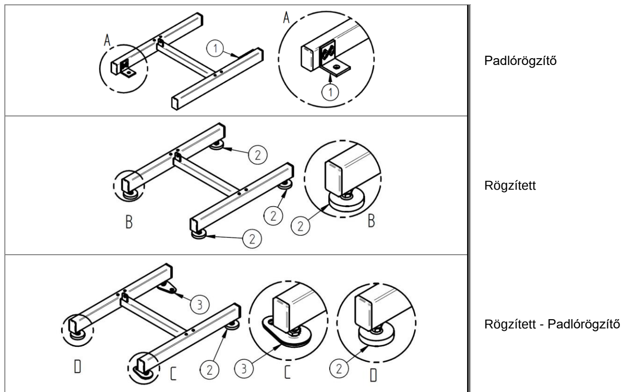
102. ábra: Darabjegyzék: HE/HM alváz felállítási változatok ZZ.982.0068.01
