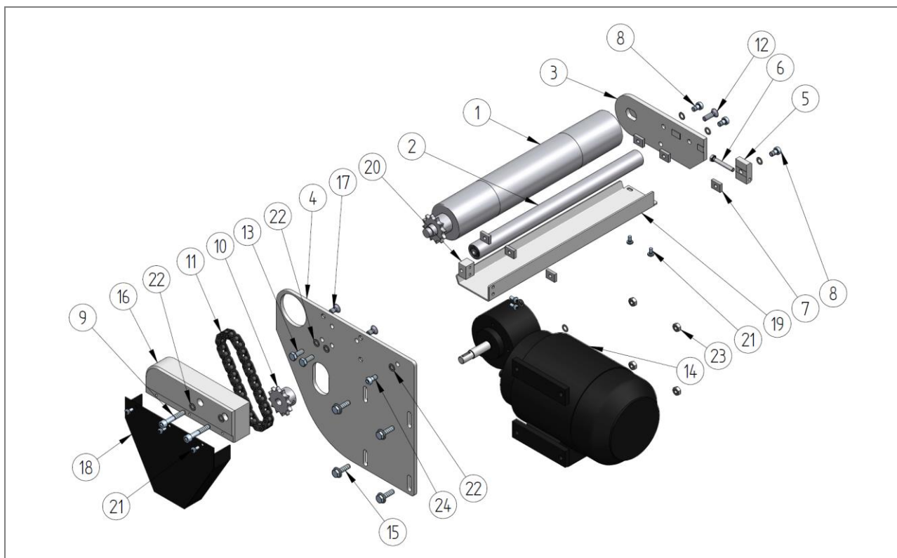
83. ábra: Darabjegyzék: Alsó hajtás - Hajtásegység/Motoregység - Hajtáspozíció: 14 - ZZ.900.0062
