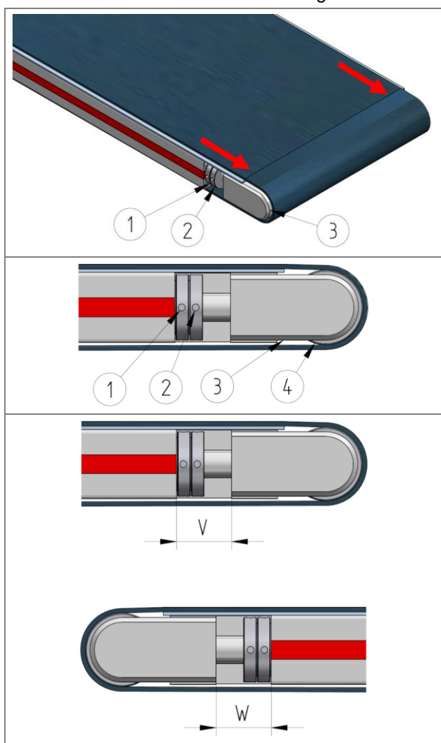
63. ábra: A heveder feszességének beállítása a terelő tartományban
