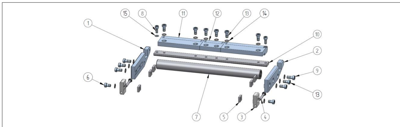
76. ábra: Darabjegyzék: Gördülő késél Ø16– U.910.0030
