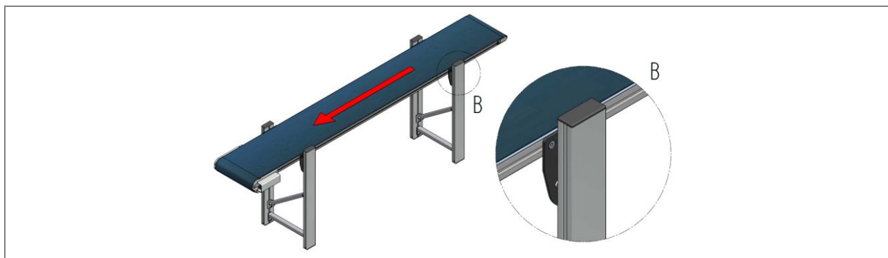
33. ábra: Teljes felépítés - Az AM 1030 alvázass szállítószalag szerelése (példa)
