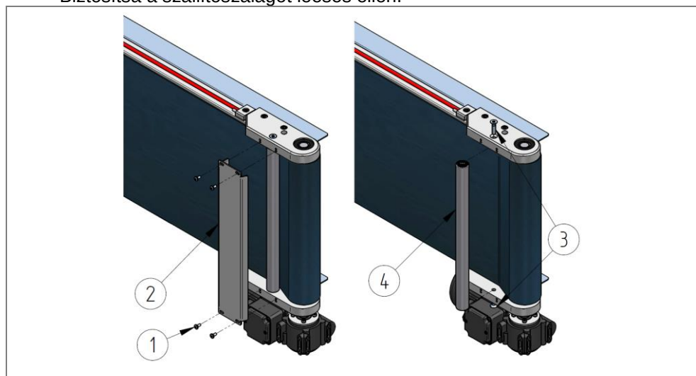
66. ábra: A szűkítőgörgő leszerelése
