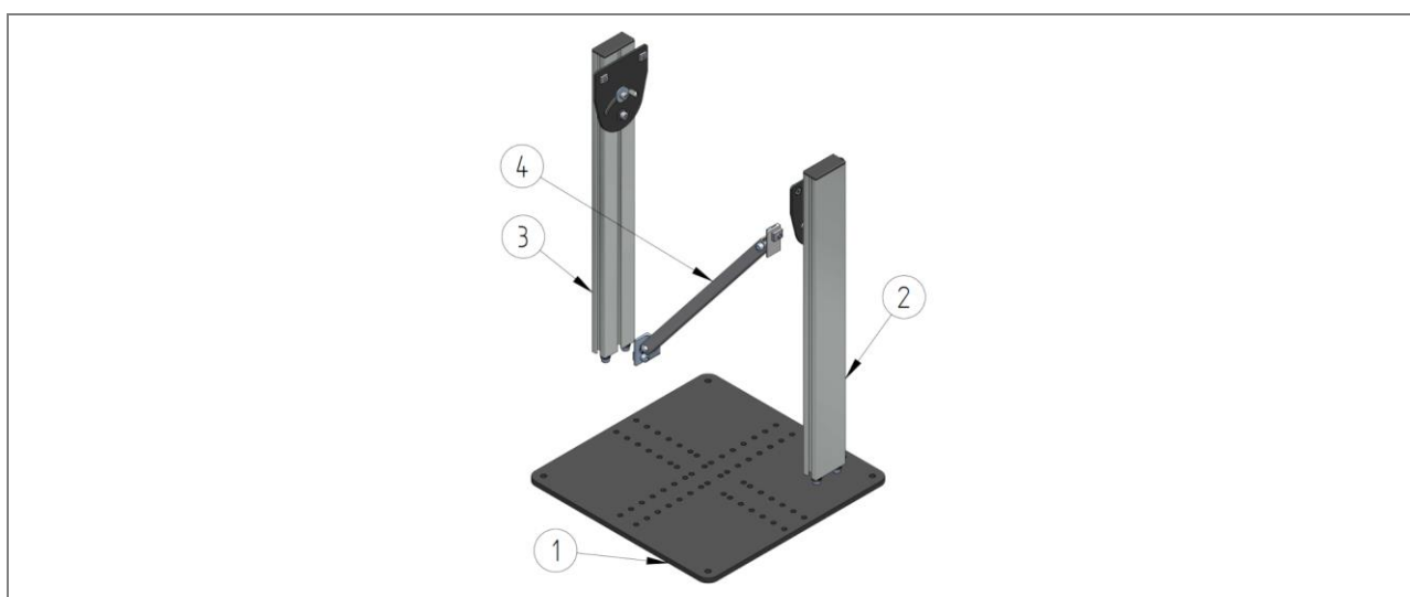
110. ábra: Darabjegyzék: BE 020 - ZZ.982.0079/BM 120 - ZZ.982.0121 alváz
