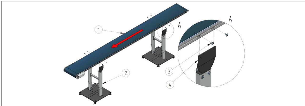
44. ábra: A BE 010 – BM 010 alváz szállítószalag szerelése (példa)
