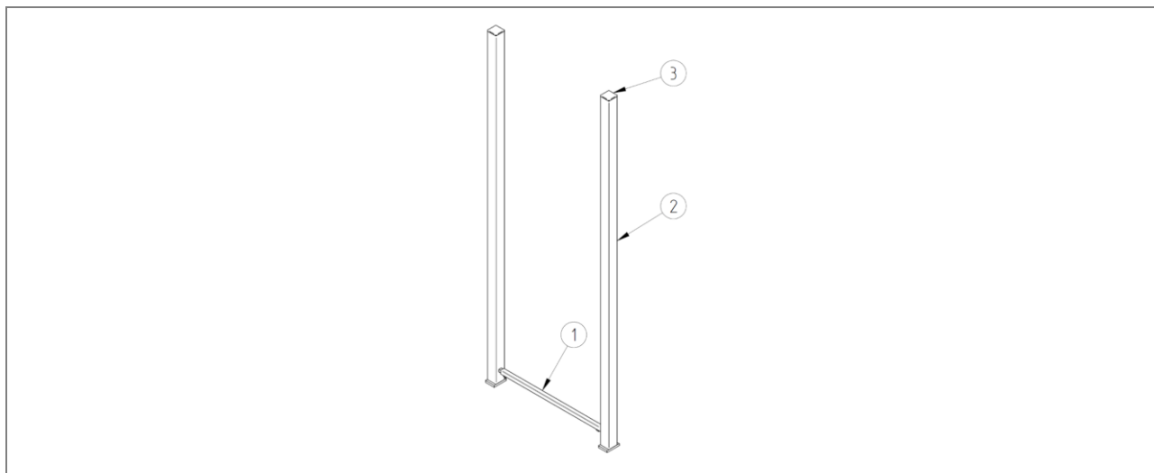
Fig. 25: Lista de piezas: Montante individual – reforzado – U.860.0017
