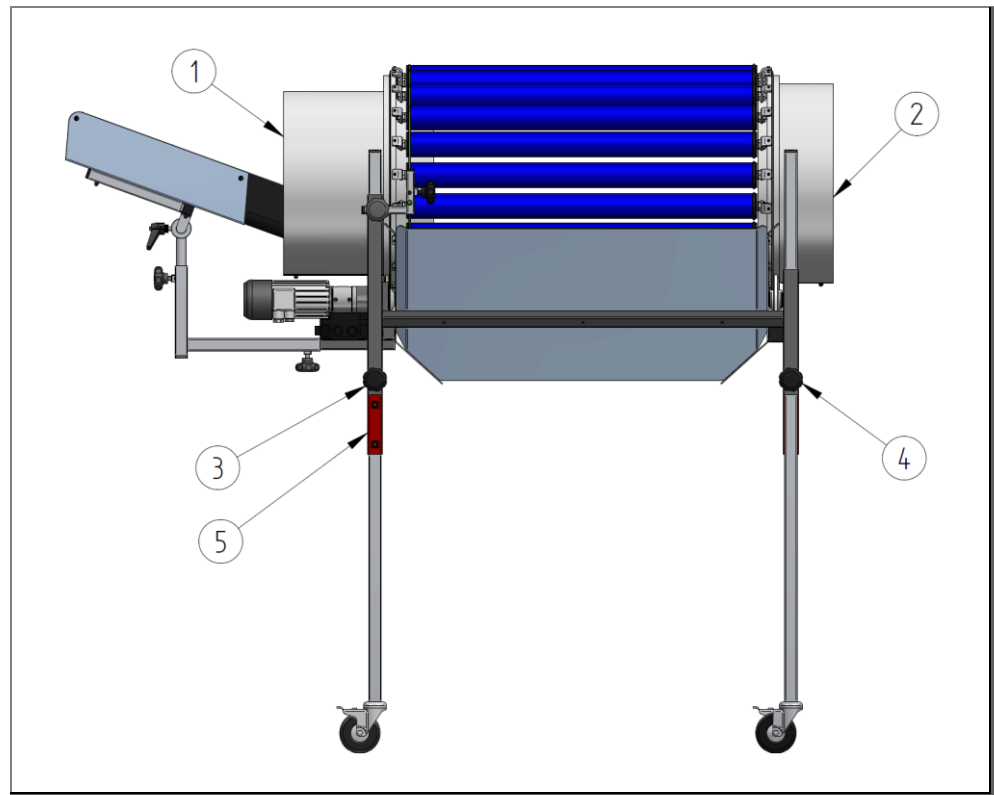
Fig. 11: Ajustar alturas e inclinación
