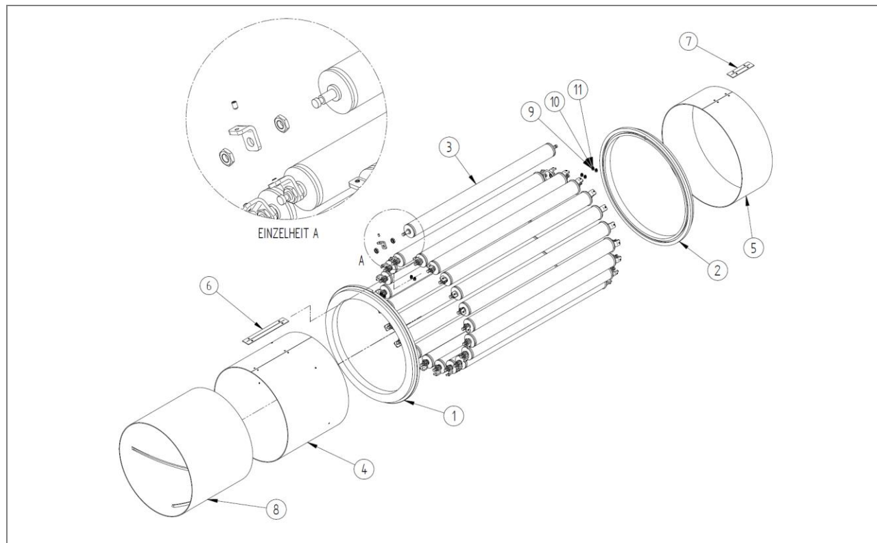
Fig. 21: Lista de piezas: Jaula de tambor 30XX B – U.866.0001
