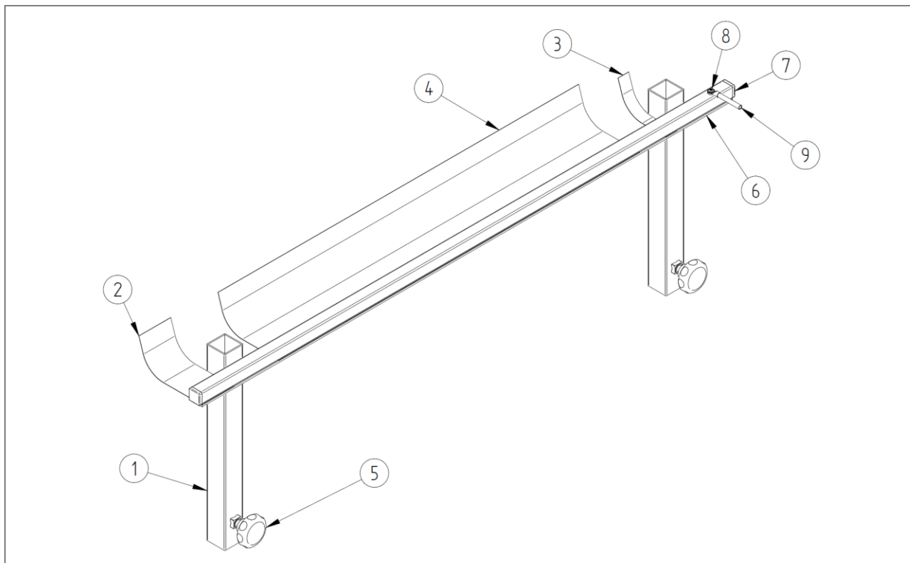
Fig. 26: Lista de piezas Accesorios: Dispositivo antiestático - ZZ.867.0003
