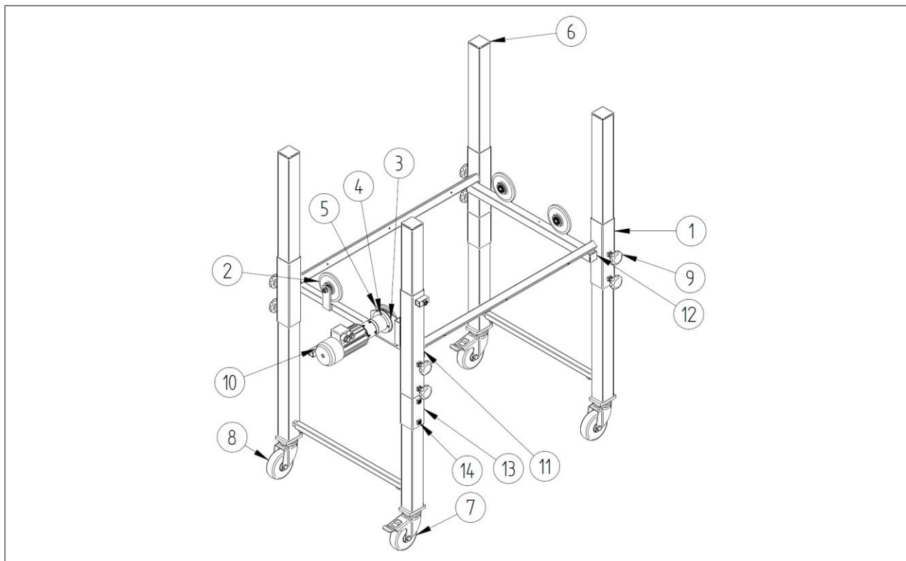
Fig. 23: Lista de piezas: Bastidor inferior – reforzado – ZZ.860.0021
