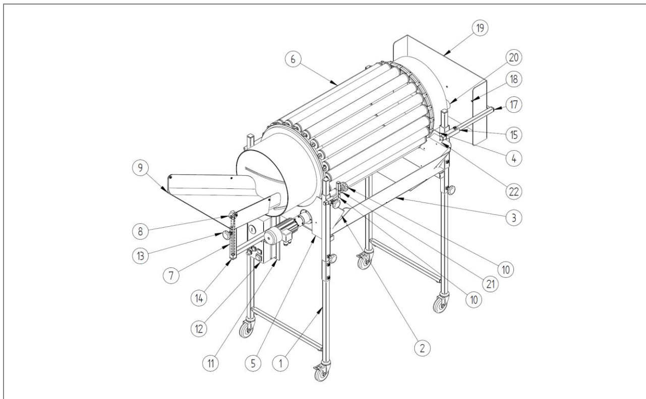
Fig. 20: Lista de piezas: Tambor de desprendimiento con ajuste individual A 30XX B – ZZ.866.0002
