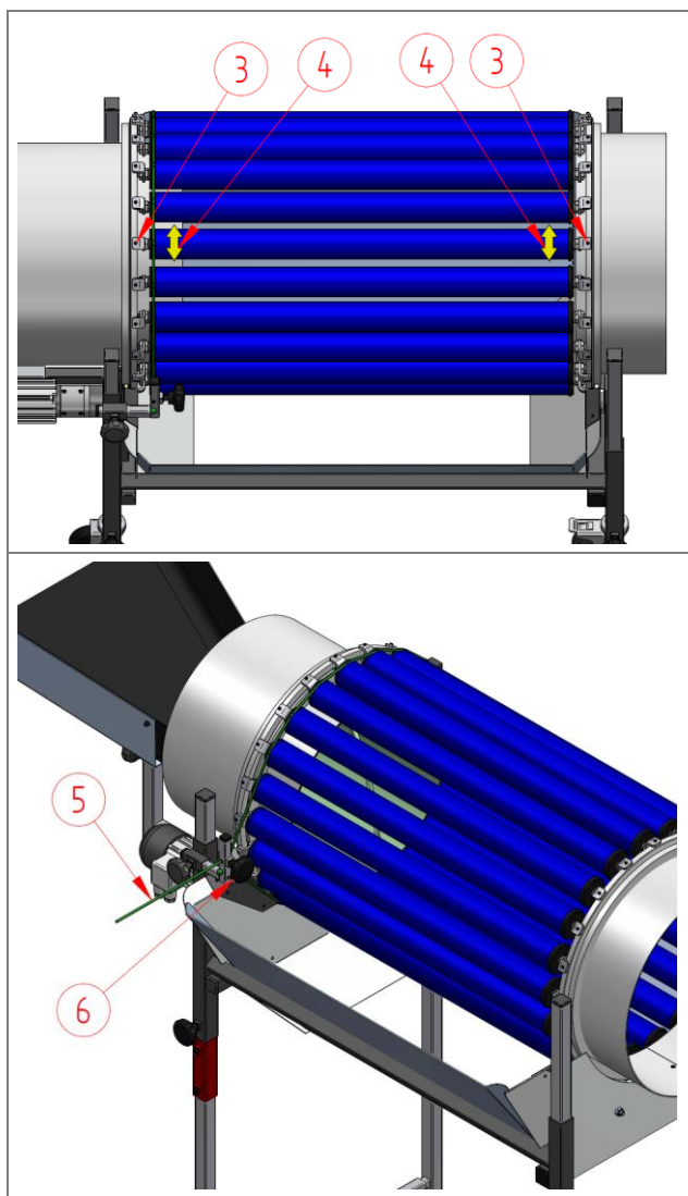
Fig. 10: Ajustar la ranura de separación (ajuste individual)
