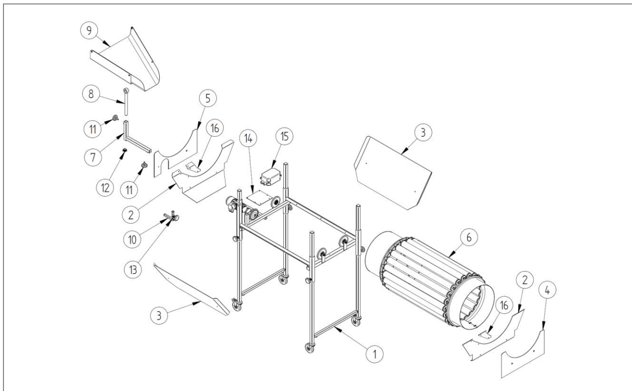
Rys. 19: Lista części: Bęben separacyjny z pojedynczą regulacją– ZZ.866.0001
