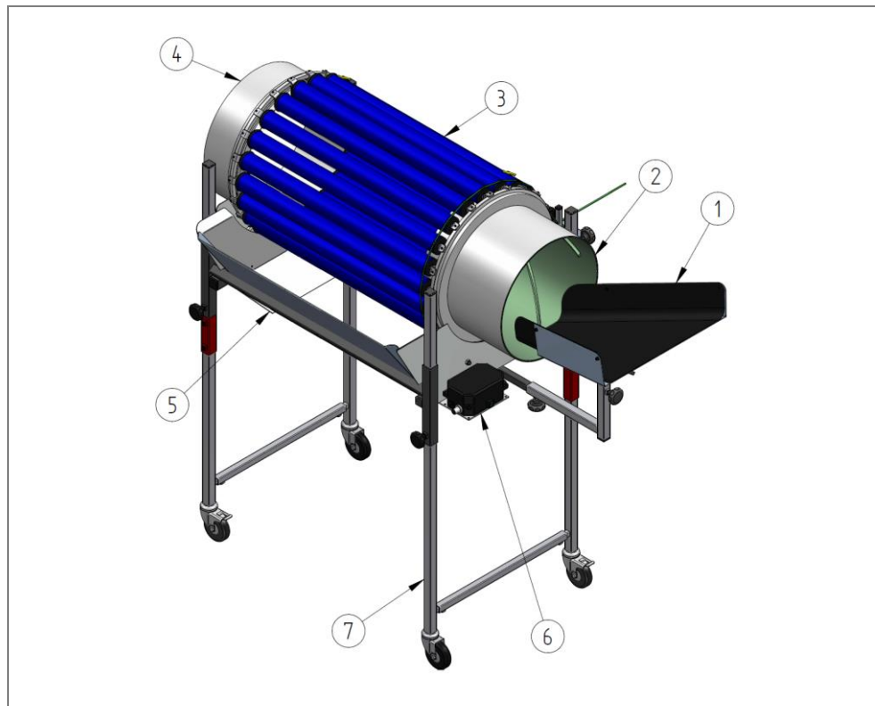
Rys. 3: Bęben separacyjny z pojedynczą regulacją
