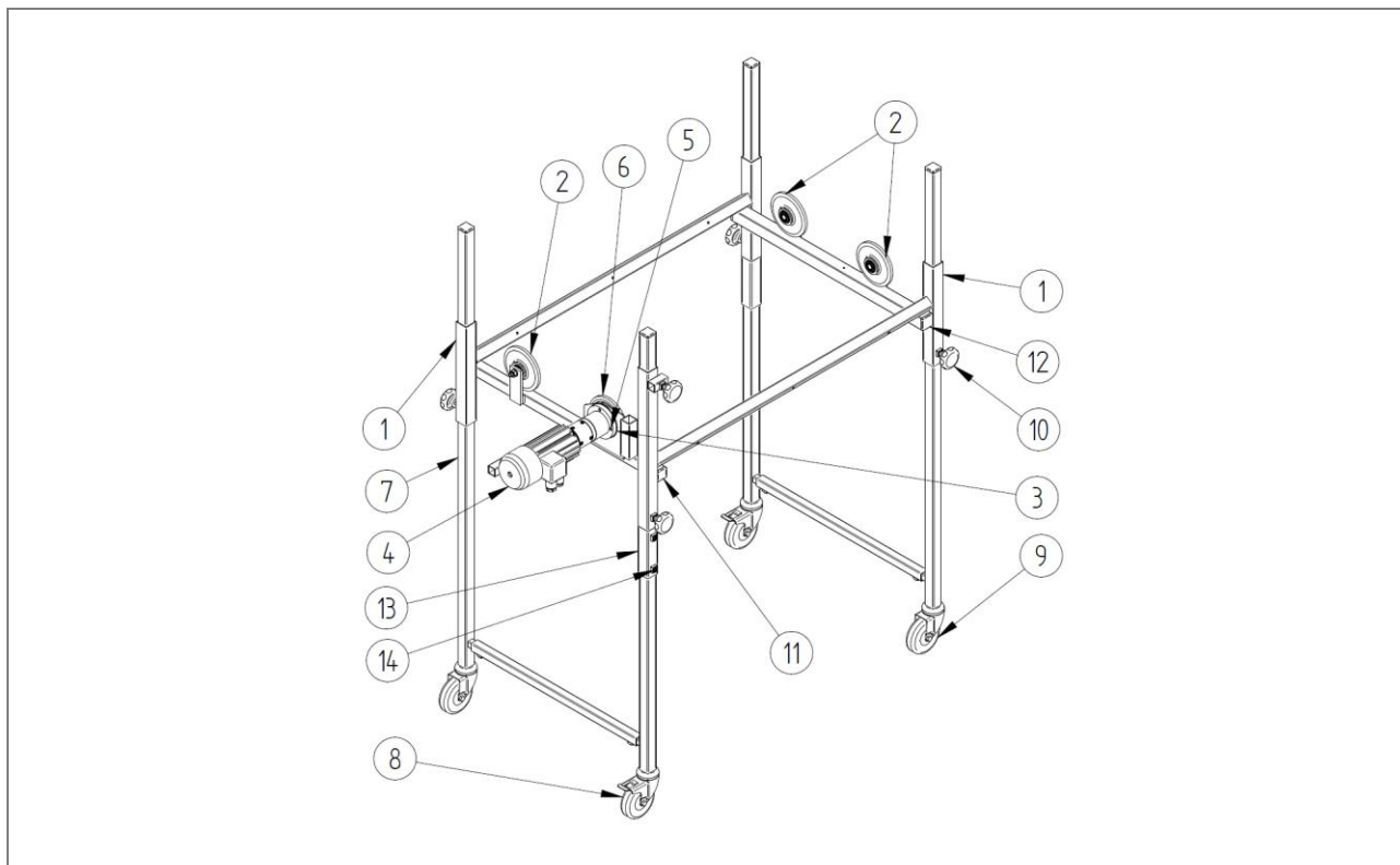
Rys. 22: Lista części: Rama podstawy – bęben separacyjny – ZZ.860.0003
