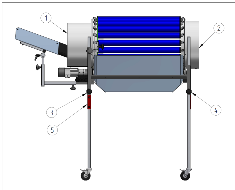
Rys. 11: Ustawianie wysokości i nachylenia
