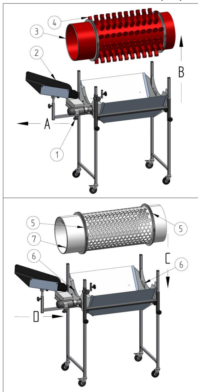
Rys. 14: Wymiana kosza bębna została przedstawiona przykładowo dla kosza bębna otworowego i jeżowego.
