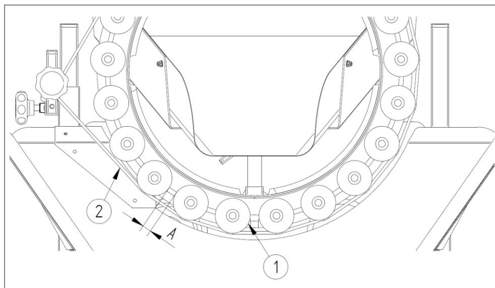
Rys. 4: Rolki separacyjne i szczelina separacyjna pomiędzy nimi
