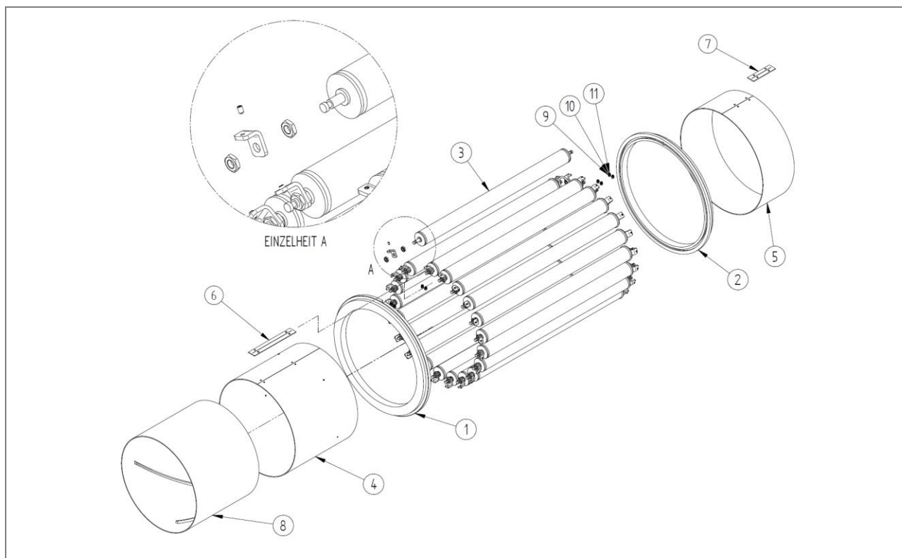
Rys. 21: Lista części: Kosz bębna 30XX B – U.866.0001
