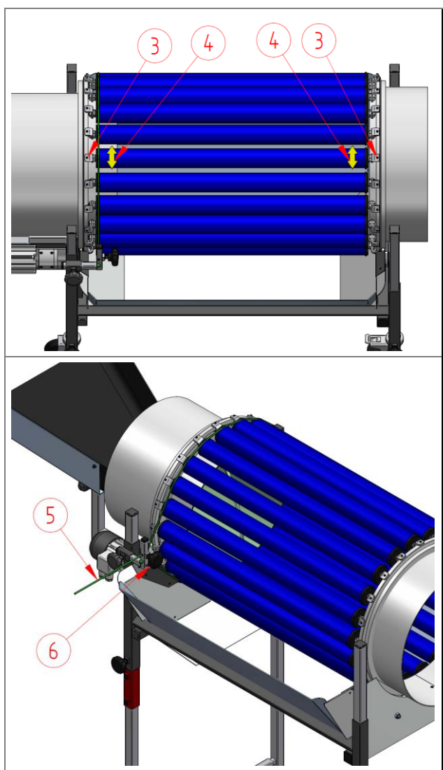
Rys. 10: Ustawianie szczeliny separacyjnej (pojedyncza regulacja)
