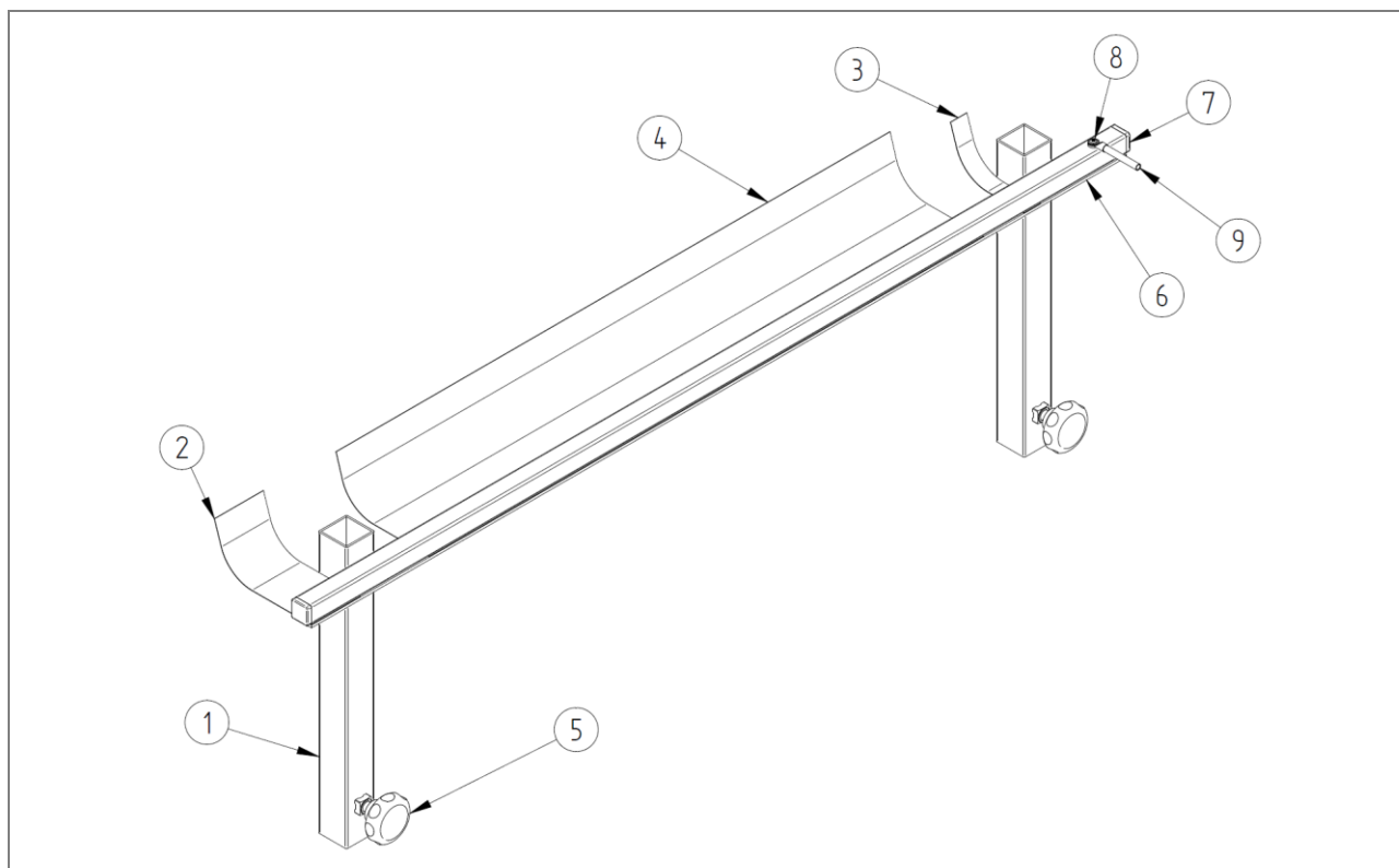
Rys. 26: Akcesoria, lista części: Układ antystatyczny – ZZ.867.0003
