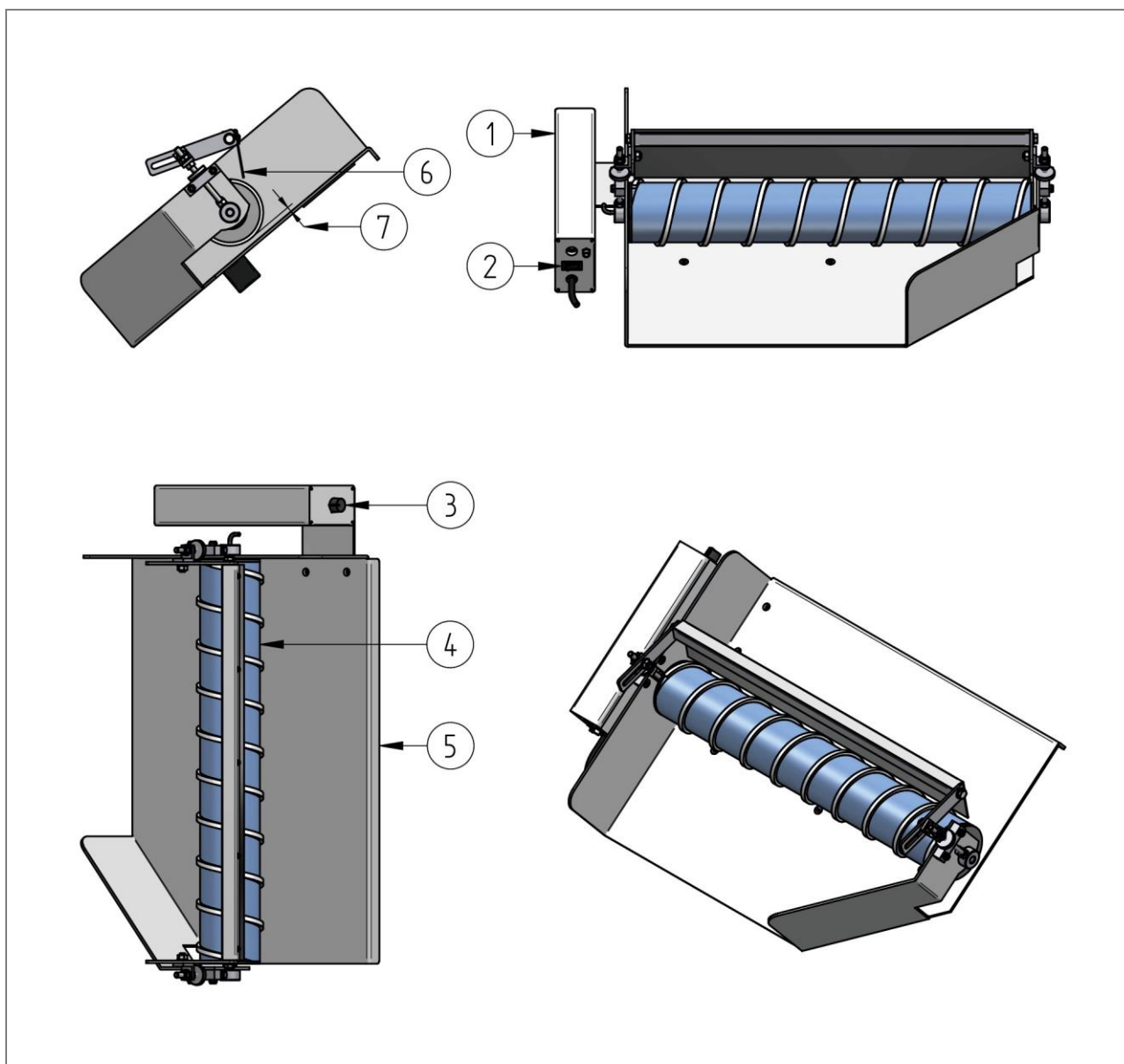
Rys. 3: Widok ogólny separatora ślimakowego
