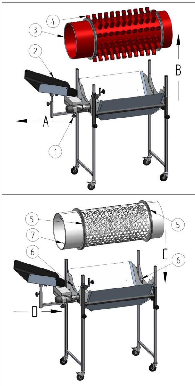
Rys. 11: Wymiana kosza bębna została przedstawiona przykładowo dla kosza bębna otworowego i żeżowego.
