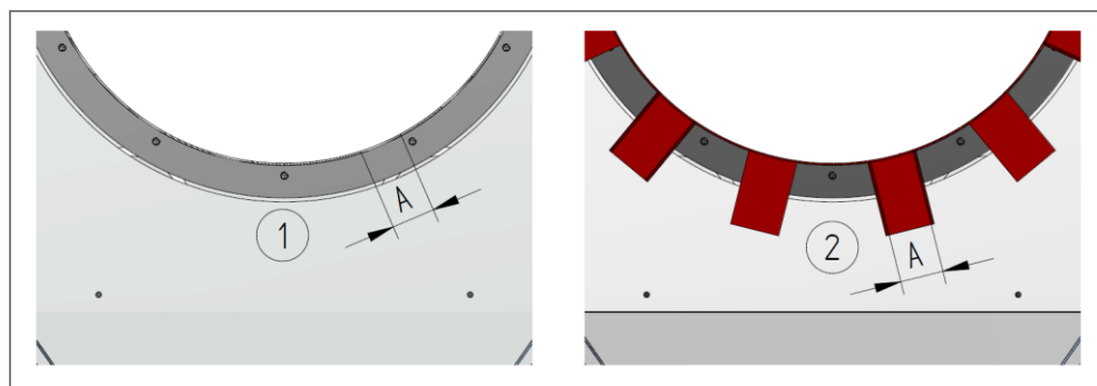
Rys. 4: Bęben separacyjny otworowy/jeżowy
