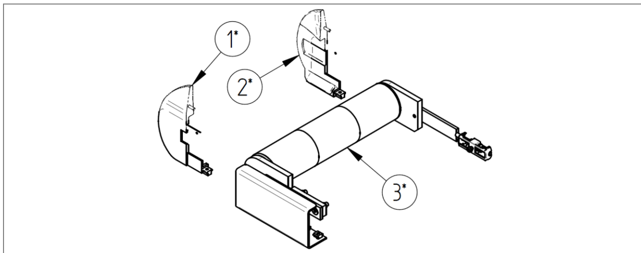
Rys. 104: Lista części: Elektrobęben – Pozycja napędu 14 – ZZ.900.0151.00
