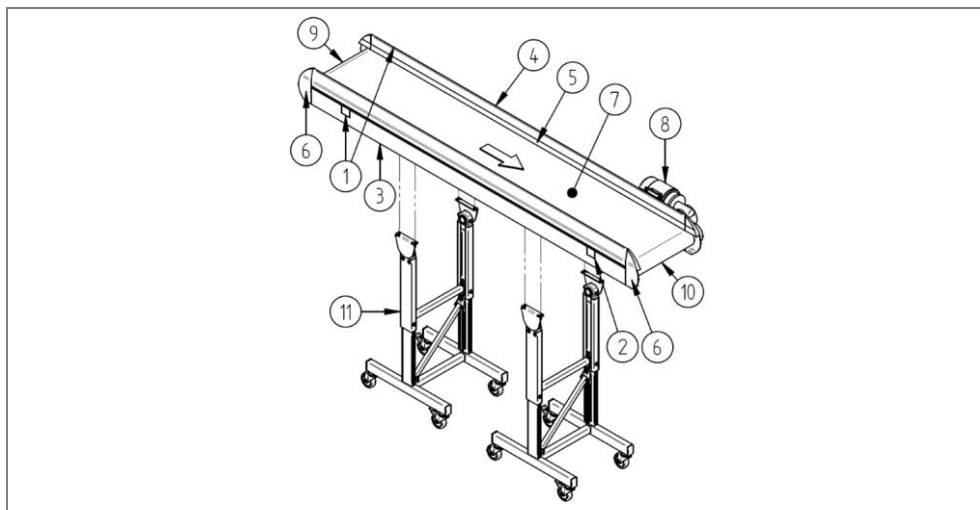
Rys. 69: Przenośnik taśmowy – nazwy elementów
