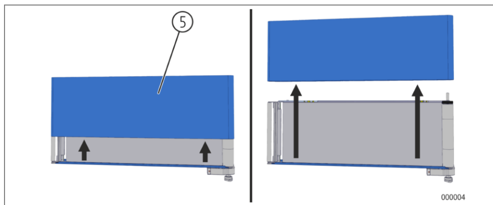
Rys. 73: Ściąganie taśmy
