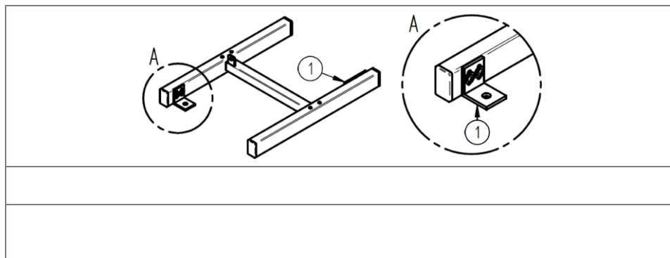
Rys. 130: Lista części: Rama podstawy, warianty ustawienia HE/HM ZZ.982.0068.01
