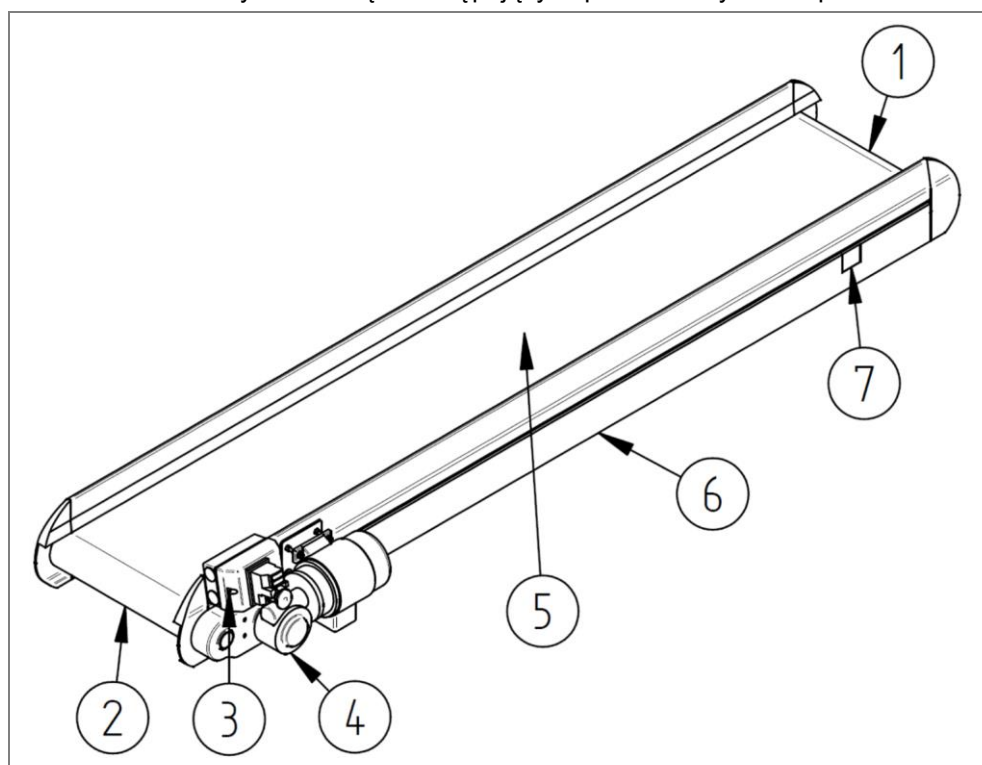
Rys. 2: Prosty przenośnik taśmowy (przykładowy)
