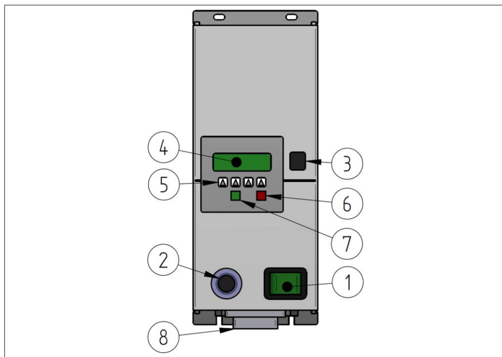
Rys. 61: Sterownik kombi
