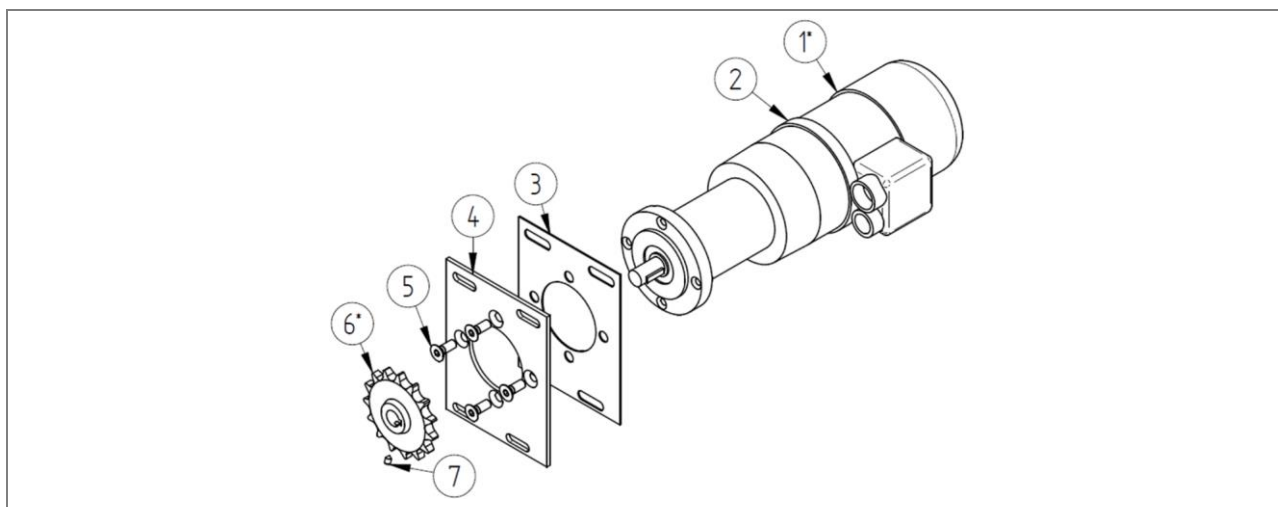
Rys. 99: Lista części: Napęd wewnętrzny – Jednostka silnika – Pozycja napędu 14 – T.900.0004.00/T.900.0005.00
