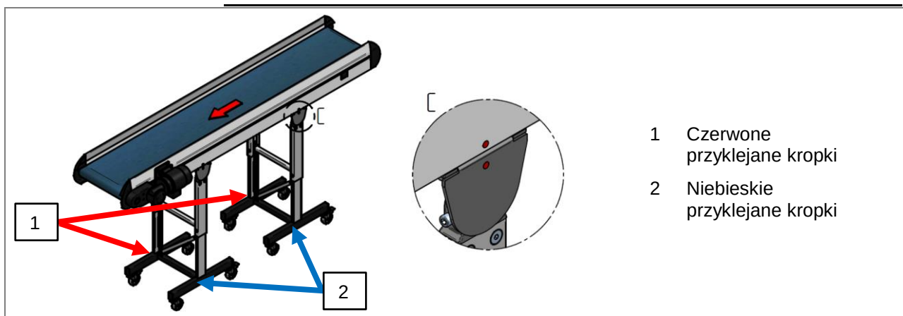
Rys. 46: Kompletna konstrukcja, montaż przenośnika taśmowego z ramą podstawy HE 010 – HM 010 (przykładowy)
