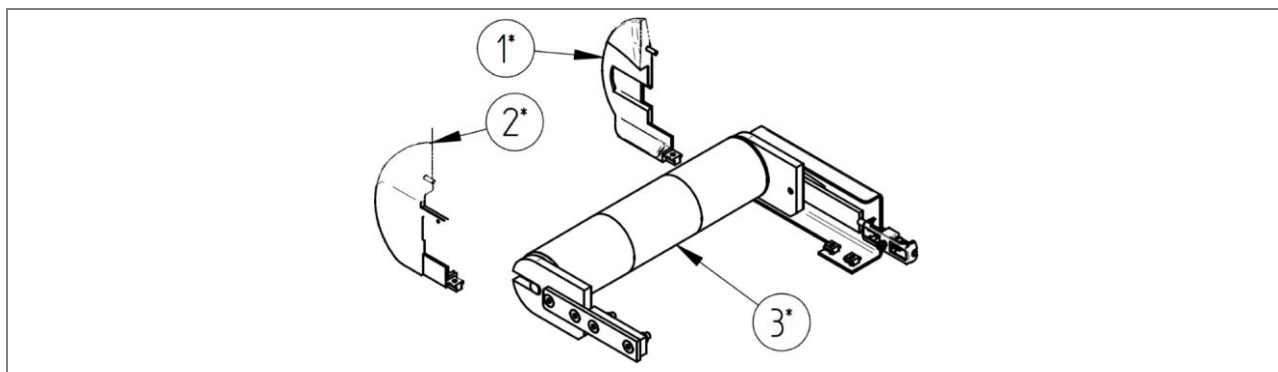
Rys. 106: Lista części: Elektrobęben – Pozycja napędu 23 – ZZ.900.0152.00
