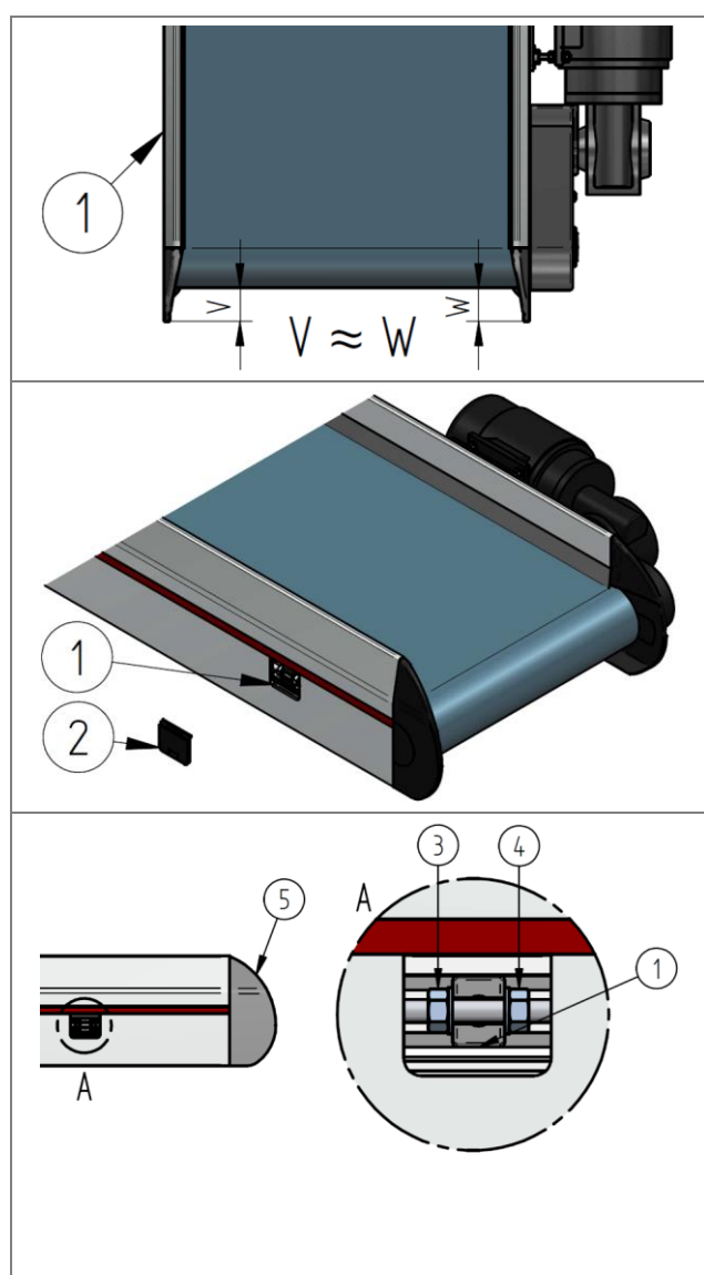
Rys. 67: Sprawdzanie i ustawianie kąta prostego rolki napędowej
