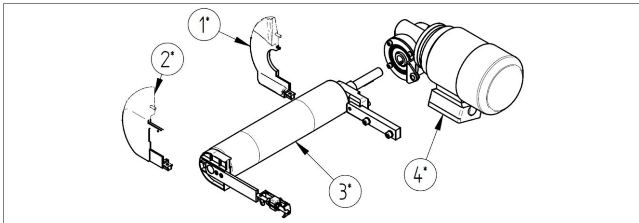
Rys. 102: Lista części: Napęd kołnierowy – Pozycja napędu 23 – ZZ.900.0150.00
