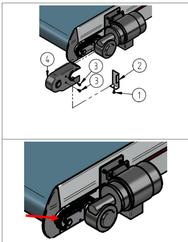
Rys. 77: Smarowanie łańcucha
