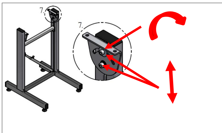
Rys. 52: Montaż ramy podstawy – HE 260 / HM 260
