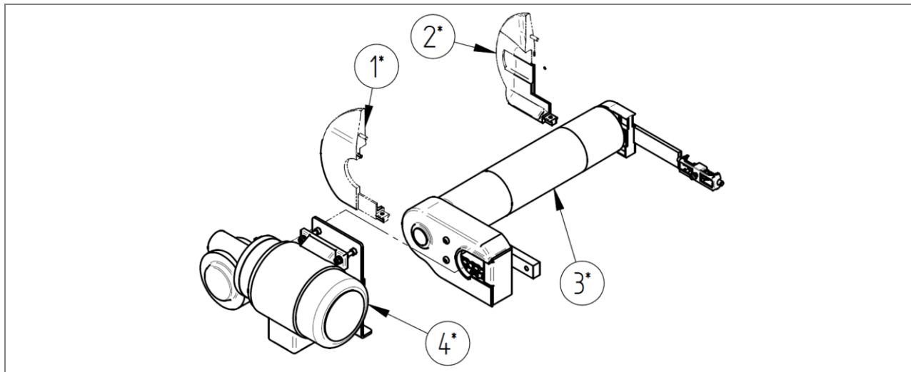
Rys. 88: Lista części: Napęd zewnętrzny – Pozycja napędu 14 - ZZ.900.0142.00
