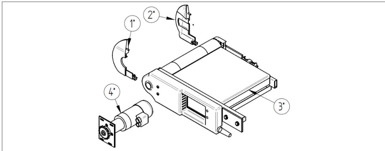
Rys. 97: Lista części: Napęd wewnętrzny – Pozycja napędu 14 - ZZ.900.0145.00
