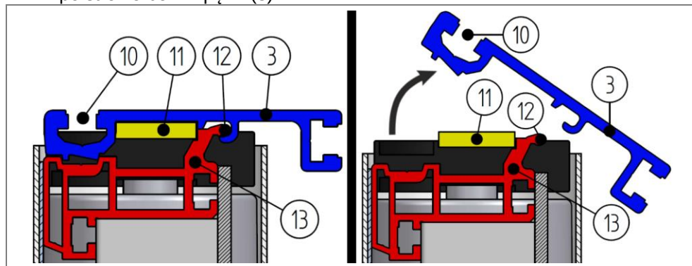
Rys. 72: Wyjmowanie profilu prowadzącego
