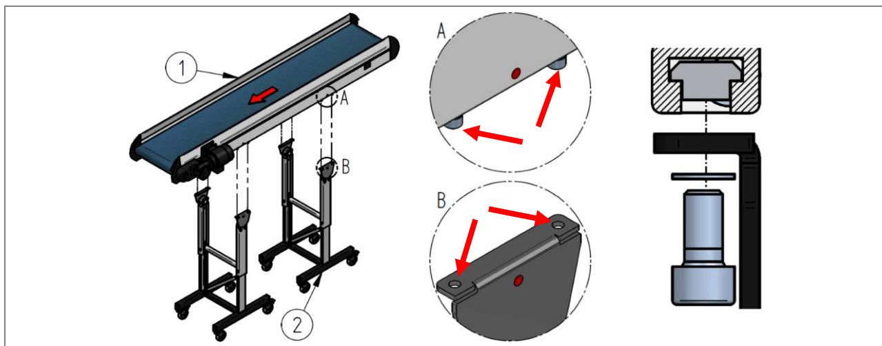
Rys. 45: Montaż przenośnika taśmowego z ramą podstawy HE 010 – HM 010 (przykładowy)
