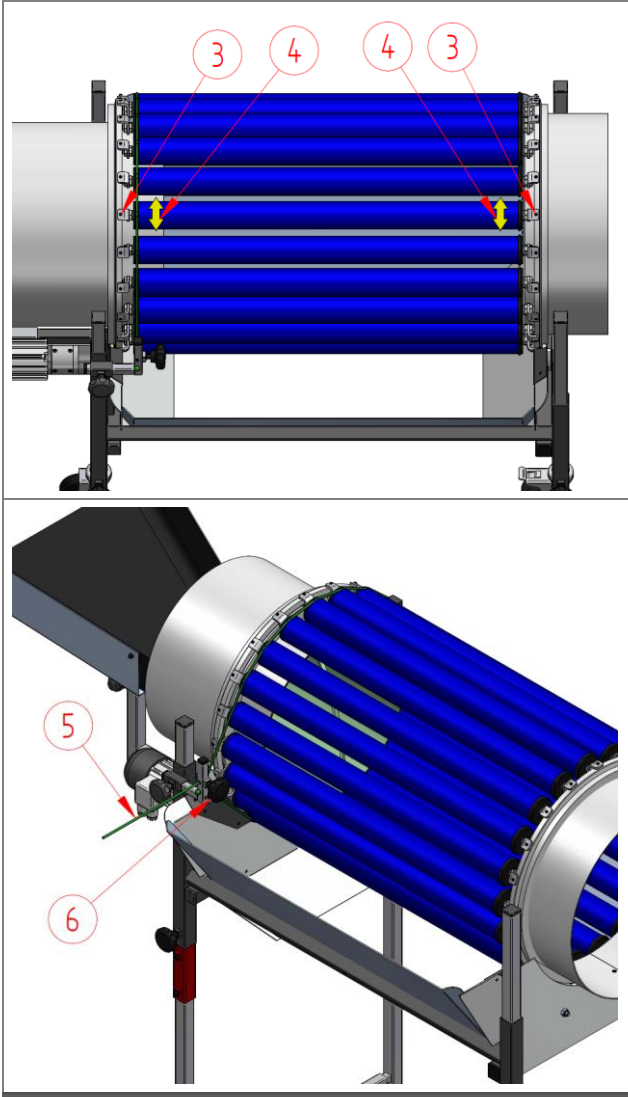
Şekil 10: Ayırıştırma boşluğunu ayarlama (tek başına ayarlama)
