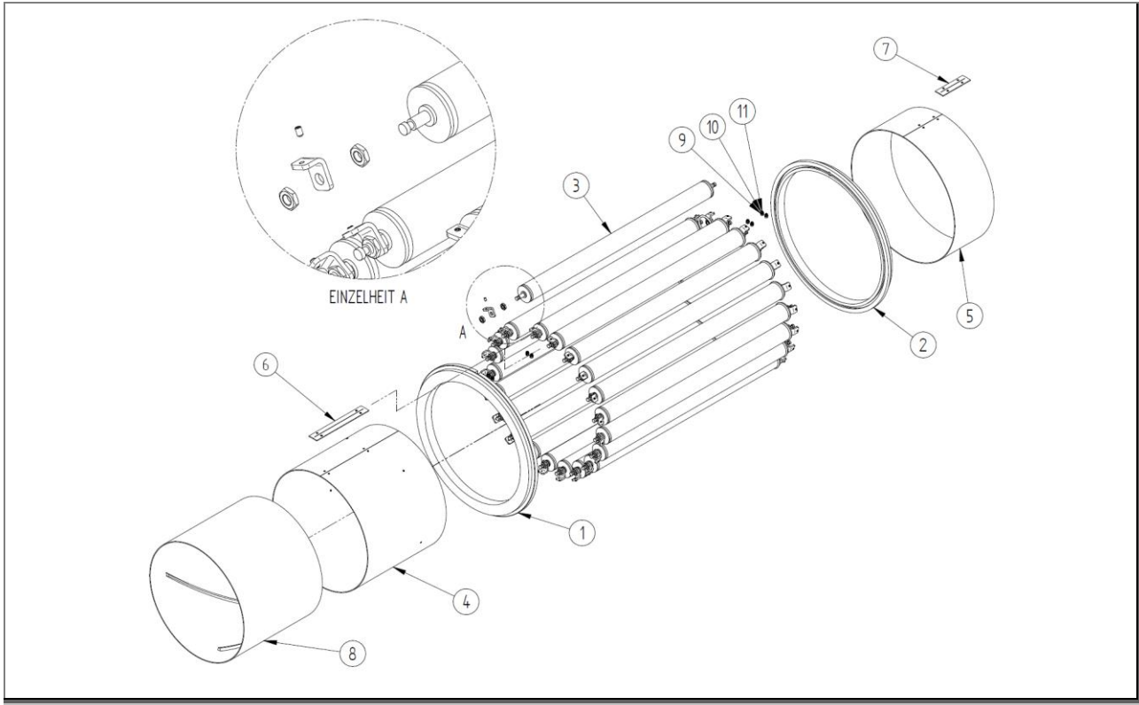
Şekil 21: Parça listesi: 30XX B tambur kafesi – U.866.0001
