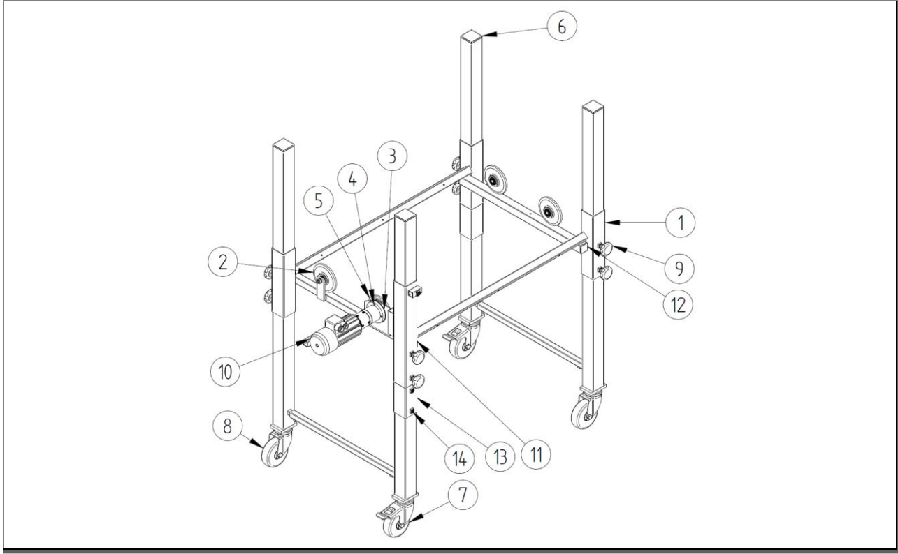
Şekil 23: Parça listesi: Alt şasi – takviyeli – ZZ.860.0021
