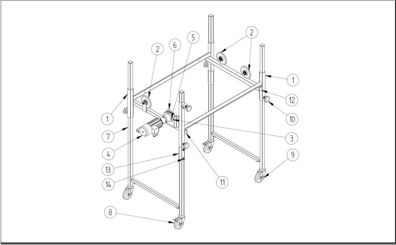
Şekil 22: Parça listesi: Alt şasi – ayırma tamburu – ZZ.860.0003
