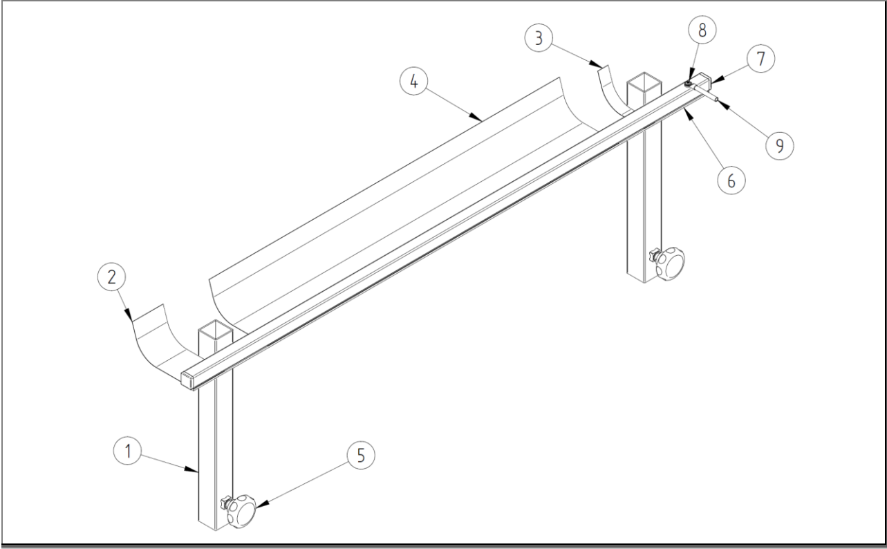
Şekil 26: Aksesuar parça listesi: Antistatik tertibat - ZZ.867.0003
