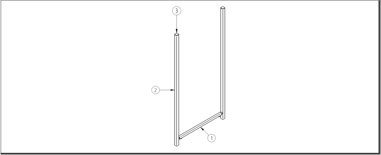
Şekil 19: Parça listesi: Tekli ayak – U.860.0005
