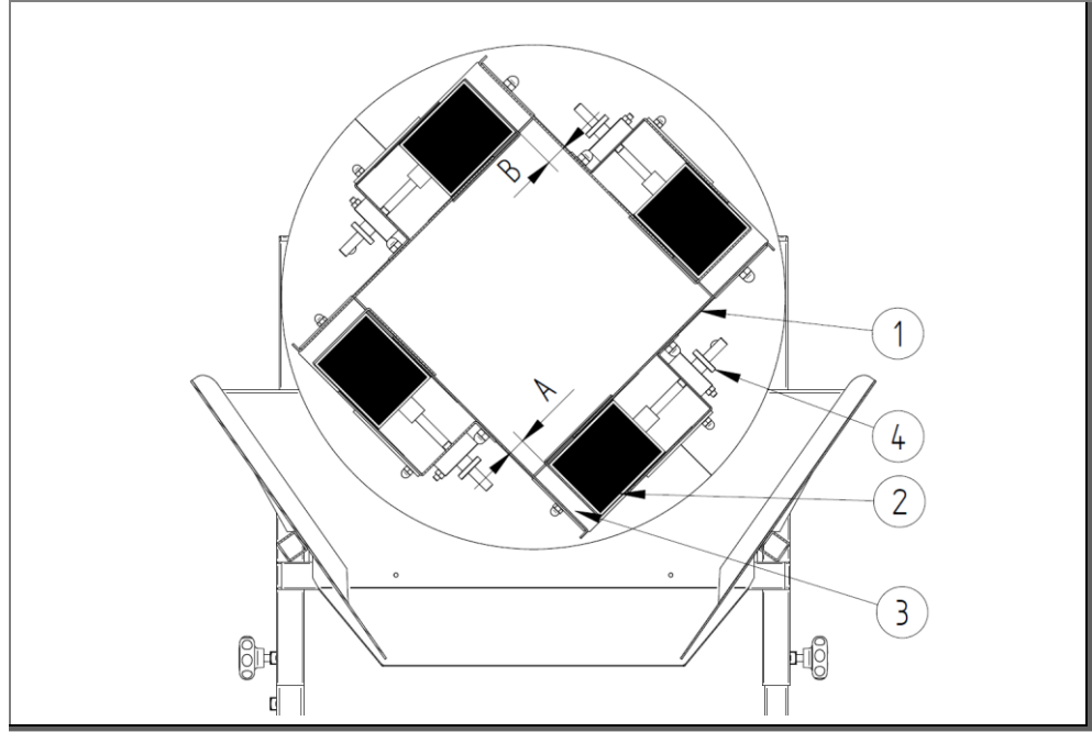
Şekil 4: Ayırma tamburunun farklı konumlardaki düşme kanalları
