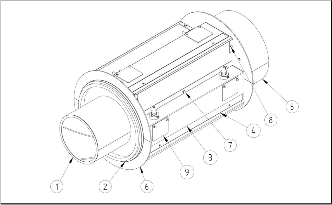
Şekil 18: Parça listesi: KR tambur kafesi – U.867.0062 / U.867.0084
