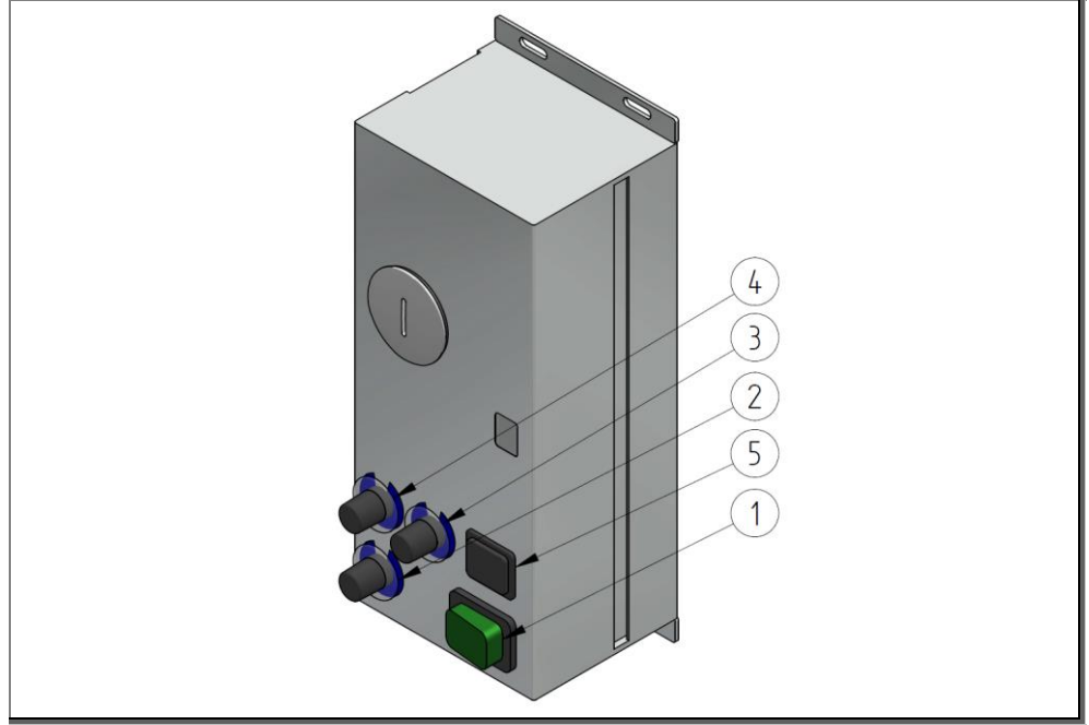
Şekil 15: "Kademesiz ayarlanabilir terse döndürülebilir" işletim türü kumanda elemanları
