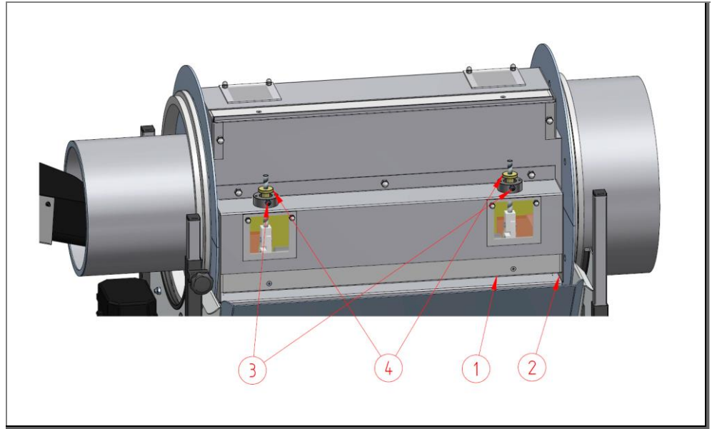
Şekil 9: Ayırıştırma boşluğunun ayarlanması
