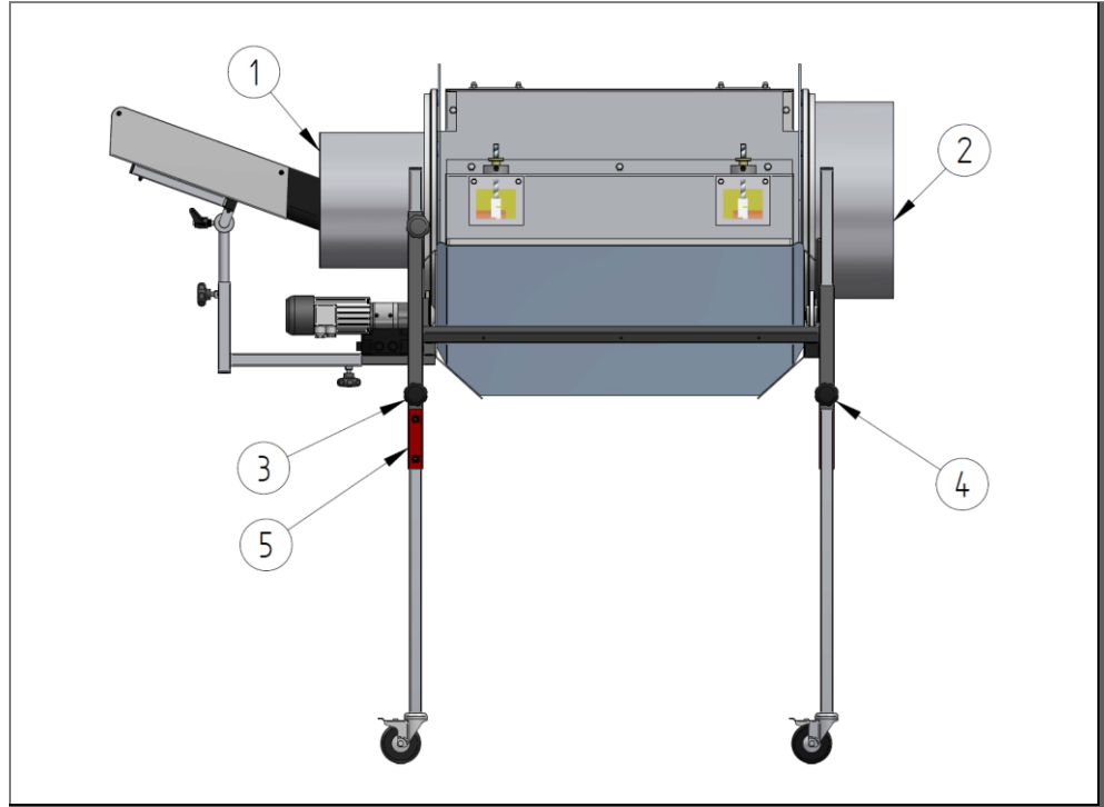
Şekil 10: Yüksekliğin ve eğimin ayarlanması
