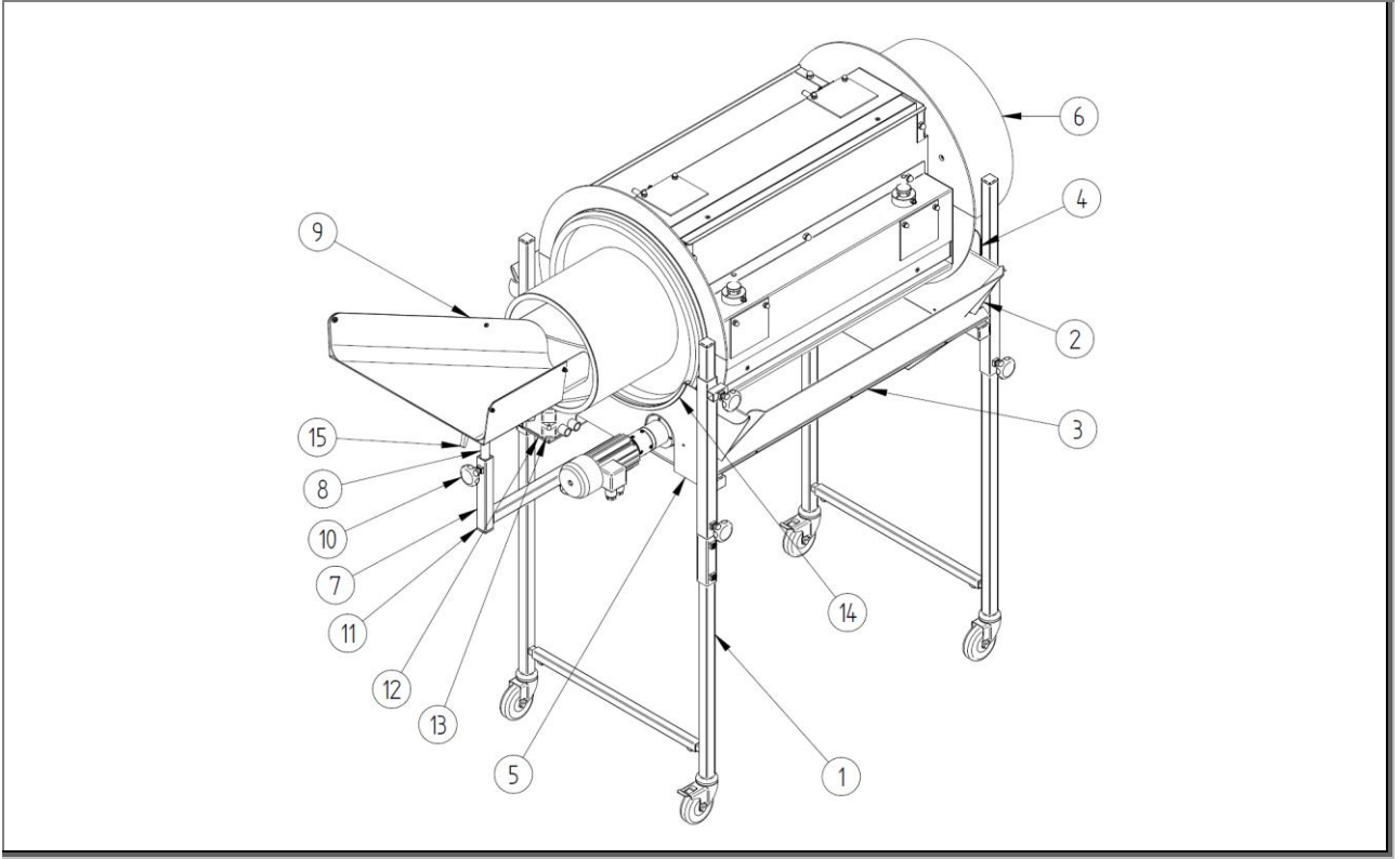
Şekil 17: Parça listesi: R dikdörtgen ayırma tamburu – ZZ.861.0065
