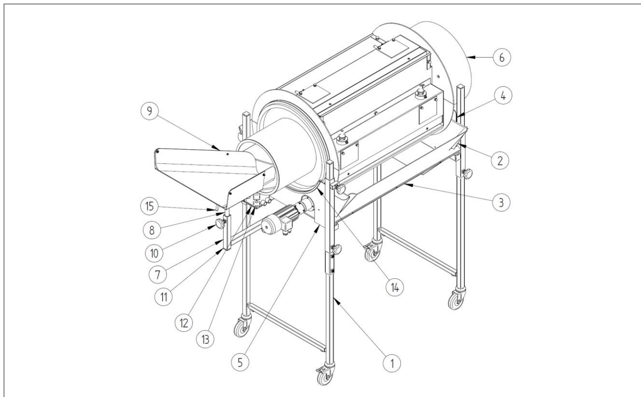
Fig. 17 : Nomenclature : tambour à séparer rectangulaire R – ZZ.861.0065
