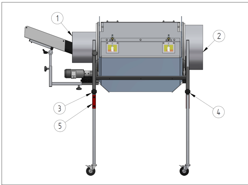
Fig. 10 : Réglage des hauteurs et de l'inclinaison
