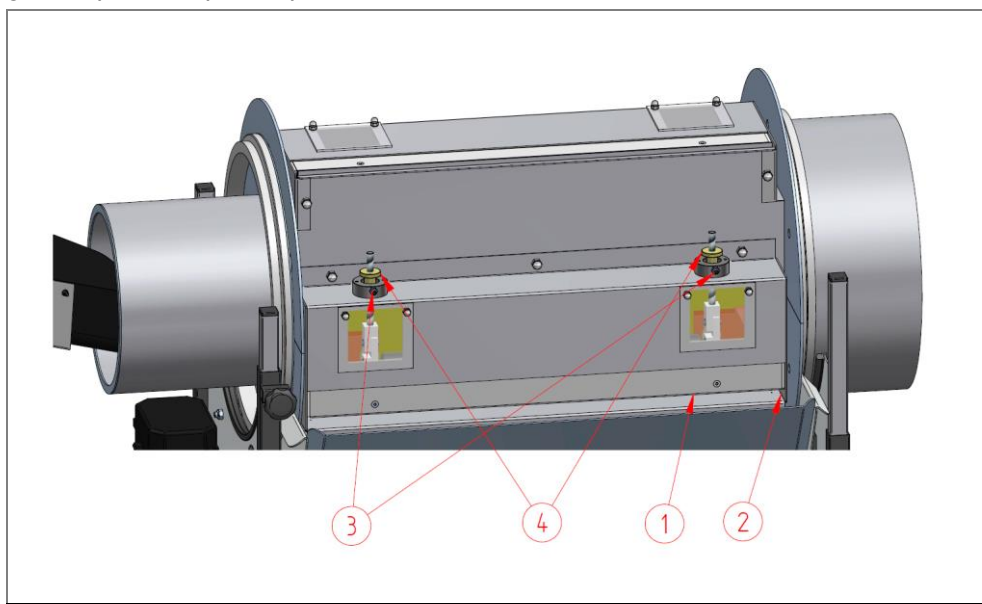
Fig. 9 : Réglage de la fente de séparation
