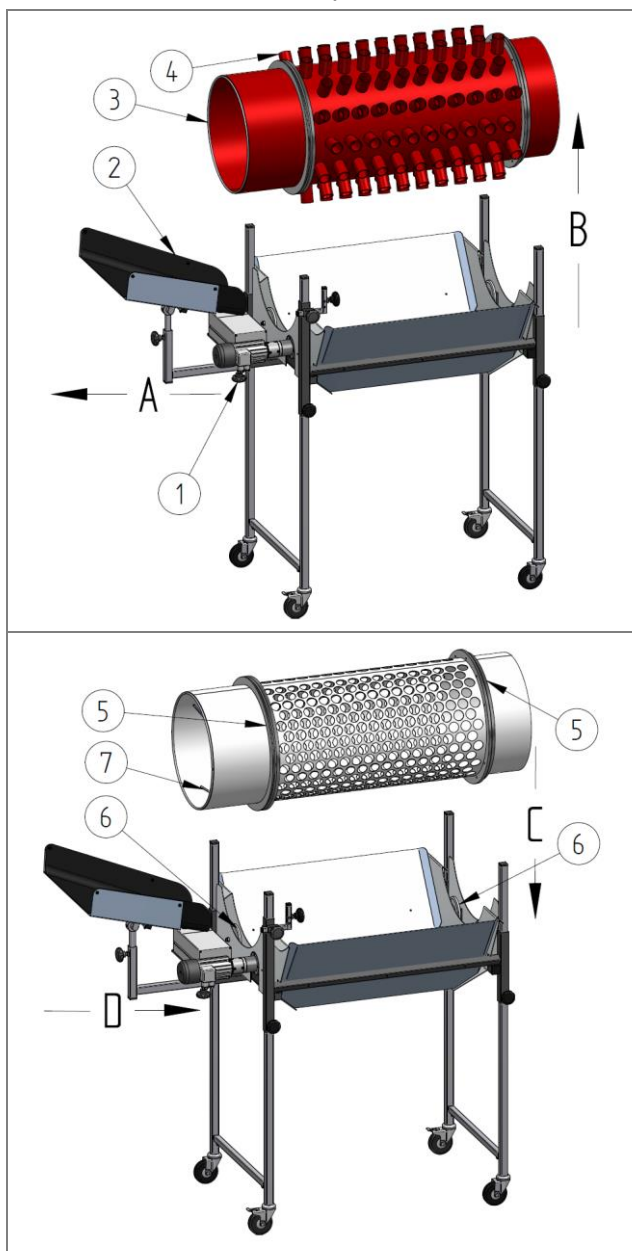
Fig. 12 : Remplacement de la cage de tambour, à l'exemple d'une cage de tambour perforé et de tambour type « hérisson » sur l'image
