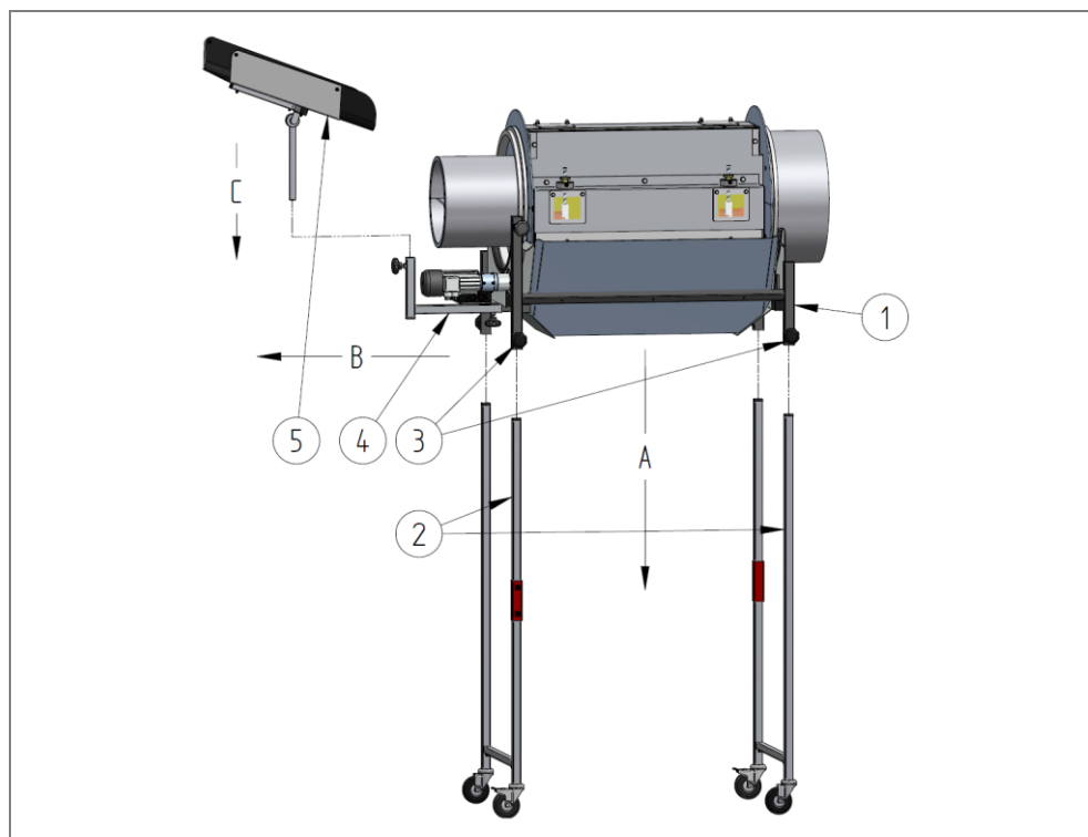
Fig. 8 : Assemblage
