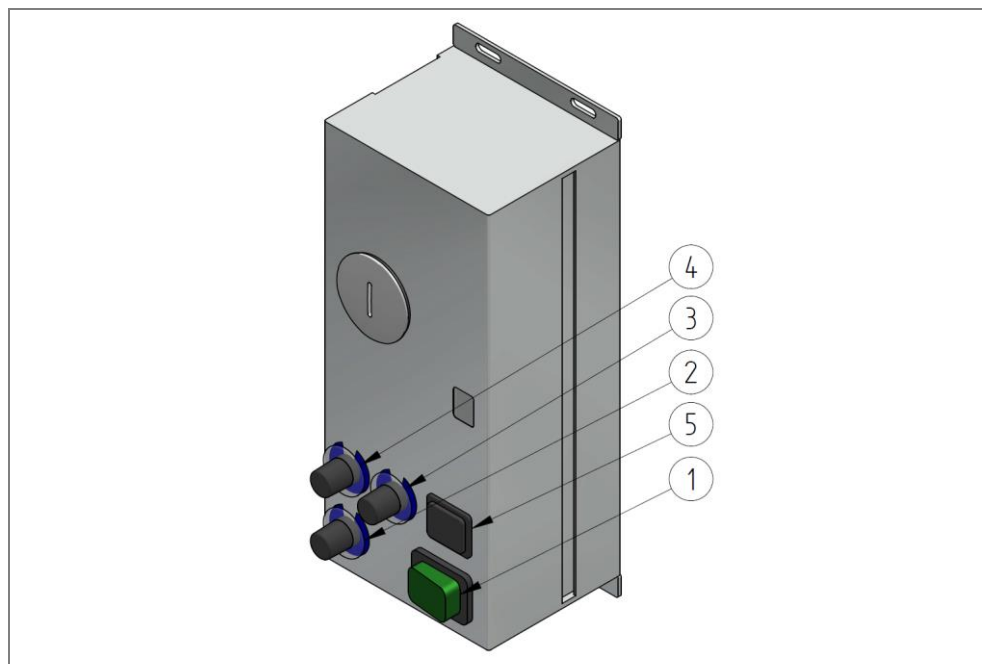
Fig. 15 : Éléments de commande pour le mode opératoire « régulation sans paliers et sens de rotation réversible »
