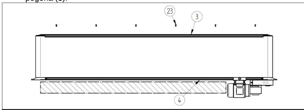
Slika 71: Razstavitev: Vodilni profil
