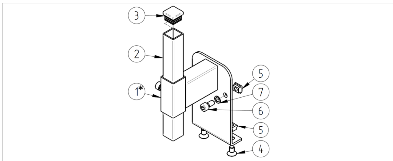
Slika 117: Kosovnica za ogrodja EM
