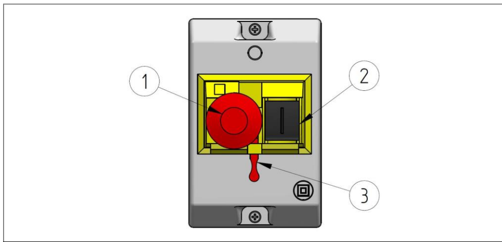
Slika 58: Glavno stikalo
