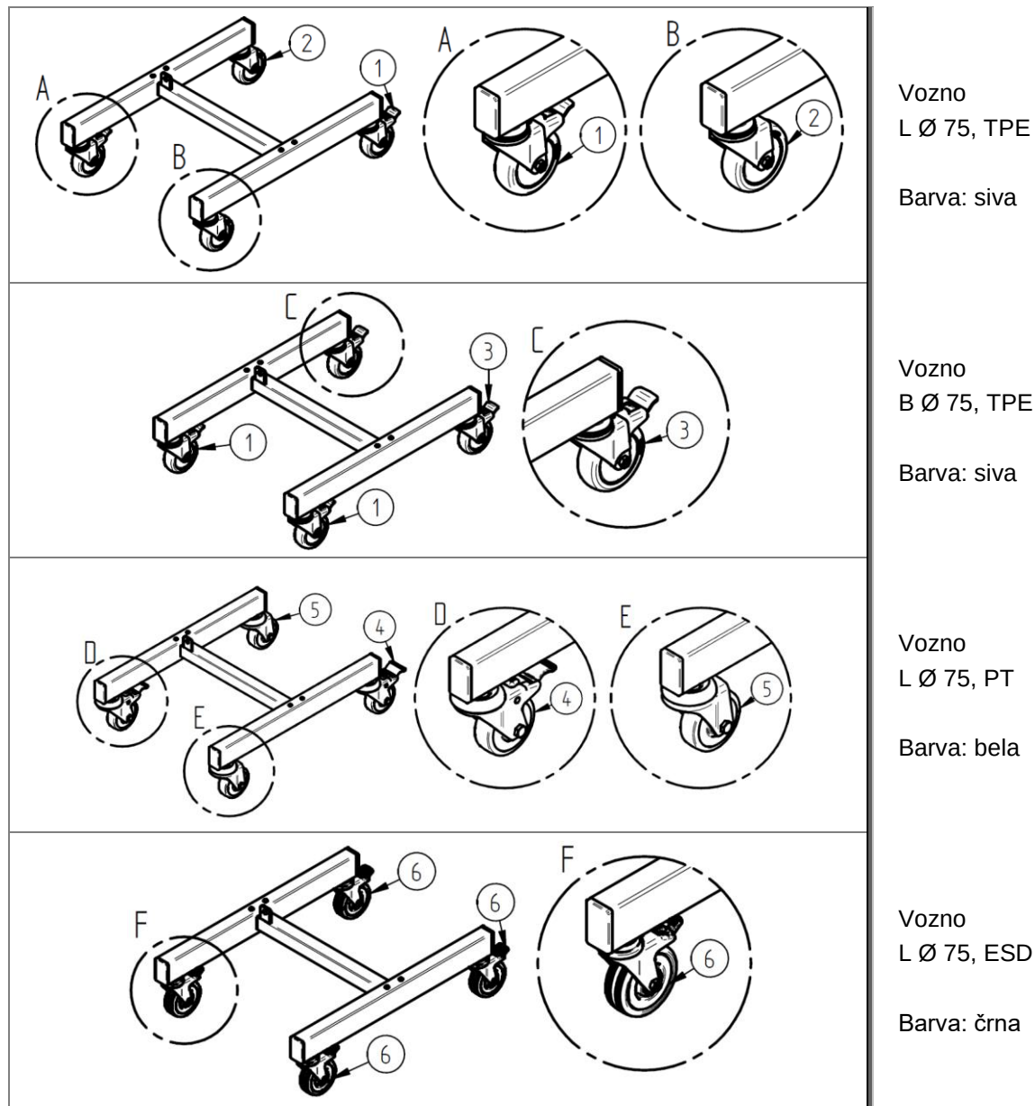
Slika 131: Kosovnica: Različice postavitve ogrodja HE/HM, kolesa s pritrdilno luknjo ZZ.982.0068.01
