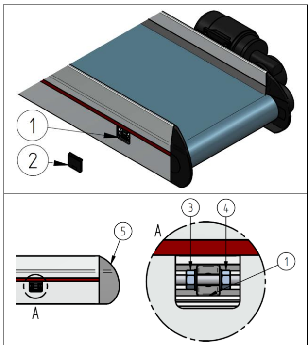
Slika 63: Priprave za nastavitve poravnosti traku (območje pogona)
