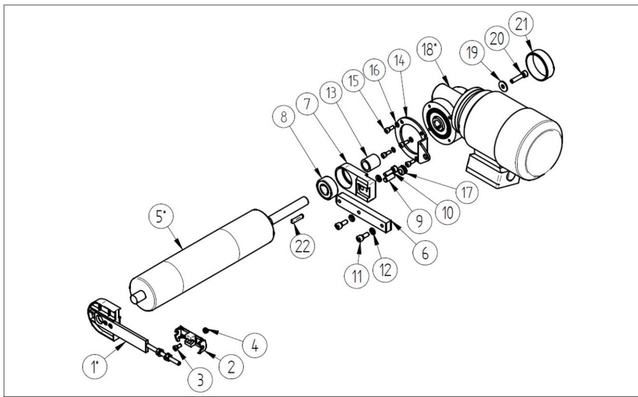
Slika 103: Kosovnica: Pogon s prirobnico – pogonska enota/motorna enota – položaj pogona 23 – ZZ.900.0034.00
