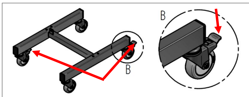
Slika 56: Blokiranje koles
