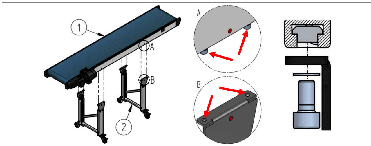
Slika 33: Namestitev transportnega traku z ogrodjem AM 010 (primer)
