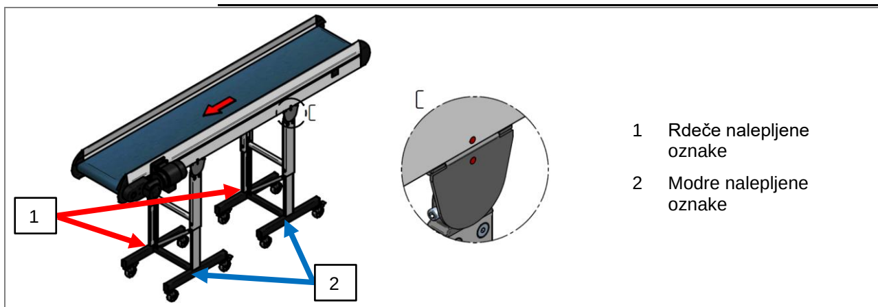
Slika 46: Celotna postavitvev transporterja z ogrodjem HE 010 – HM 010 (primer)
