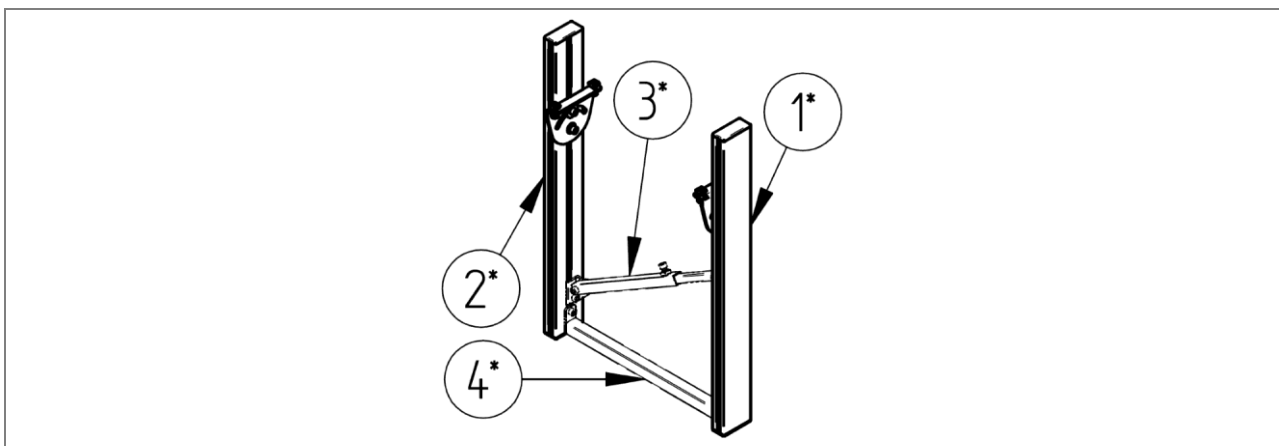
Slika 125: Kosovnica: Podpora transportnega traku AM 260 ZZ.982.0106.00
