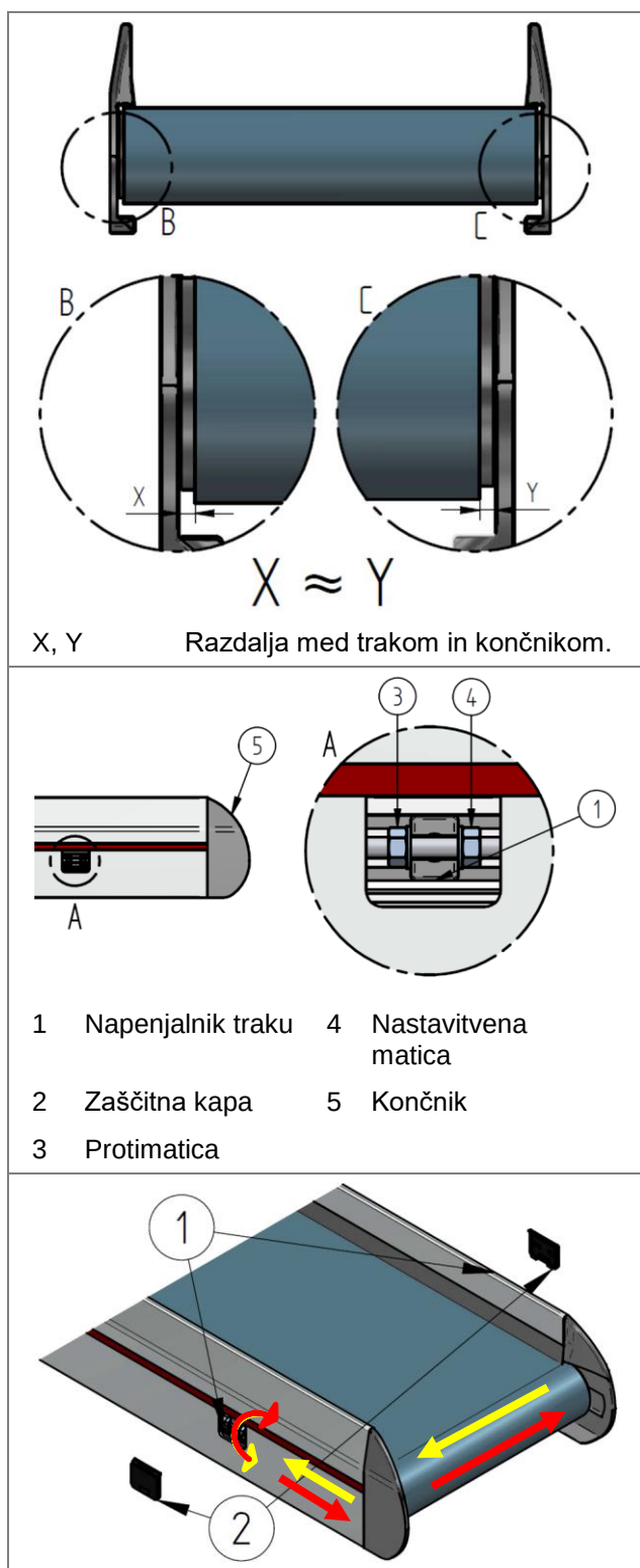
Slika 66: Nastavljanje poravnane traku v območju obračanja
