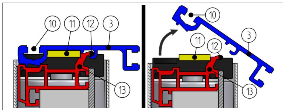
Slika 72: Odstranitev vodilnega profila
