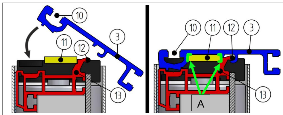
Slika 74: Namestitev vodilnega profila
