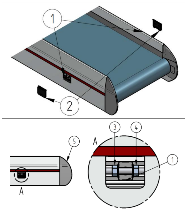
Slika 65: Priprave za nastavev poravnivosti traku (območje obračanja)
