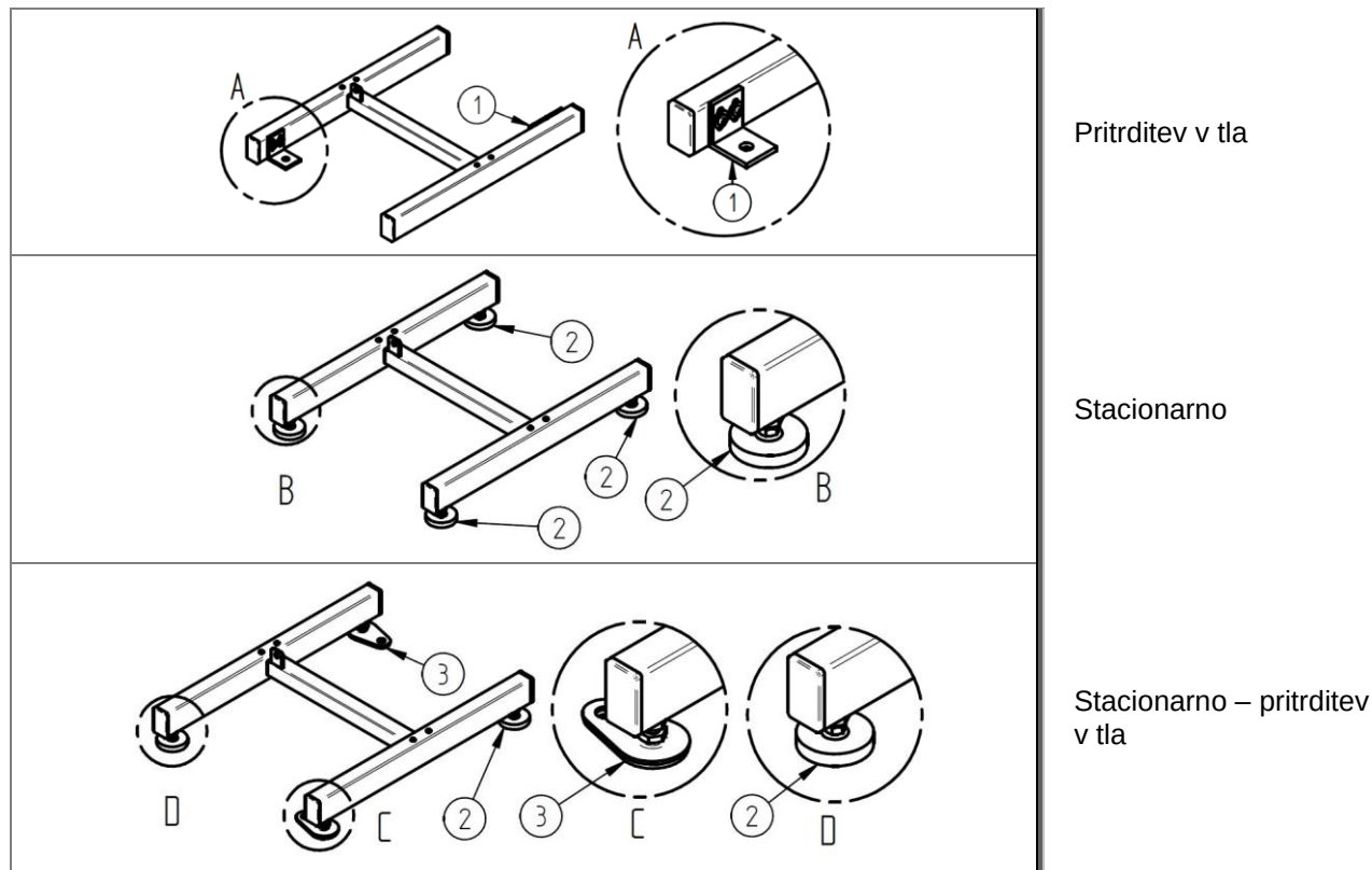
Slika 130: Kosovnica: Ogradje, različice postavitve HE/HM ZZ.982.0068.01
