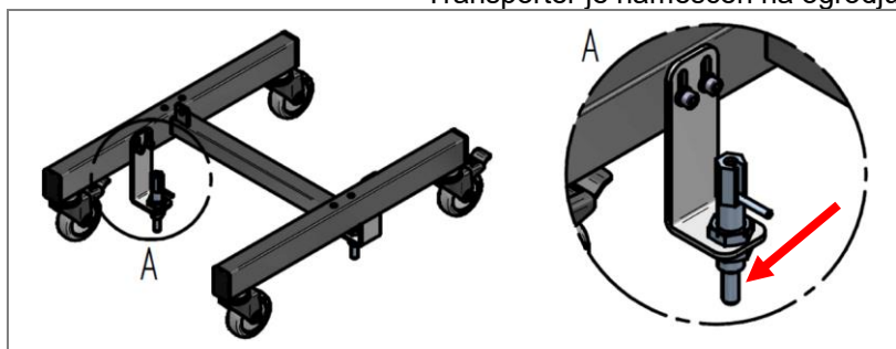
Slika 55: Talna zapora
