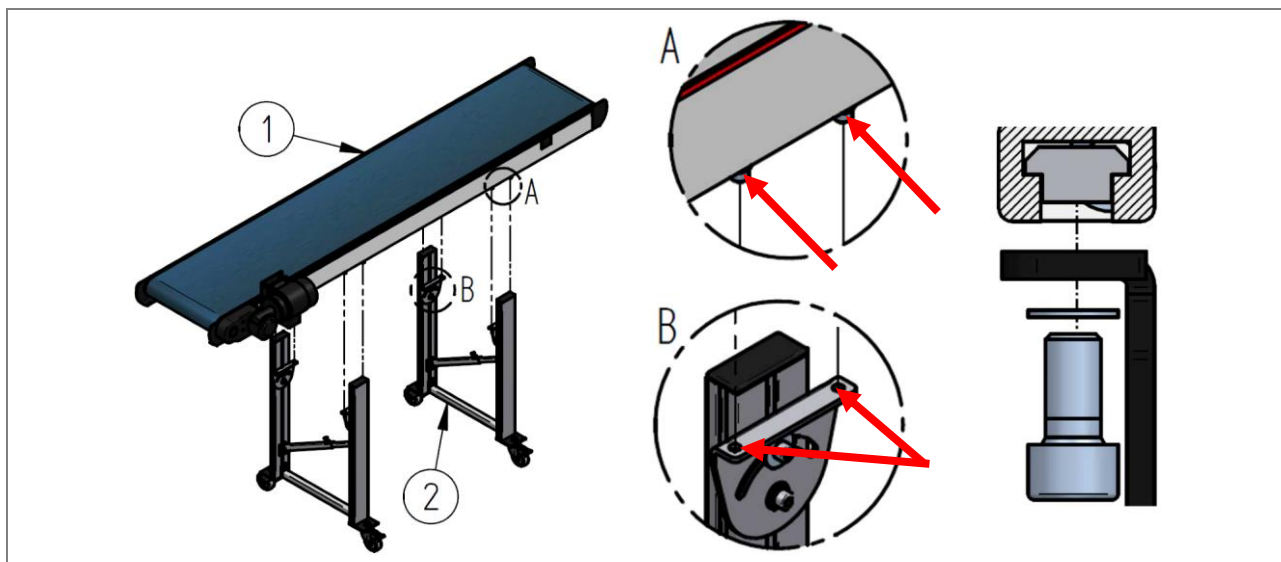
Slika 41: Namestitev transportnega traku z ogrodjem HE 030/HE 260 (primer)
