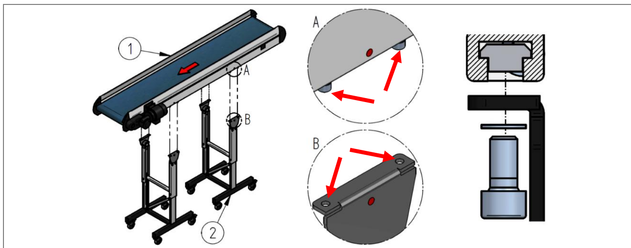
Slika 45: Namestitev transporterja z ogrodjem HE 010 – HM 010 (primer)
