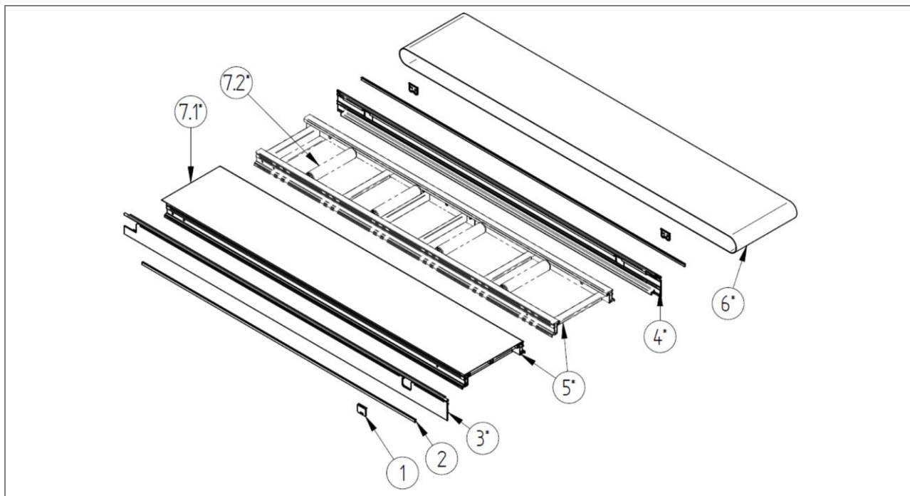
Slika 80: Kosovnica: Trup transporterja GL0 in GL7 – U.116.0002.00
