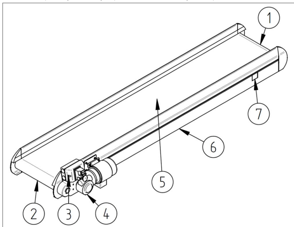
Slika 2: Raven tračni transporter (primer)
