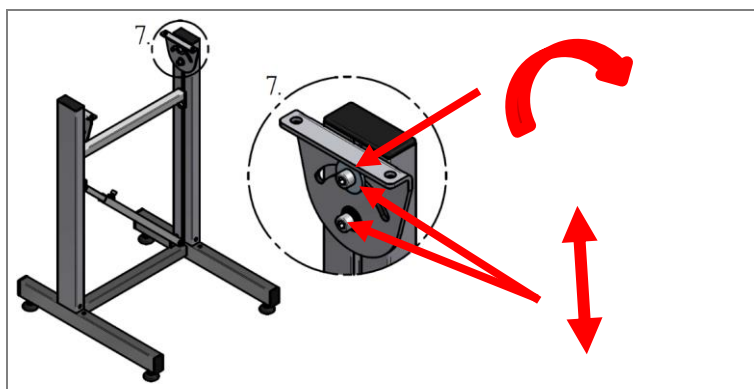
Slika 52: Namestitev ogrodja – HE 260/HM 260
