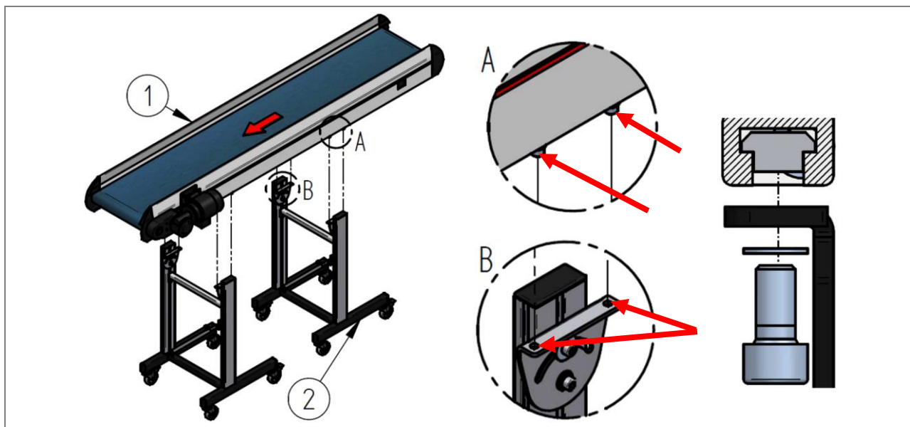
Slika 53: Namestitev transportnega traku z ogrodjem HE 030/HE 260 (primer)
