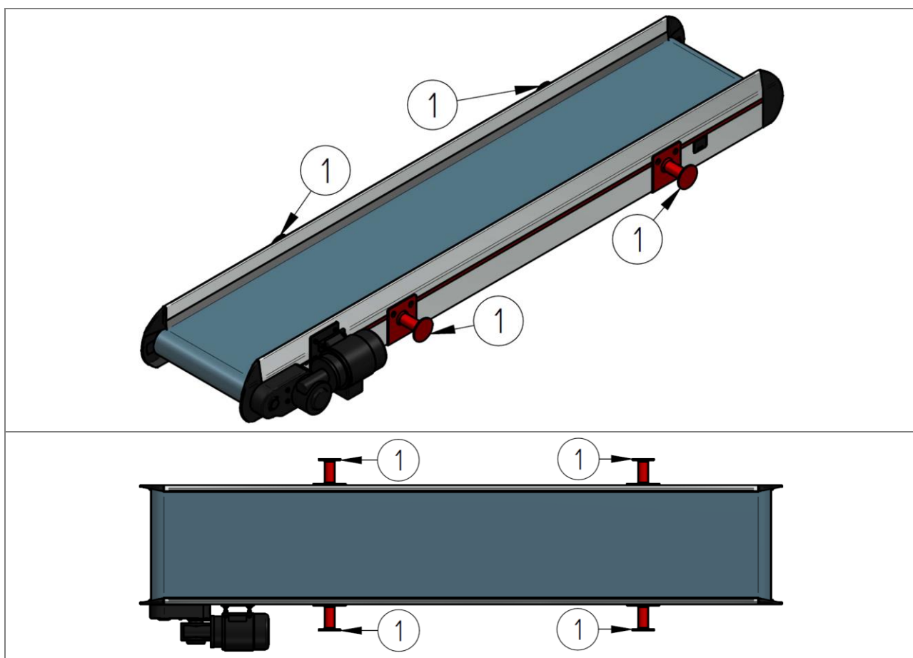
Slika 26: Točke za privez dvizne opreme (npr. vrvi)
