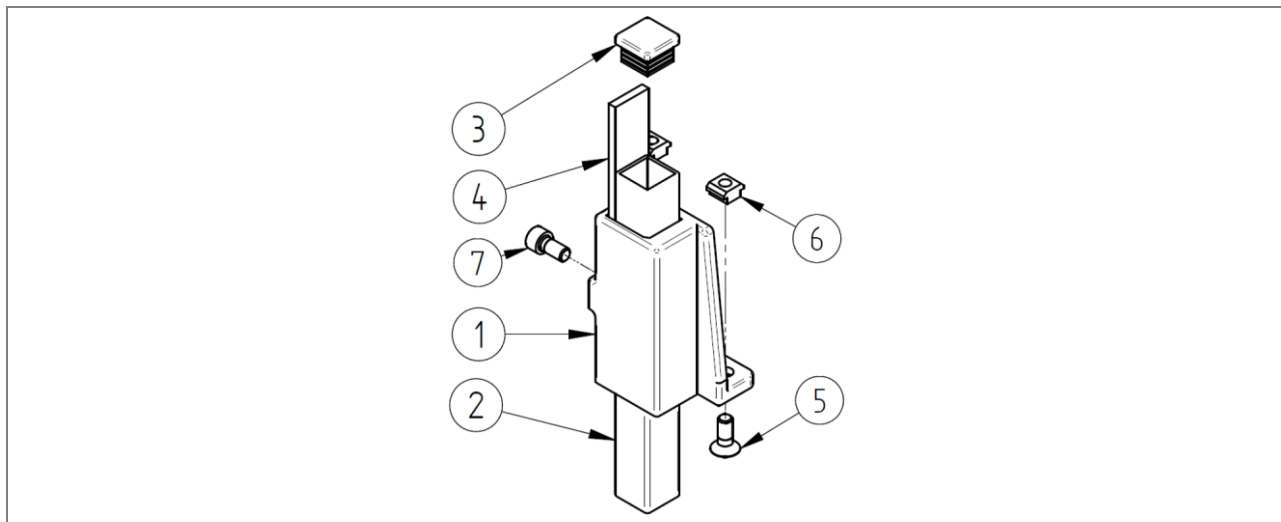
Slika 114: Kosovnica: Podpora transportnega traku IK1 U.800.0182.00
