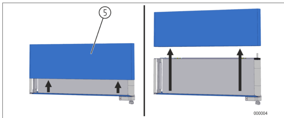
Slika 73: Snemanje traku
