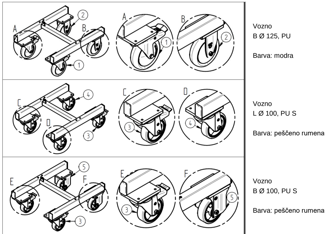
Slika 133: Kosovnica: Različice postavitve ogrodja HE/HM, kolesa s pritrdilno luknjo ZZ.982.0068.01
