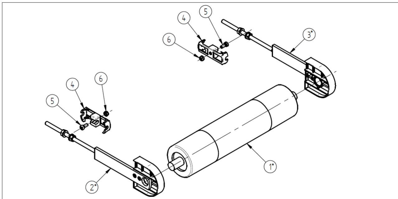
Slika 83: Kosovnica: Obračalna enota Multi-Tech Ø 80 – ZZ.800.0093.03
