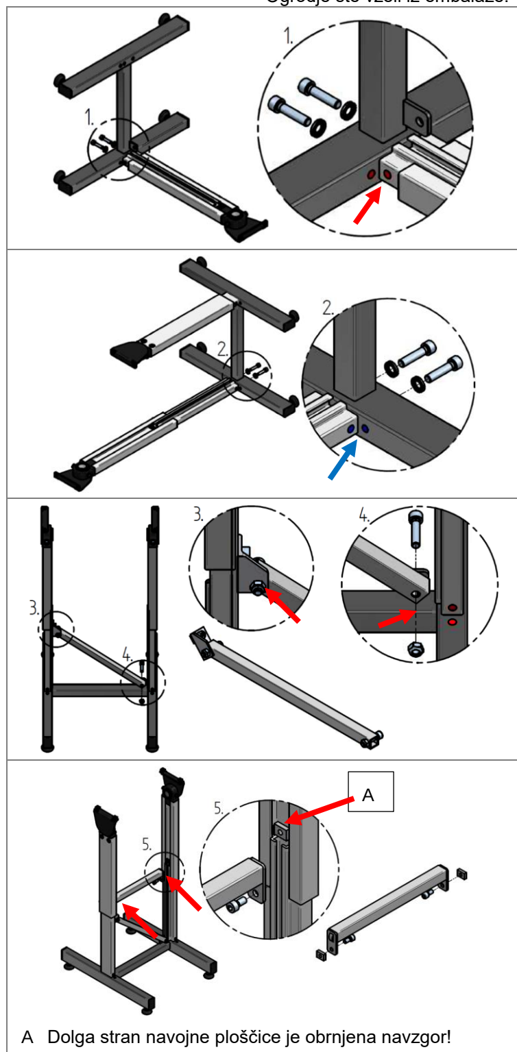
Slika 43: Namestitev ogrodja – HE 010/HM 010
