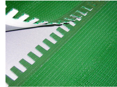
PVC-IKLUMET-Verbindung
