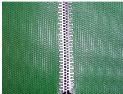
Versetzte Kleinstriemenhakenverbindung
