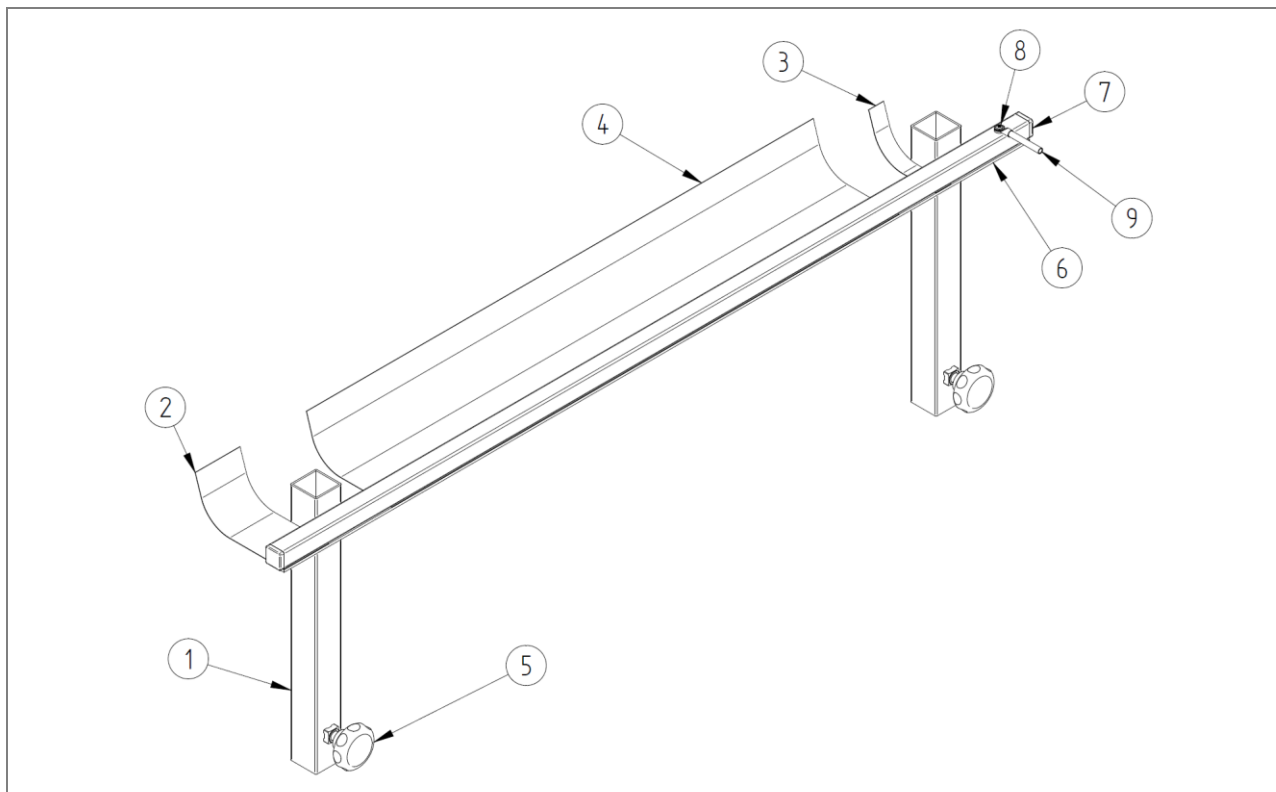
Abb. 32: Zubehör Stückliste: Antistatik-Vorrichtung - ZZ.867.0003
