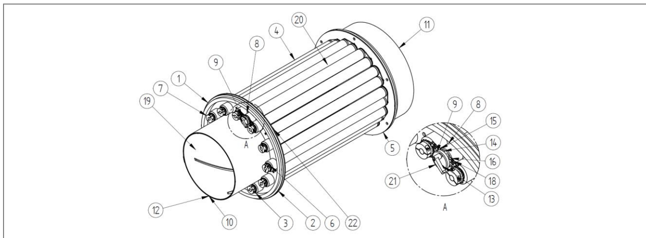
Abb. 24: Stückliste: Trommelkäfig KPZ 35XX B – U.865.0001
