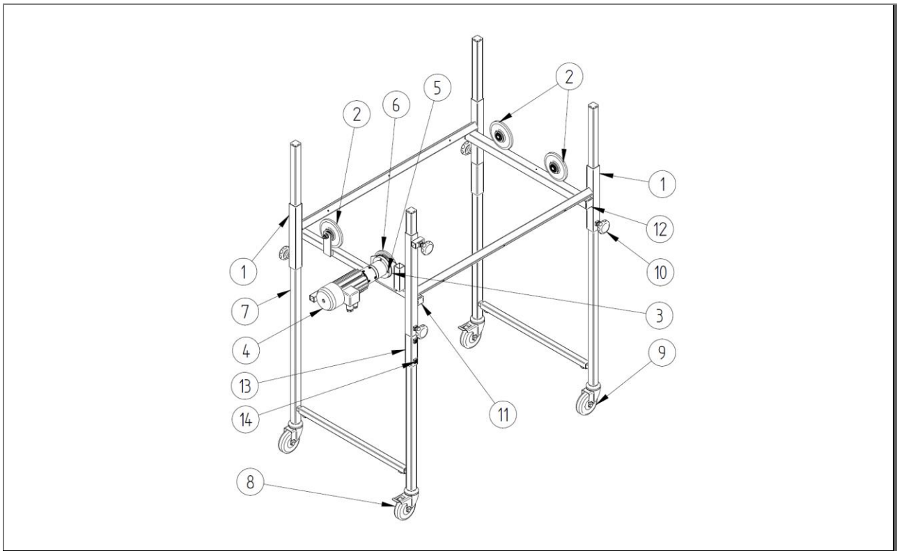
Abb. 26: Stückliste: Untergestell – Separiertrommel – ZZ.860.0003
