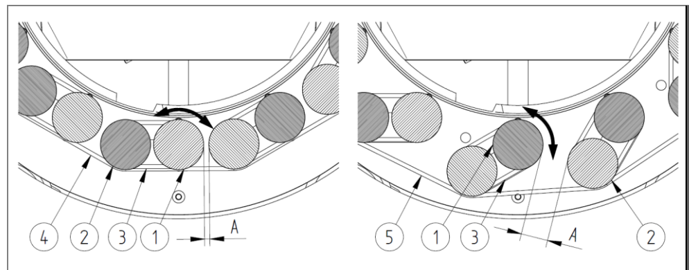
Abb. 4: Rollenpaare der Separiertrommel in verschiedenen Stellungen
