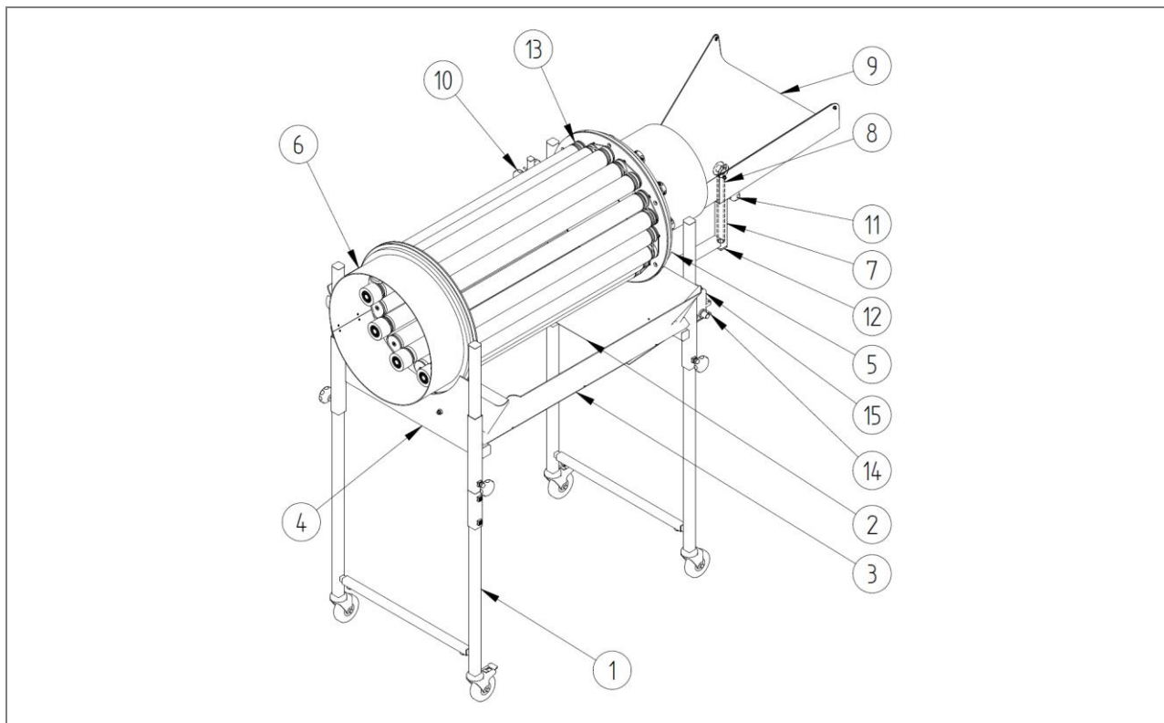
Abb. 19: Stückliste: Separiertrommel PZ 25XX B – ZZ.865.0002
