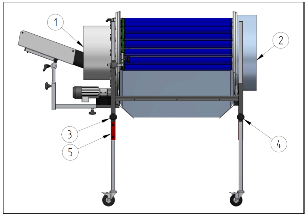
Abb. 11: Einstellen der Höhen und Neigung
