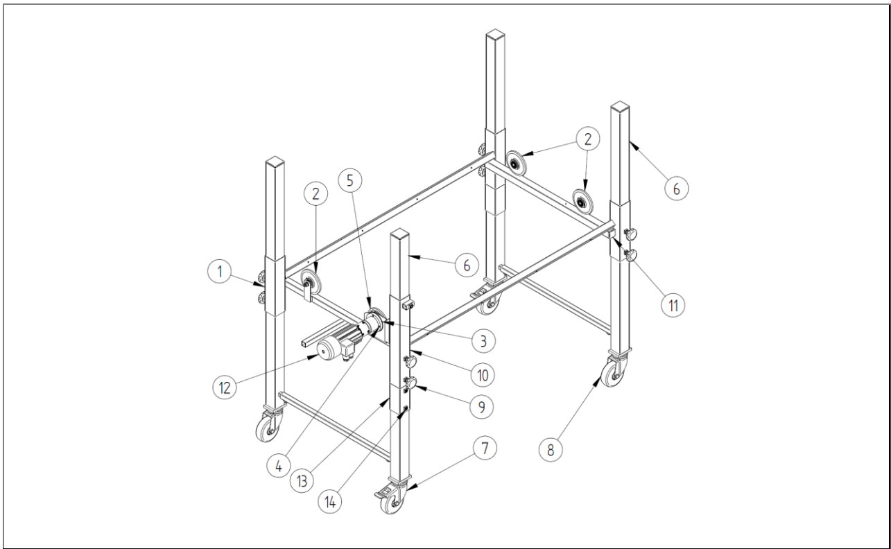
Abb. 28: Stückliste: Untergestell – verstärkt – ZZ.860.0005
