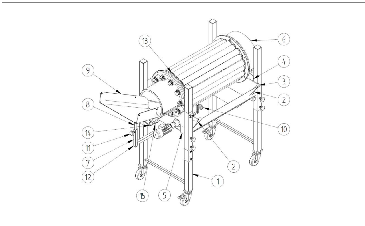
Abb. 21: Stückliste: Separiertrommel PZ 25XX B, verstärkt – ZZ.865.0067
