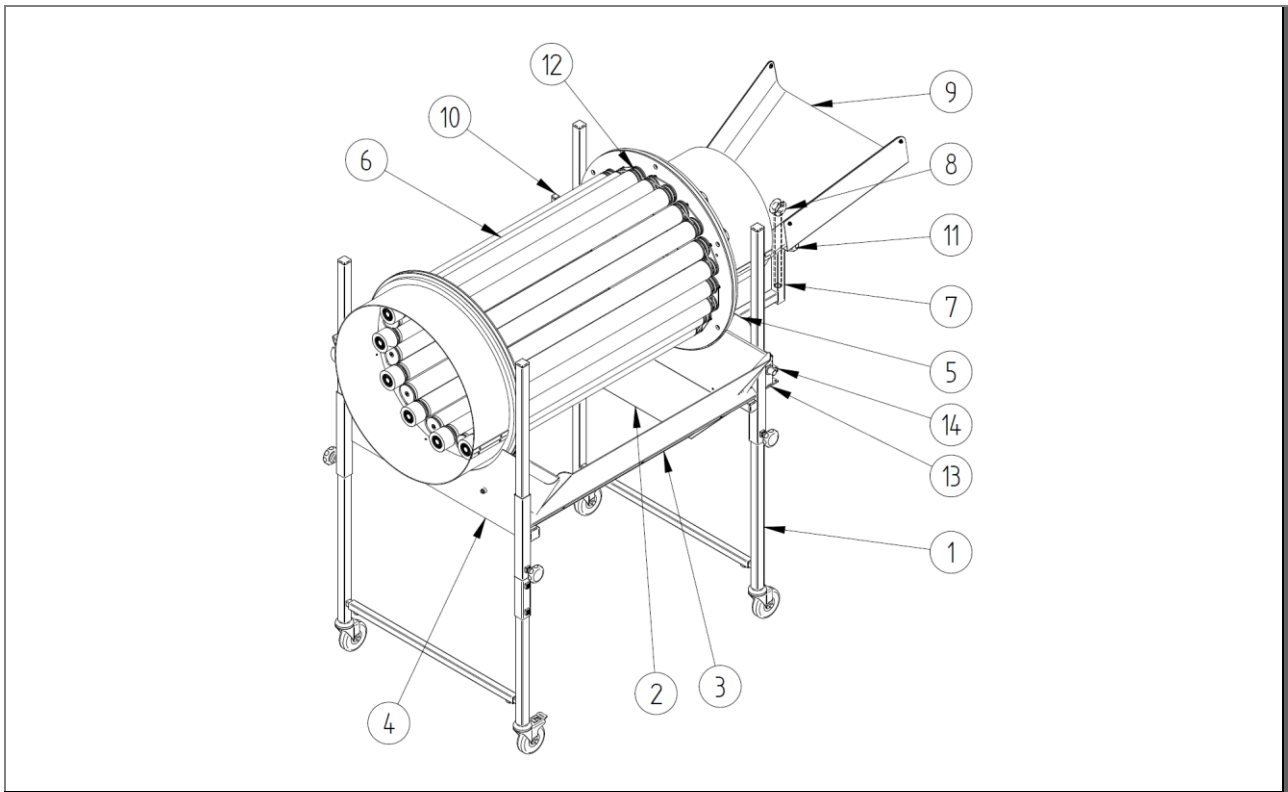
Abb. 20: Stückliste: Separiertrommel PZ 35XX B – ZZ.865.0001
