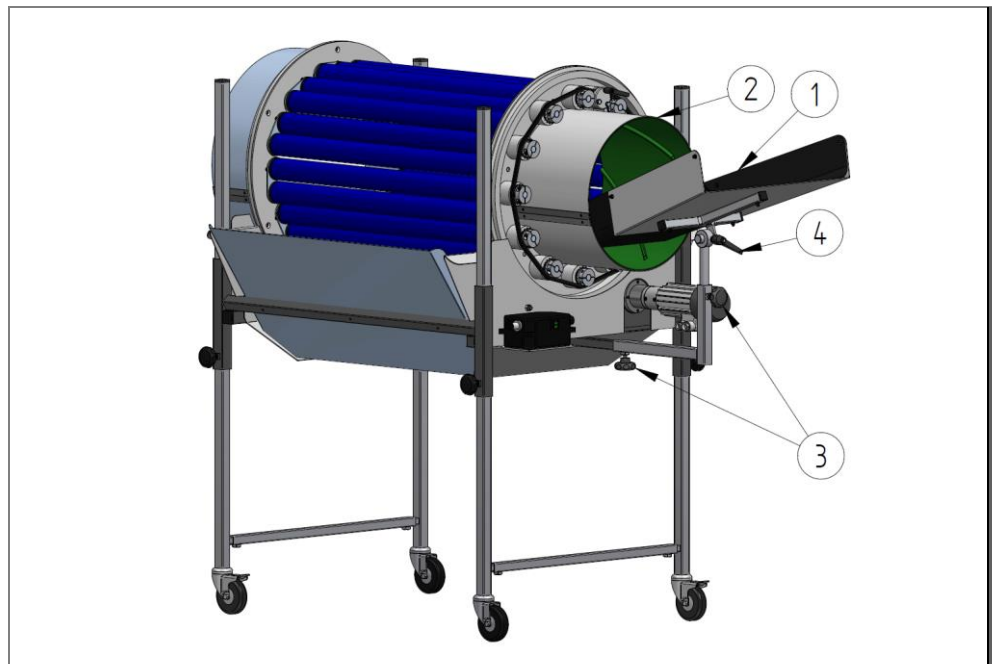
Abb. 12: Einstellmöglichkeiten der Einlaufrutsche
