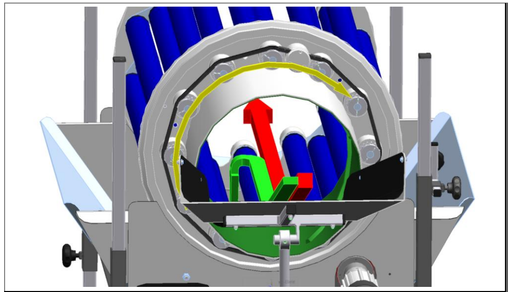
Abb. 2: Funktionsprinzip und Teiledurchlaufrichtung
