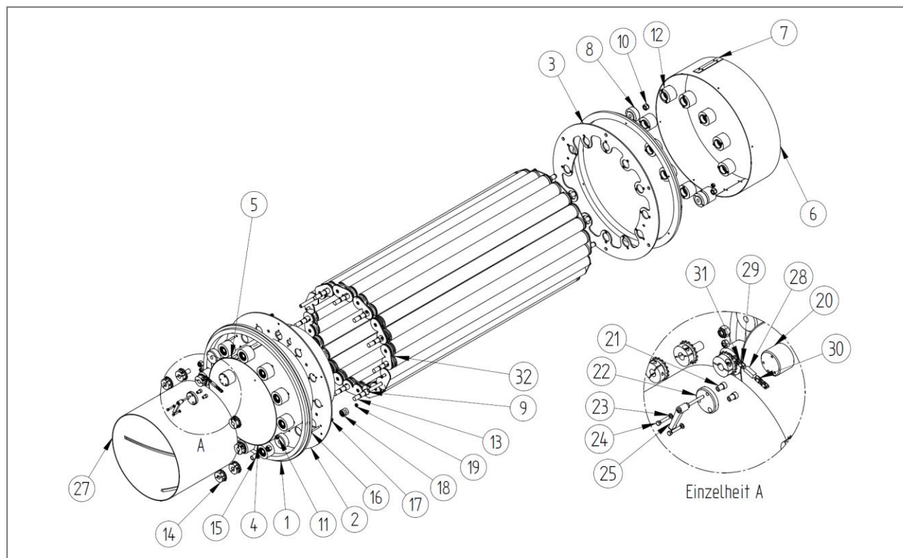
Abb. 25: Stückliste: Trommelkäfig KPZ 35XX B, verstärkt – U.865.0006
