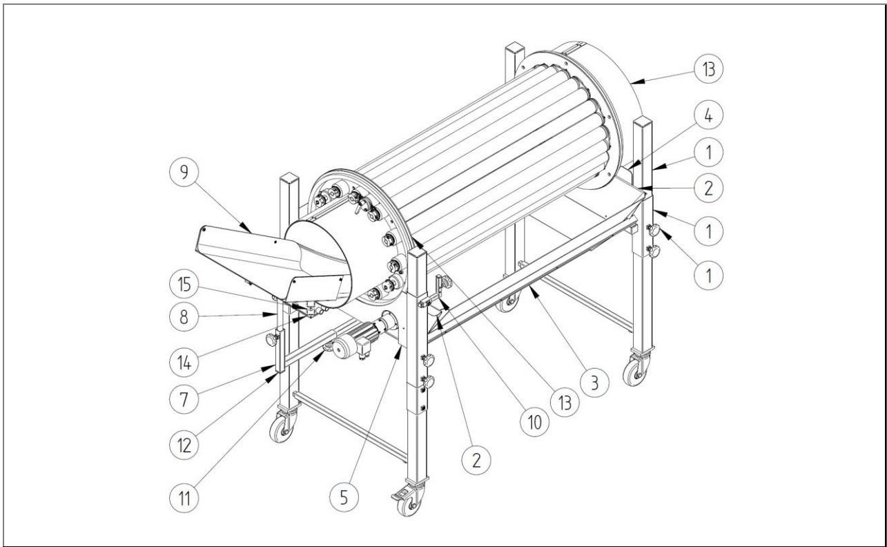
Abb. 22: Stückliste: Separiertrommel PZ 35XX B, verstärkt – ZZ.865.0008
