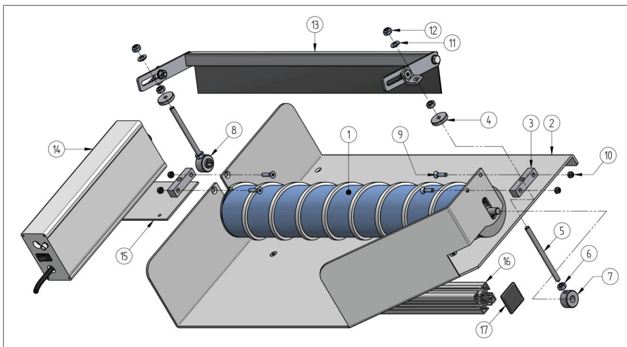
Abb. 13: Explosionsdarstellung Schneckenseparierer
