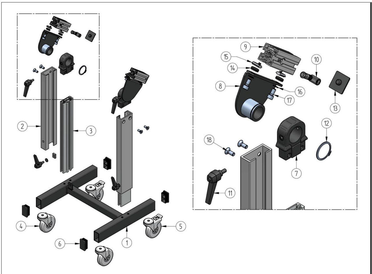
Abb. 16: Untergestell MSL/MSR
