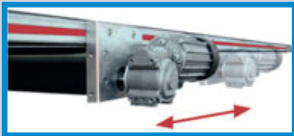
Commande d'entraînement central avec moteur installé au-dessous du corps de la bande
