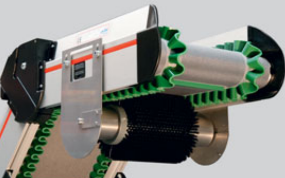
Brosse-racloir motorisée
