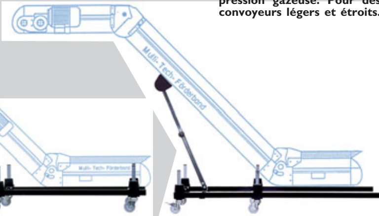
KF 010 , plateformes de support, roues réglables longitudinalement et en hauteur. Pour convoyeurs à inclinaison avec courte bande ascendante.
