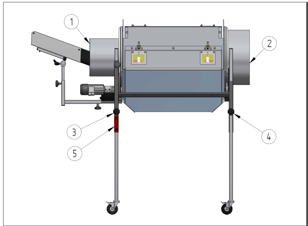
Fig. 10 : Réglage des hauteurs et de l'inclinaison
