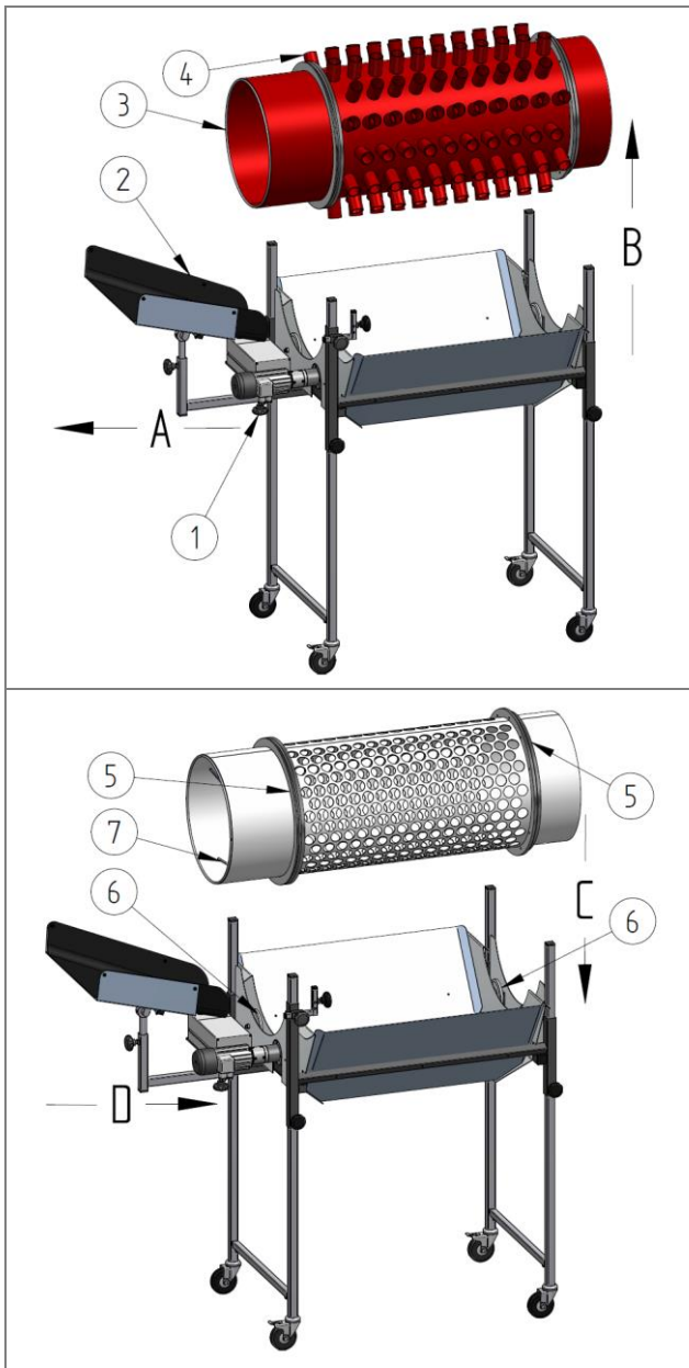
Fig. 12 : Remplacement de la cage de tambour, à l'exemple d'une cage de tambour perforé et de tambour type « hérissron » sur l'image
