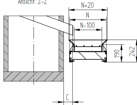
Ansicht: Z-Z
