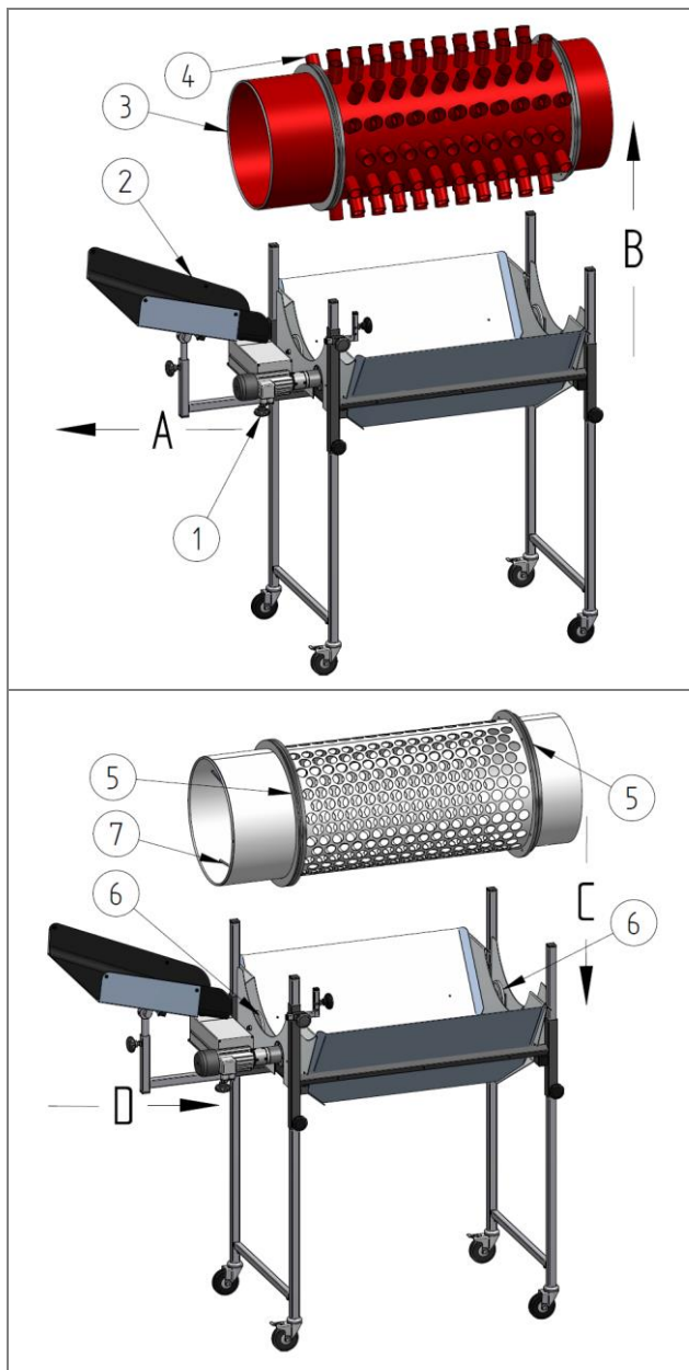
12. ábra: A dobkosár cseréje, az ábrán a perforált és a tuskés dobkosár példáján látható
