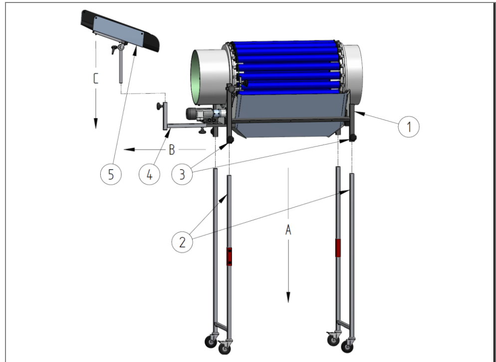
Rys. 9: Konstrukcja
