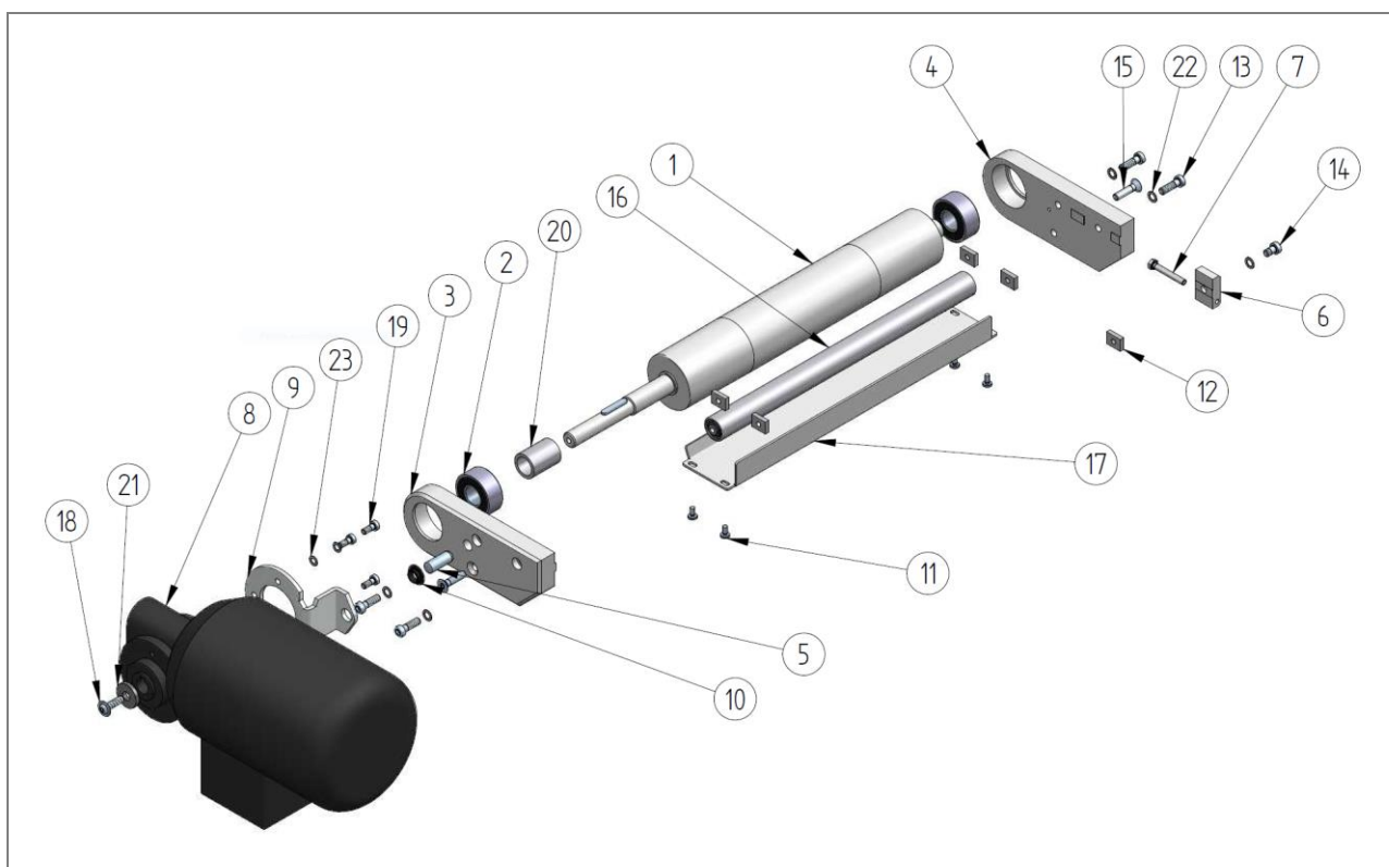
Rys. 81: Lista części: Napęd kołnierzowy – Jednostka napędowa / Jednostka silnika – Pozycja napędu 1234 – ZZ.900.0057
