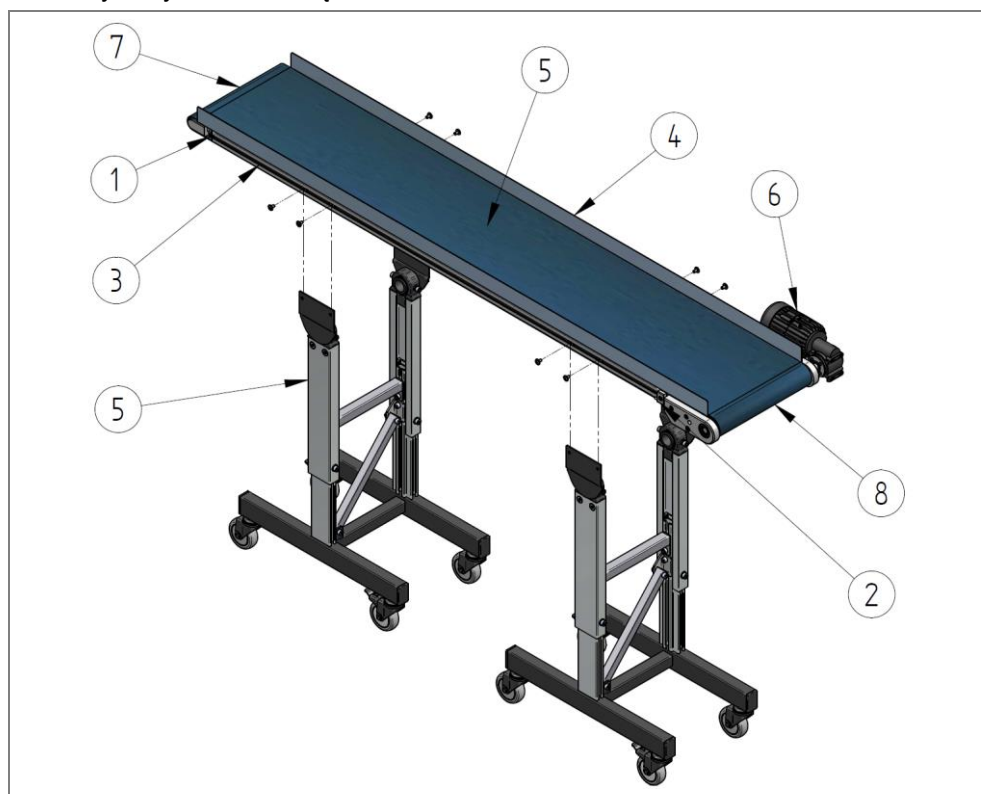
Rys. 64: Przenośnik taśmowy – nazwy elementów
