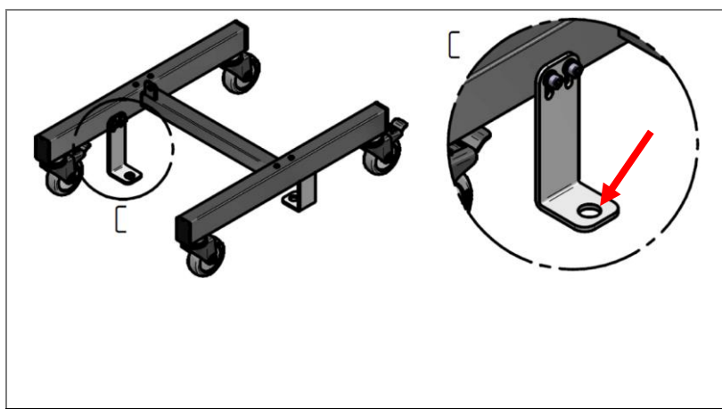
Rys. 52: Mocowanie podłogowe
