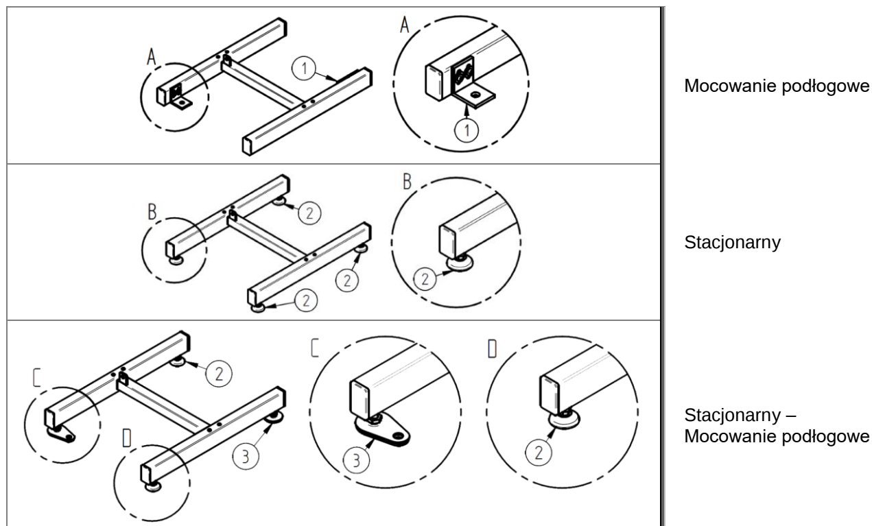
Rys. 102: Lista części: Rama podstawy, warianty ustawienia HE/HM ZZ.982.0068.01
