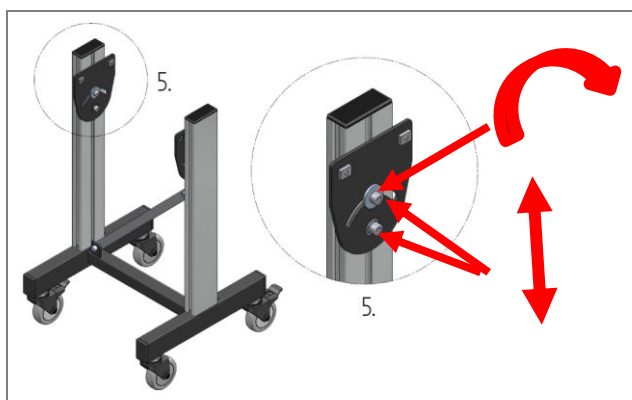
Rys. 39: Regulacja ramy podstawy – HE 060 / HM 590
