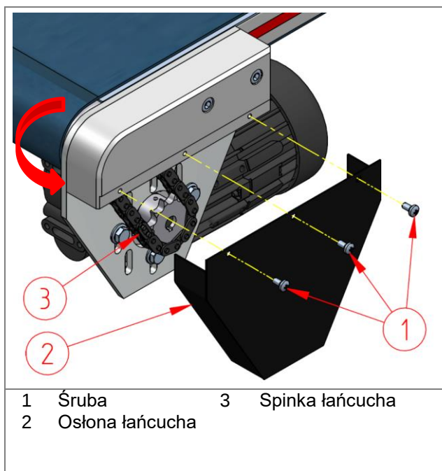
Rys. 68: Napęd łańcuchem: Sprawdzanie swobody pracy przebiegu taśmy
