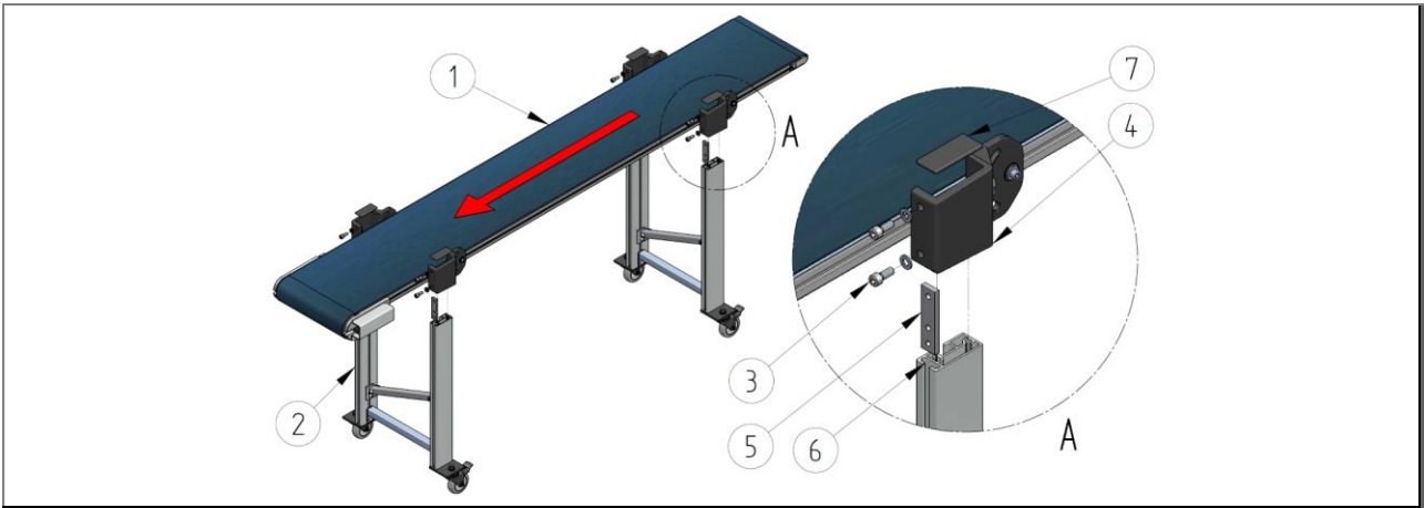
Rys. 28: Montaż przenośnika taśmowego z ramą podstawy AM 140 (przykładowy)
