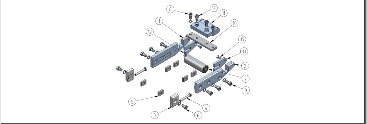
Şekil 77: Parça listesi: Yön değiştirme Ø16, Nominal genişlik 70 – U.910.0030
