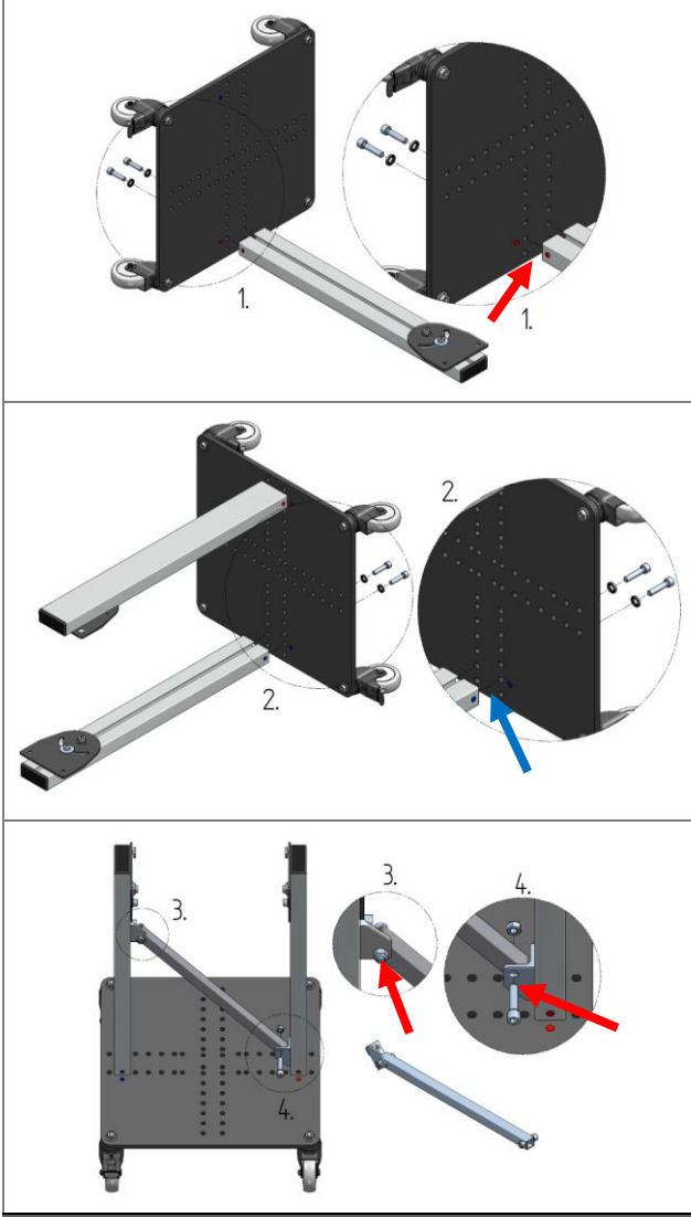
Şekil 46: BE 020 / BM 120 alt şasisinin montajı
