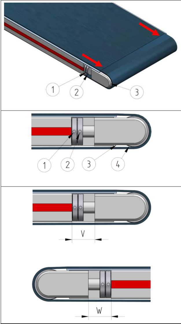
řekil 63: Yön deęiřtirme bölgesindeki bant (kayıř) gerginlięinin ayarlanması
