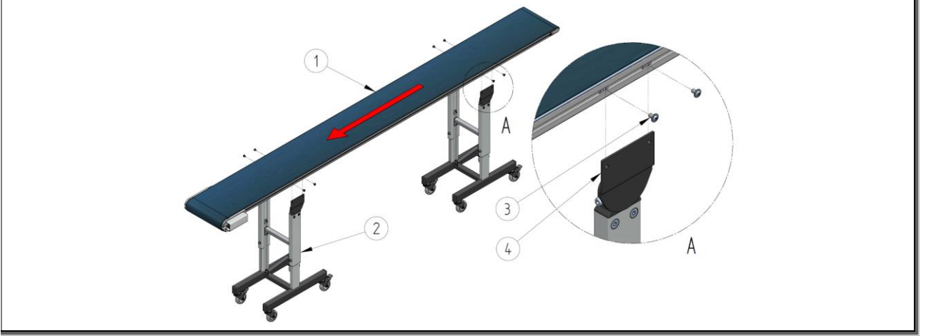
Şekil 36: HE 050 – HM 480 alt şasili konveyörün montajı (örnek)
