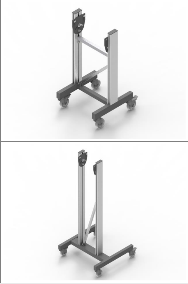
Şekil 13: Alt şasi HE 030
