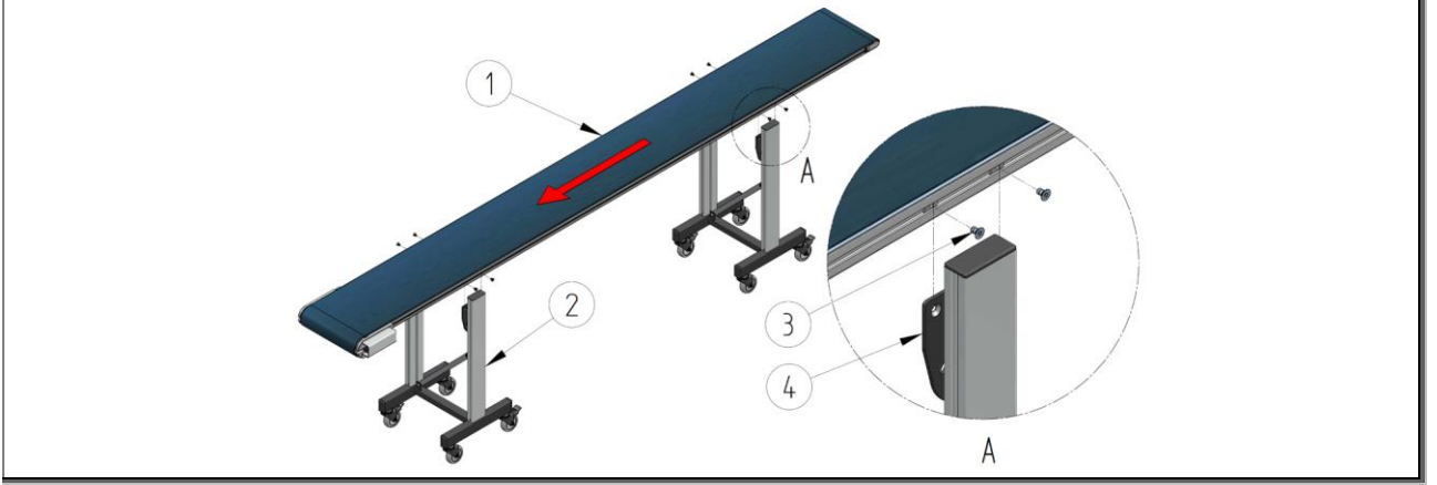
Şekil 40: HE 060 – HM 590 alt şasili konveyörün montajı (örnek)
