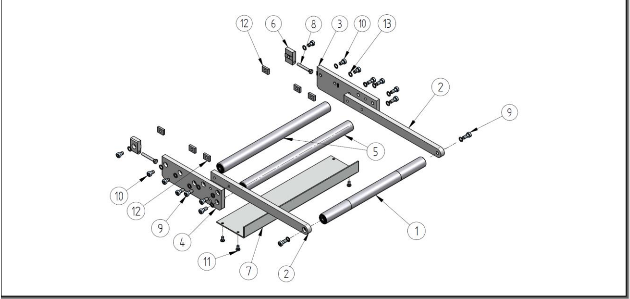
Şekil 75: Parça listesi: Yön değiştirme Ø22 – ZZ.800.0220
