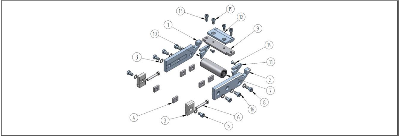
Şekil 79: Parça listesi: Yön değiştirme Ø8, Nominal genişlik 70 – U.910.0031
