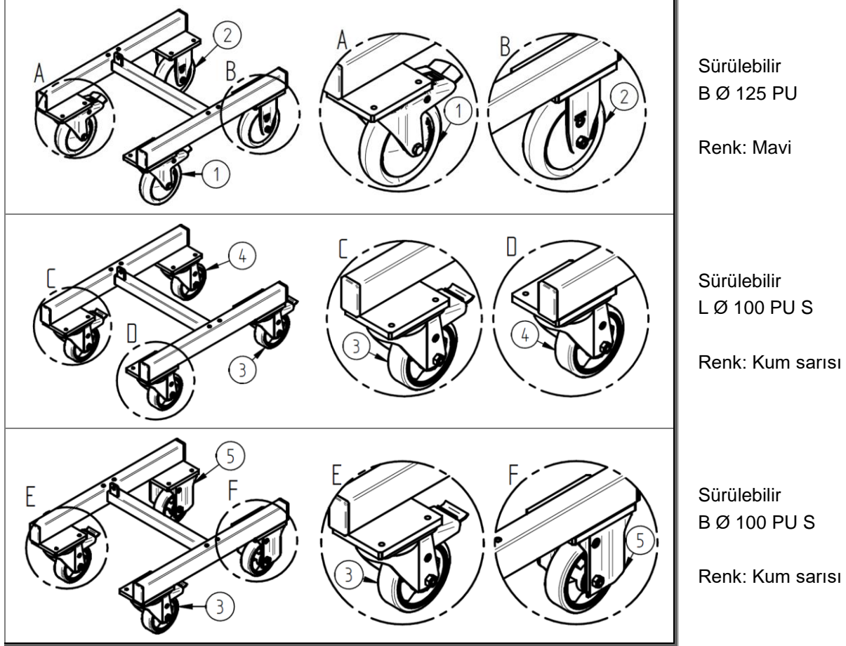
Şekil 105: Parça listesi: Alt şasi kurulum varyantları HE/HM Cıvata delikli tekerlekler ZZ.982.0068.01
