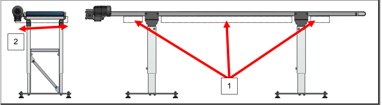
Şekil 22: Kaldırma düzenekleri (örn forklift) için bağlantı alanları
