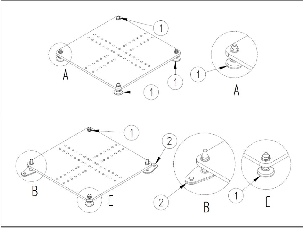
Şekil 111: Parça listesi: Alt şasi kurulum varyantları BE- ZZ.982.0079 / BM - ZZ.982.0121
