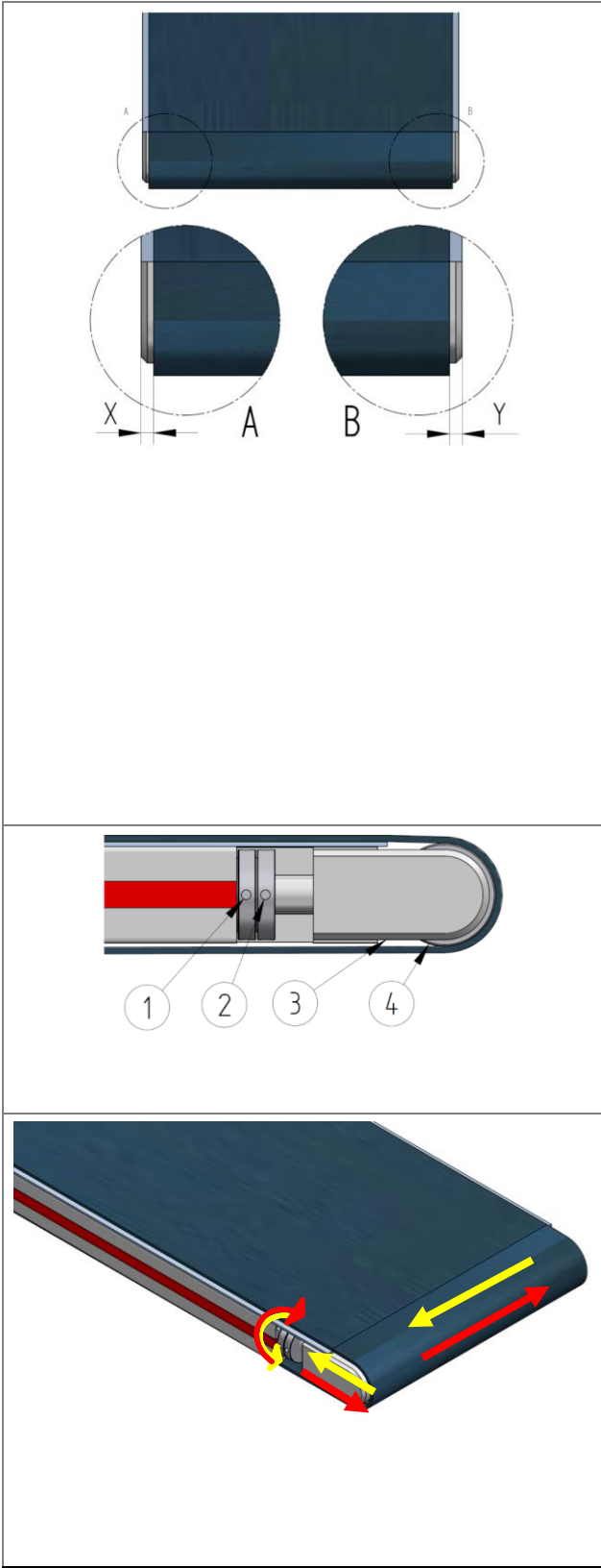
Şekil 61: Yön değiştirme bölgesindeki bant (kayış) senkronizasyonunun ayarlanması
