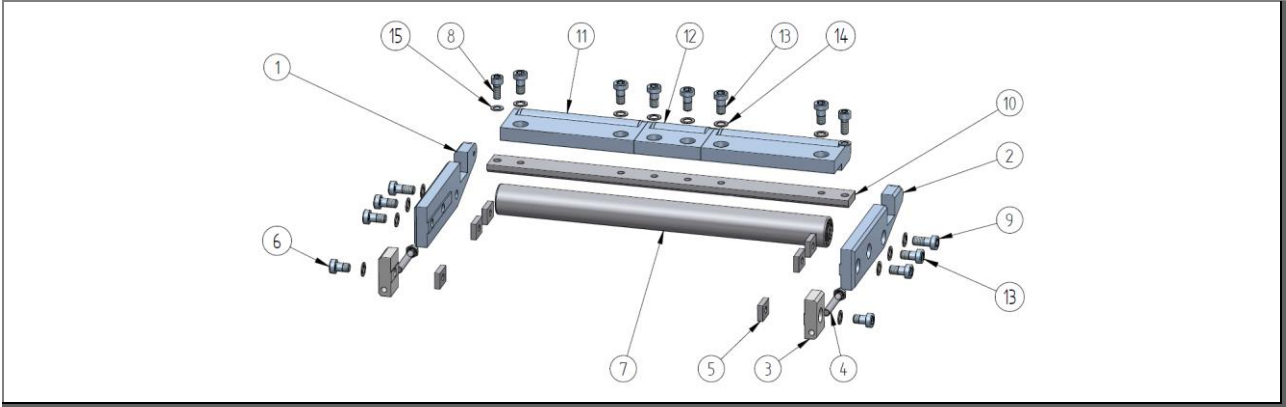
Şekil 76: Parça listesi: Döner bıçak ağızı Ø16 – U.910.0030
