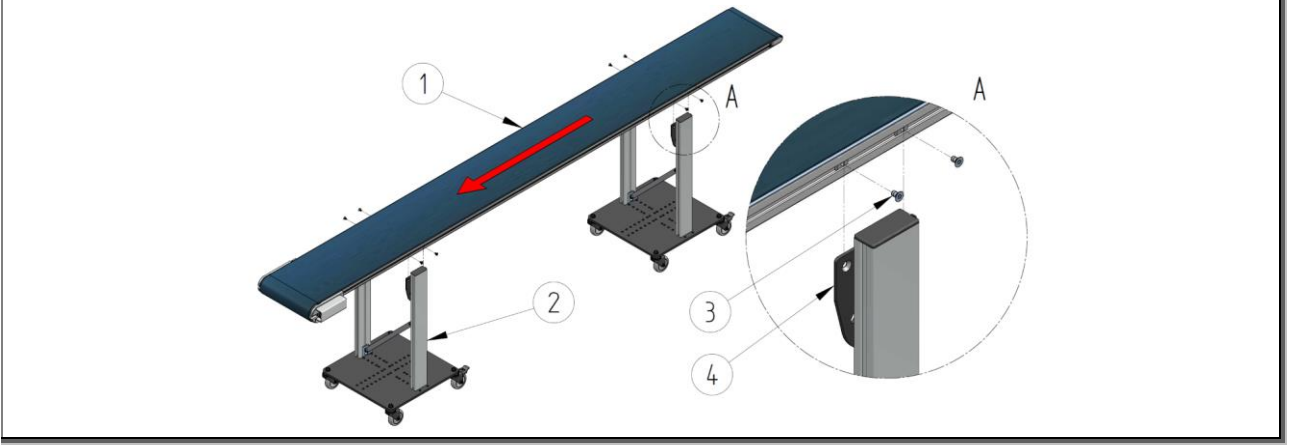
Şekil 48: BE 020 – BM 120 alt şasili konveyörün montajı (örnek)
