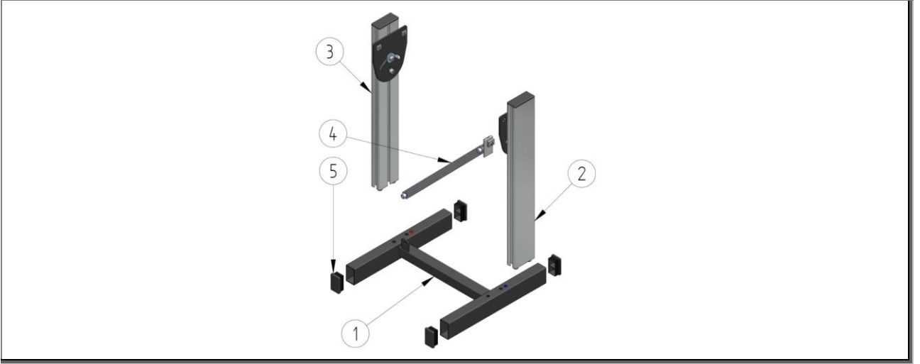
Şekil 101: Parça listesi: Alt şasi HE 060 - ZZ.982.0080 / HM 590 - ZZ.982.0081
