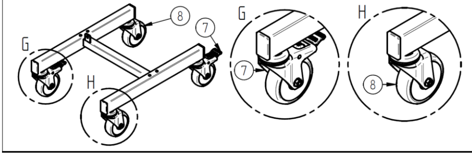
Şekil 104: Parça listesi: Alt şasi kurulum varyantları HE/HM Cıvata delikli tekerlekler ZZ.982.0068.01
