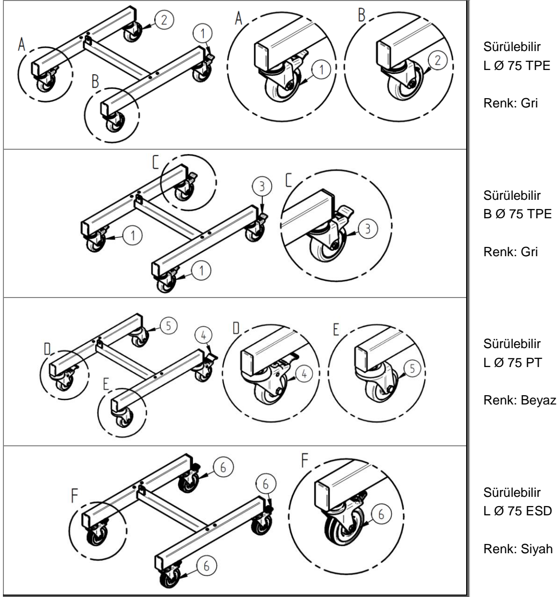
Şekil 103: Parça listesi: Alt şasi kurulum varyantları HE/HM Cıvata delikli tekerlekler ZZ.982.0068.01
