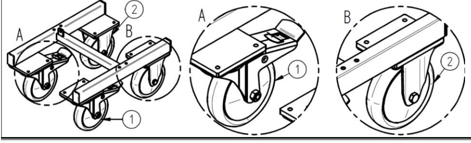
Şekil 106: Parça listesi: Alt şasi kurulum varyantları HE/HM Cıvata delikli tekerlekler ZZ.982.0068.01
