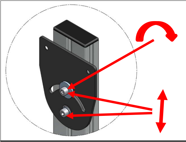
Şekil 31: AM 1030 alt şasisinin ayar olanakları
