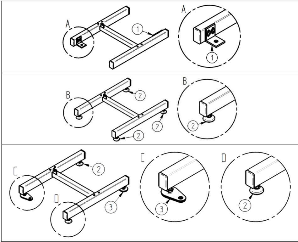
Şekil 102: Parça listesi: Alt şasi kurulum varyantları HE/HM ZZ.982.0068.01
