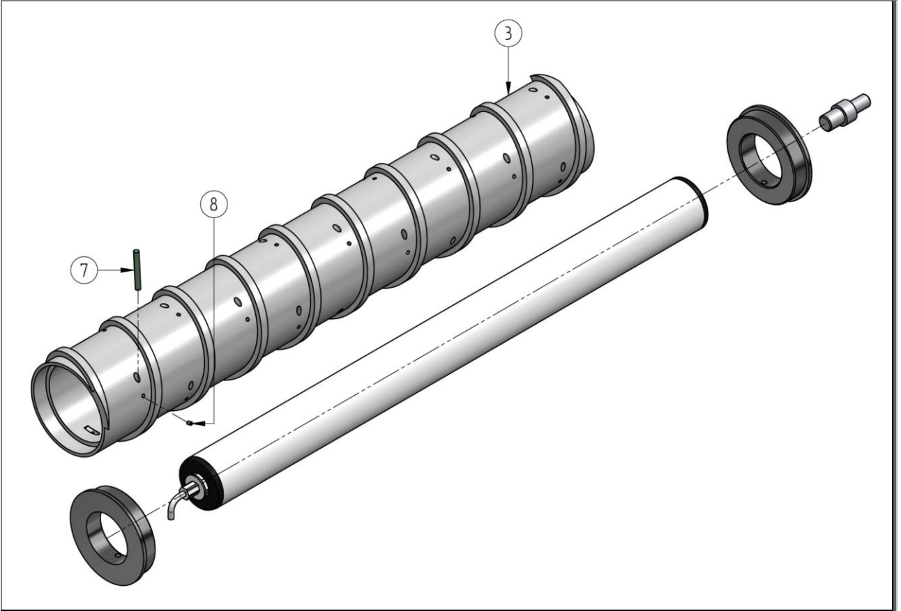
Res. 15: Paslanmaz çelik helikon silindri, motor ile
