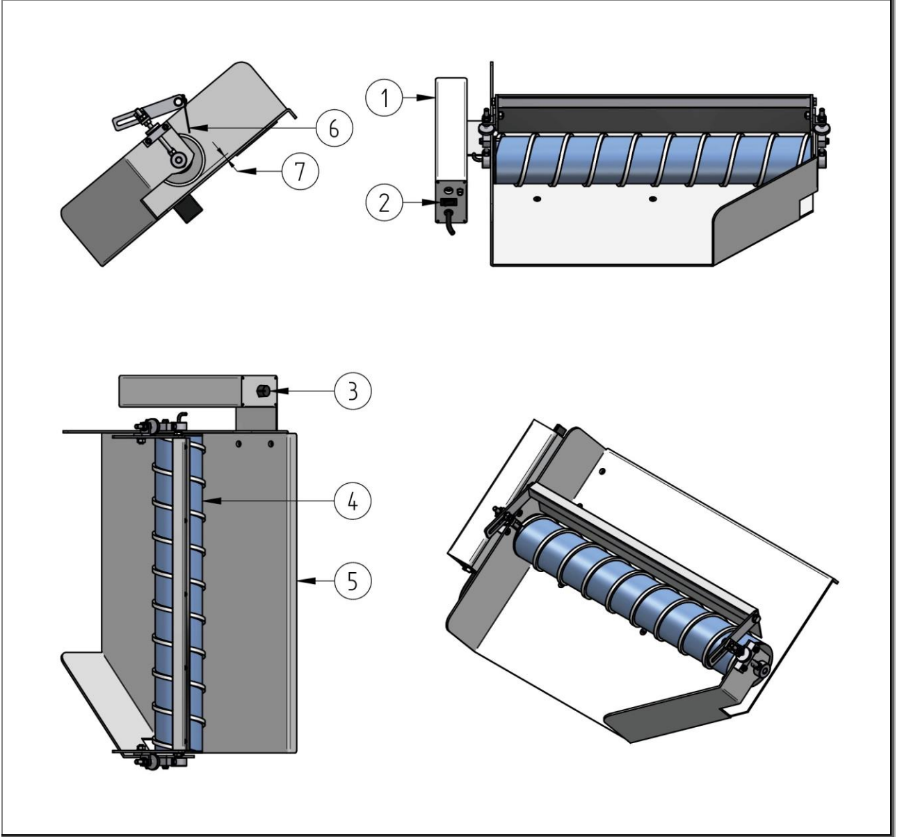
Res. 3: Helezon ayırıcı genel görünümü
