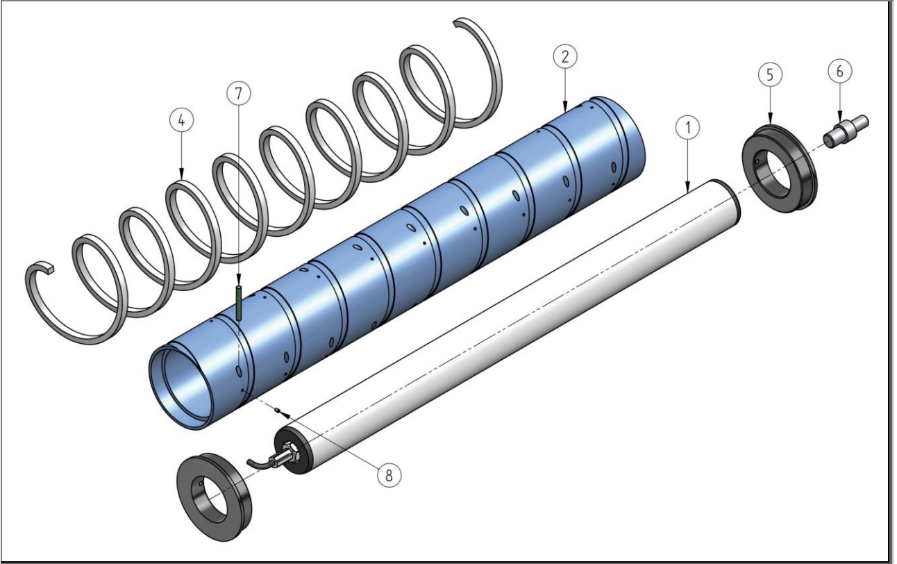
Res. 14: PVC helikon silindri (standart), motor ile
